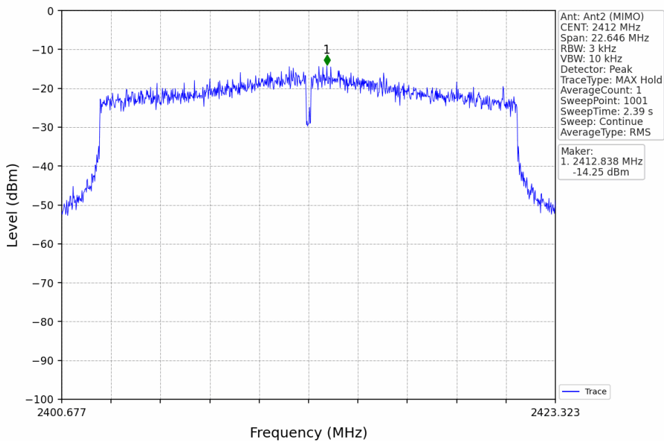
802.11ax(HEW20)_LCH_2412MHz_RU242_Left_Ant2 (MIMO)_NTNV
