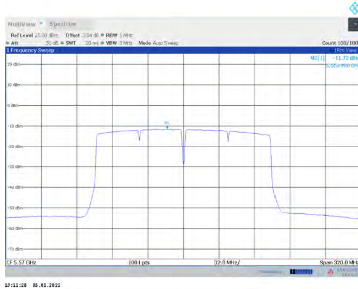
11AC160MIMO_Ant17_5570
