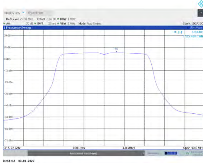
11AC20MIMO_Ant17_5220
