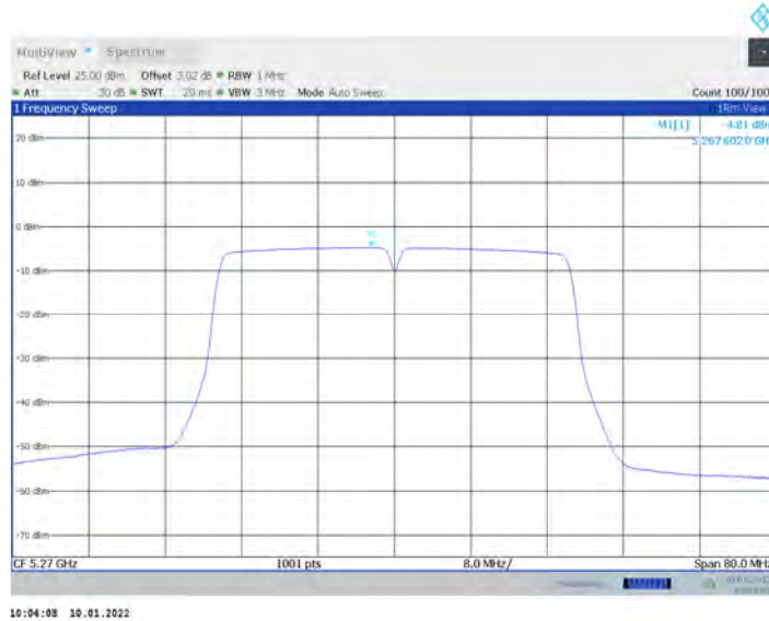
11N40MIMO_Ant17_5270
