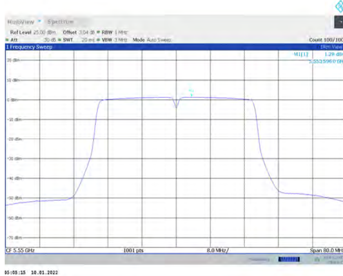
11AC40MIMO_Ant17_5550
