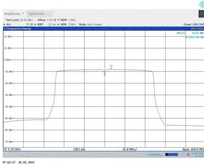
11AC80MIMO_Ant17_5290
