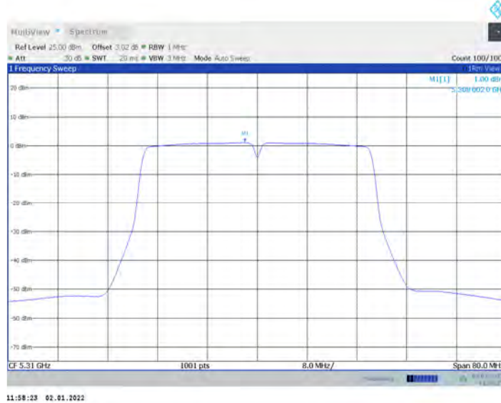
11N40MIMO_Ant17_5310
