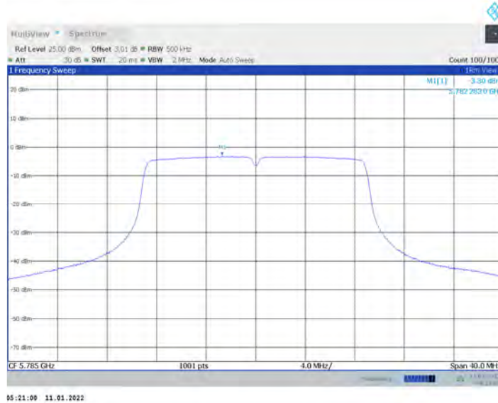
11AC20MIMO_Ant17_5785
