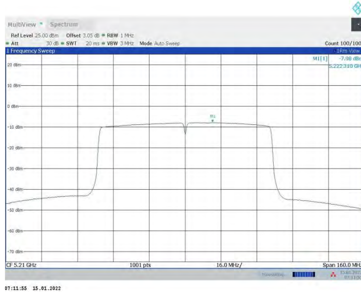
11AC80MIMO_Ant17_5210
