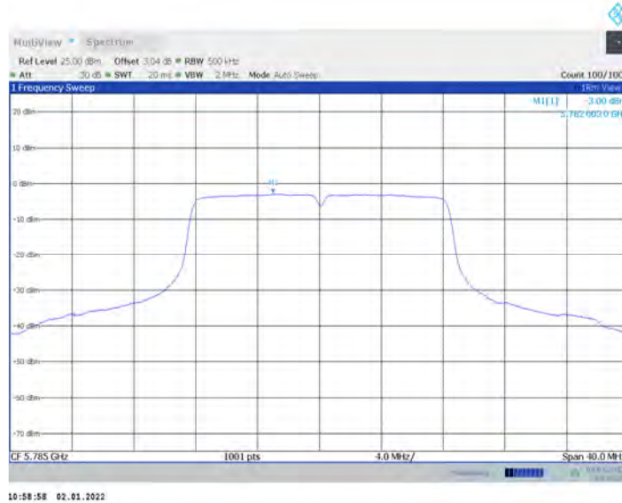
11A-CDD_Ant17_5785
