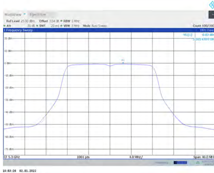
11A-CDD_Ant17_5300
