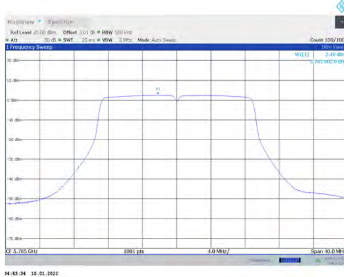
11AC20MIMO_Ant17_5785
