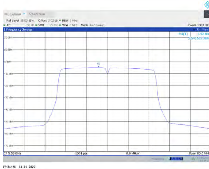
11AC40MIMO_Ant17_5550
