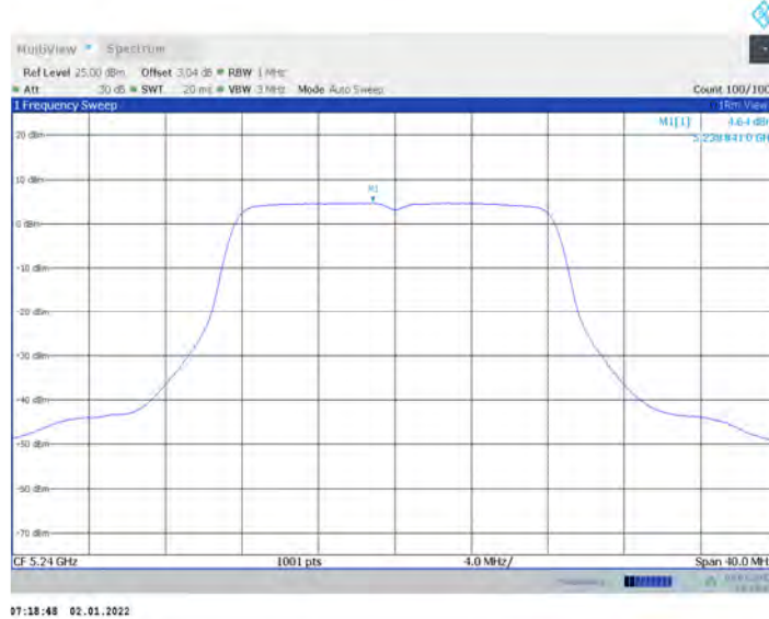
11A-CDD_Ant17_5240
