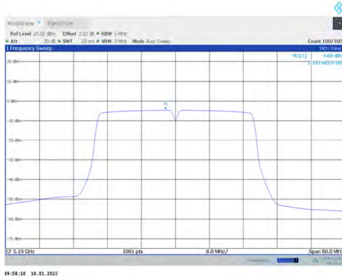
11N40MIMO_Ant17_5190
