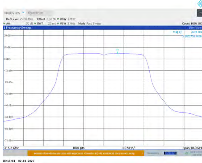
11A-CDD_Ant17_5300
