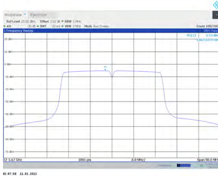
11N40MIMO_Ant17_5670
