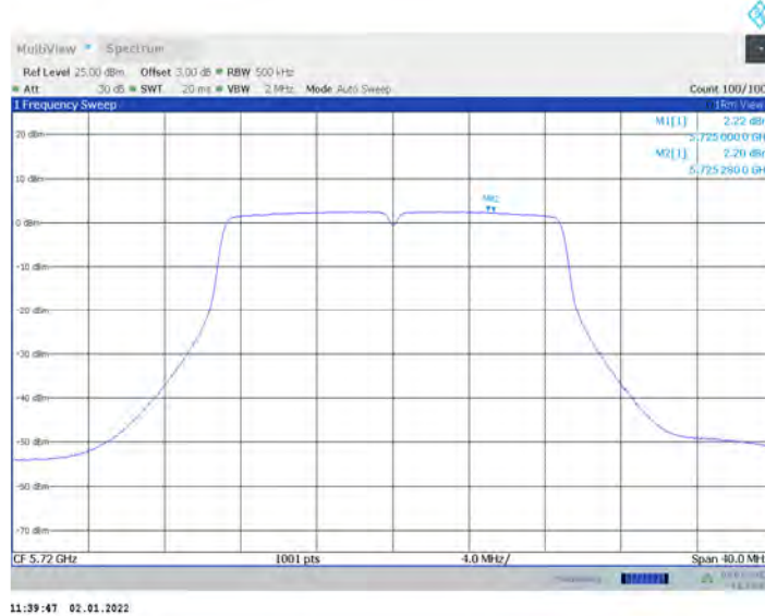
11N20MIMO_Ant17_5720_UNII-3
