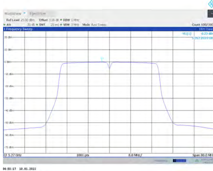
11AC40MIMO_Ant17_5270
