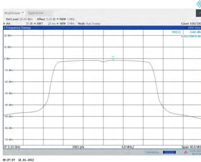
11AX20MIMO_Ant17_5220
