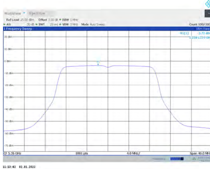
11N20MIMO_Ant17_5260
