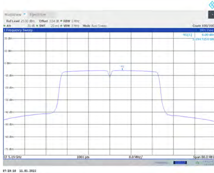
11AC40MIMO_Ant17_5190
