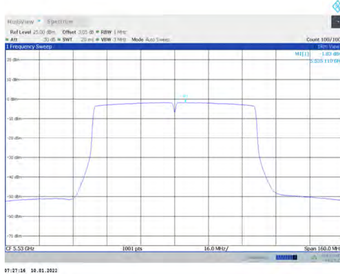
11AC80MIMO_Ant17_5530
