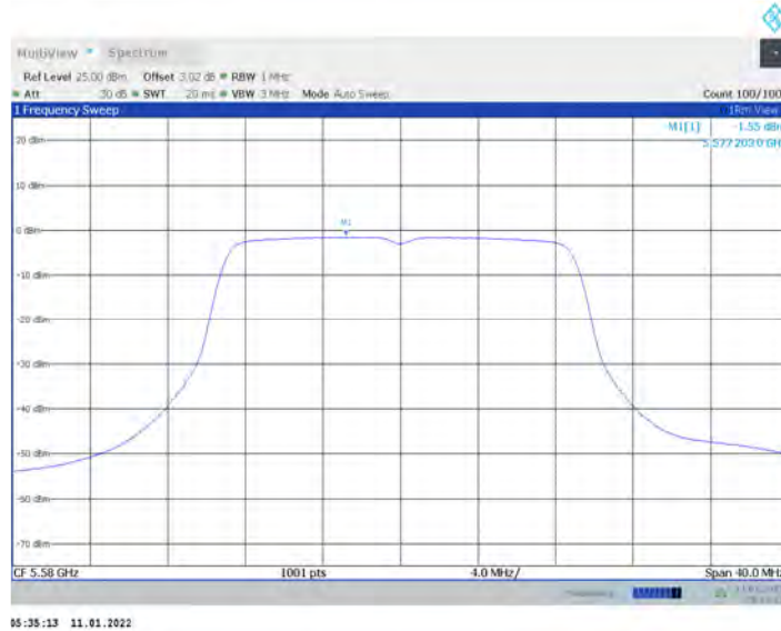
11AC20MIMO_Ant17_5580
