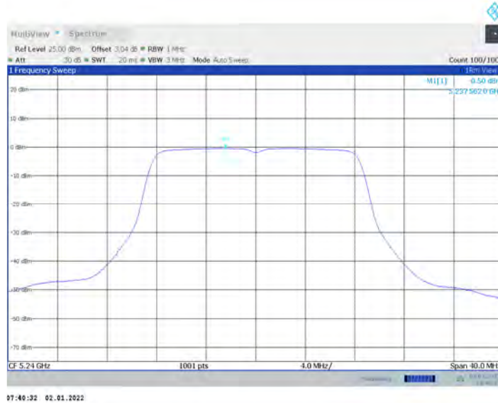
11A-CDD_Ant17_5240
