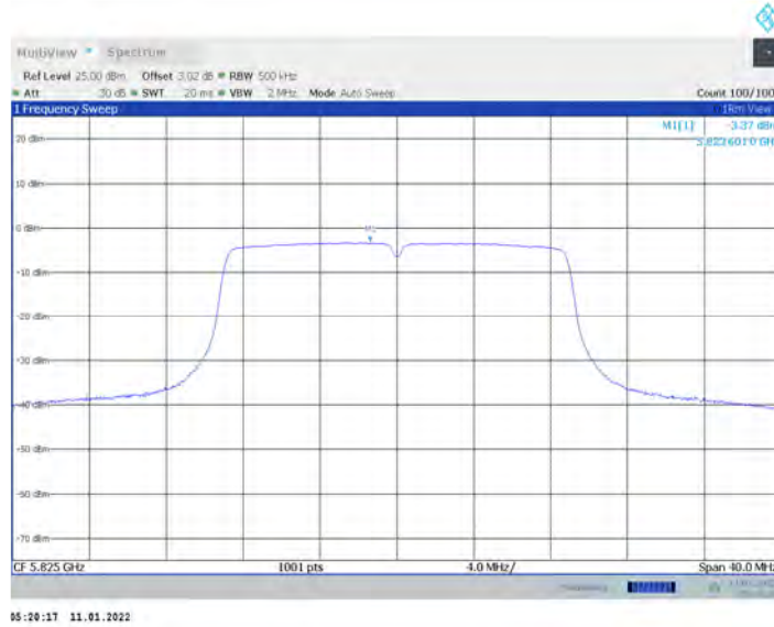
11AC20MIMO_Ant17_5825
