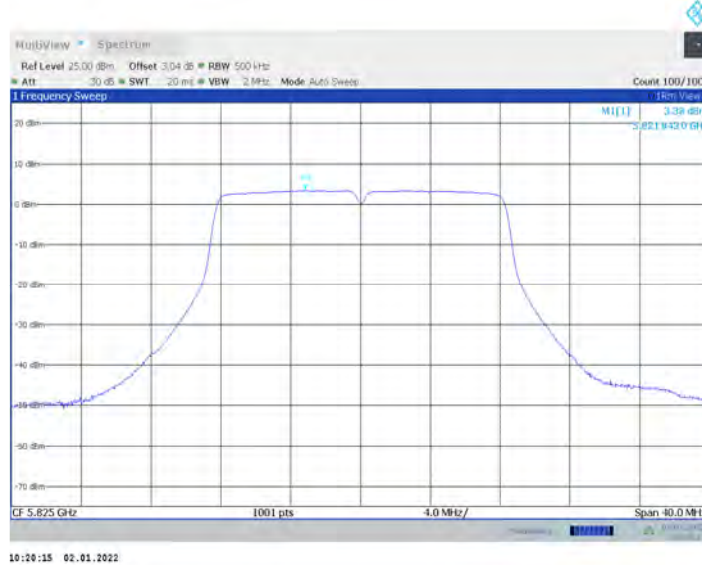
11A-CDD_Ant17_5825
