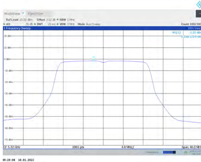
11N20MIMO_Ant17_5320
