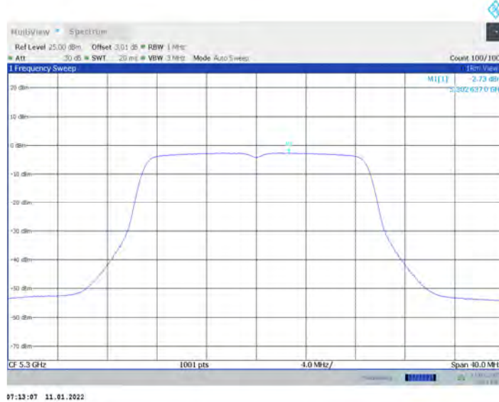
11AC20MIMO_Ant17_5300
