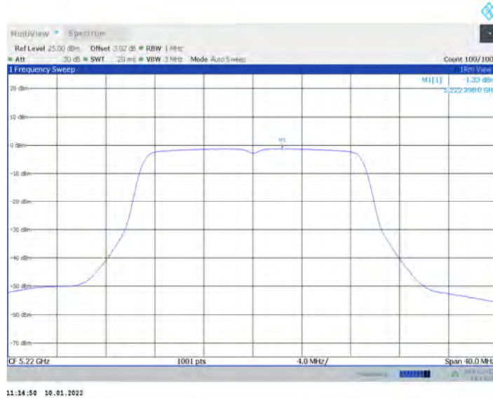
11AC20MIMO_Ant17_5220
