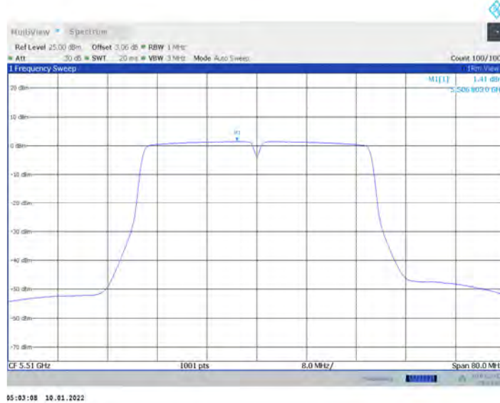
11AC40MIMO_Ant17_5510
