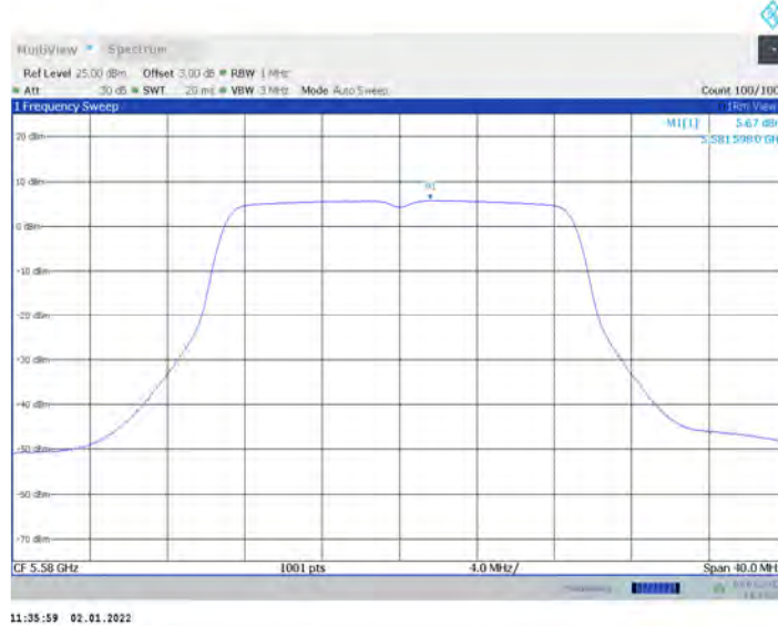
11N20MIMO_Ant17_5580
