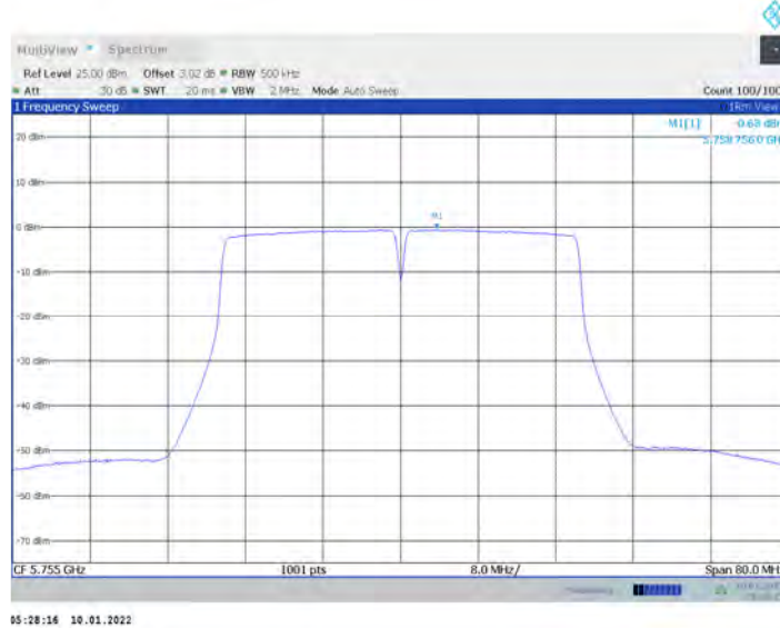
11AC40MIMO_Ant17_5755
