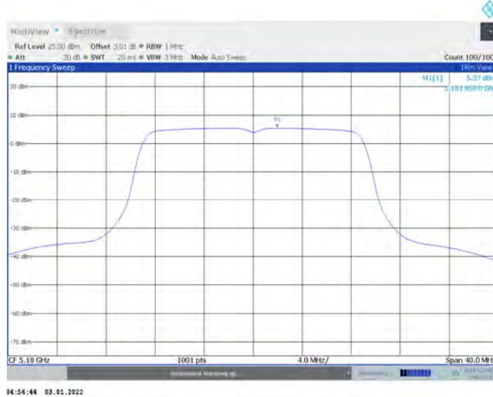
11AC20MIMO_Ant17_5180
