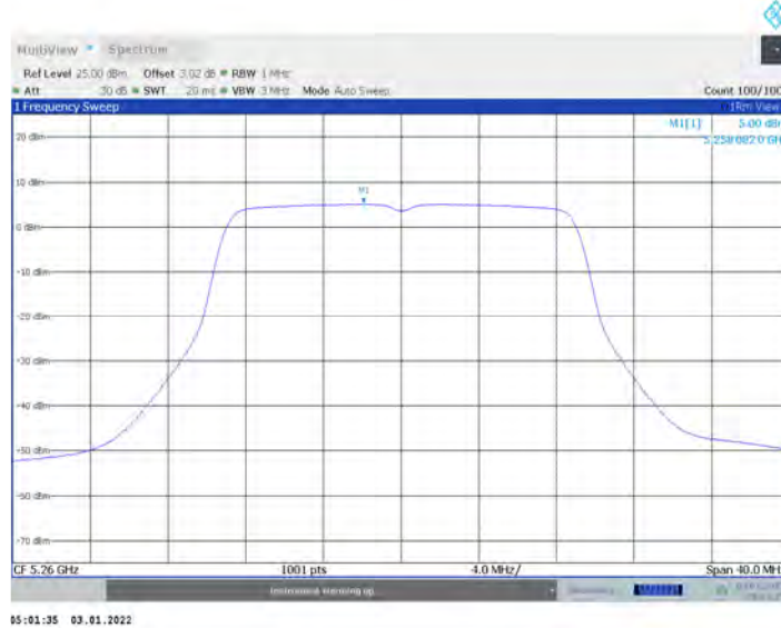
11AC20MIMO_Ant17_5260
