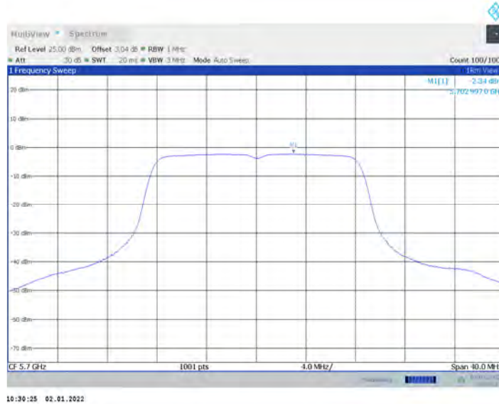
11A-CDD_Ant17_5700
