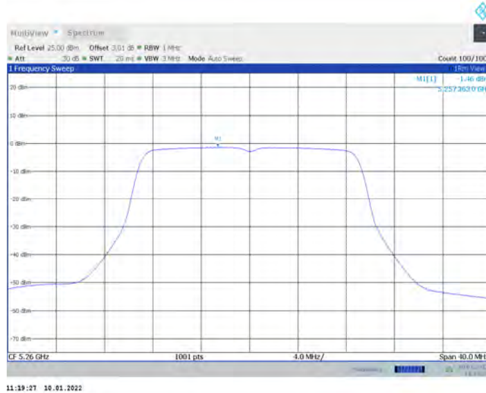
11AC20MIMO_Ant17_5260
