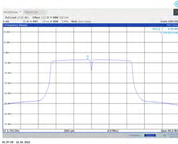
11N40MIMO_Ant17_5795
