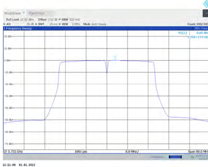
11N40MIMO_Ant17_5755
