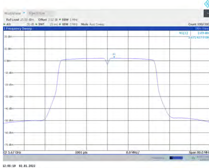
11N40MIMO_Ant17_5670
