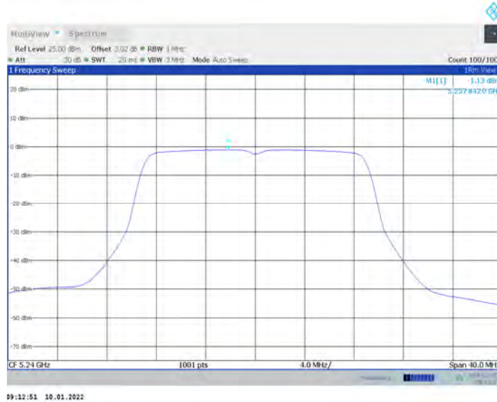
11N20MIMO_Ant17_5240
