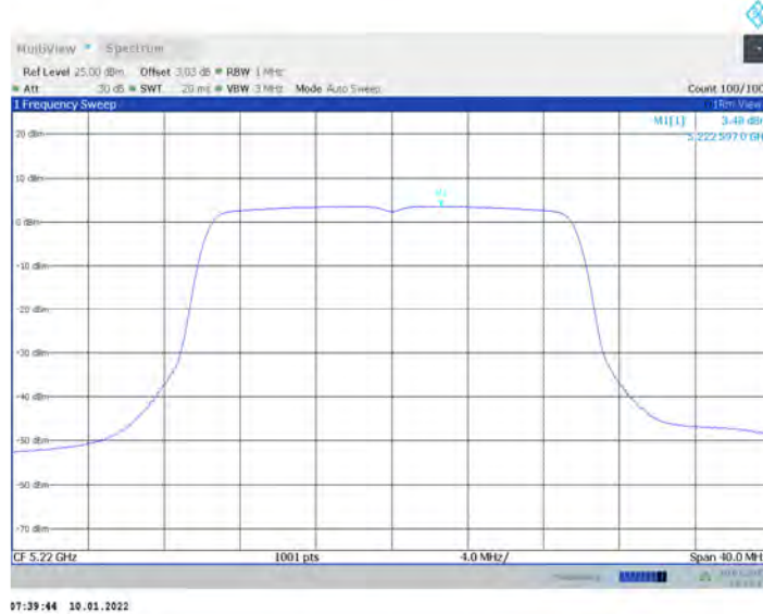
11AX20MIMO_Ant17_5220
