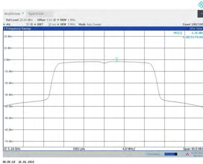
11AX20MIMO_Ant17_5180
