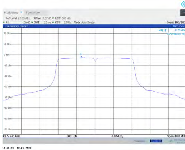
11A-CDD_Ant17_5745
