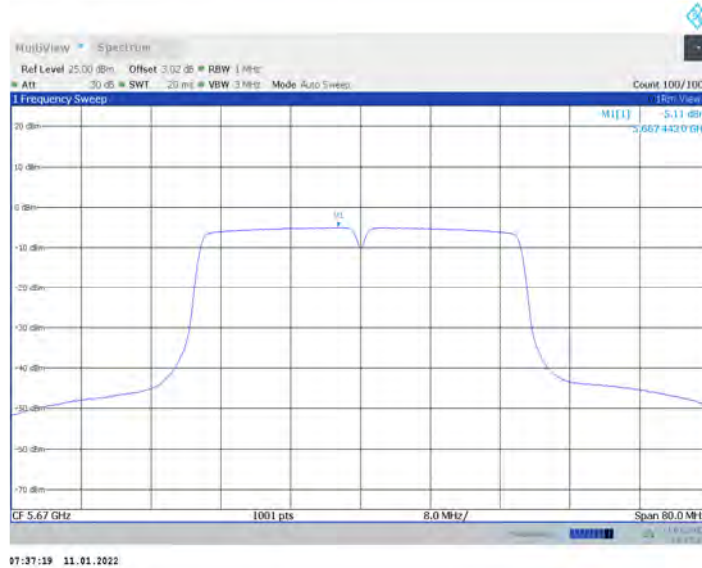
11AC40MIMO_Ant17_5670
