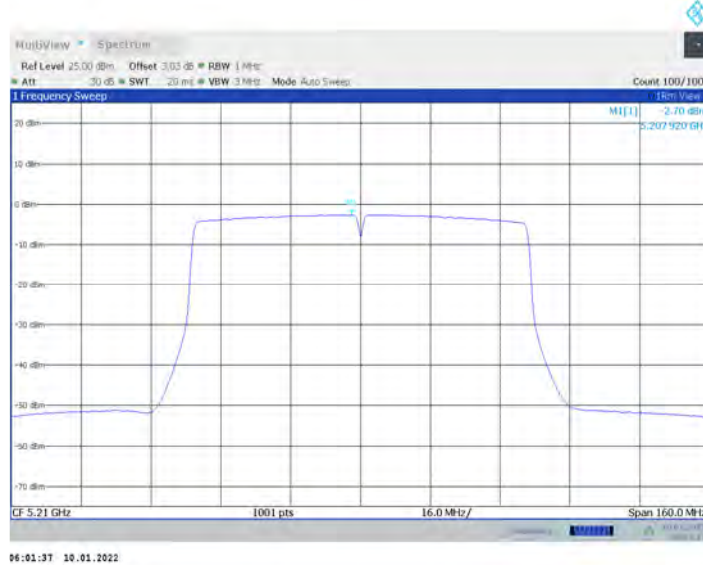
11AC80MIMO_Ant17_5210
