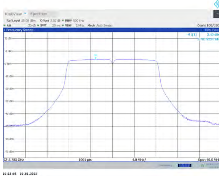
11A-CDD_Ant17_5785
