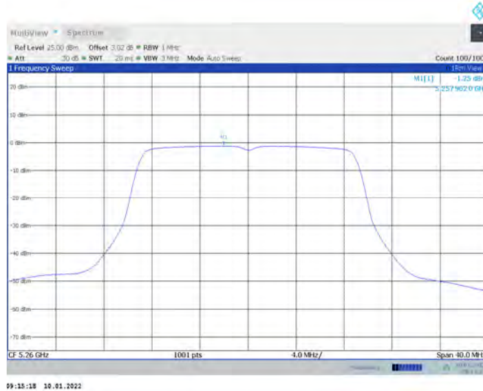
11N20MIMO_Ant17_5260
