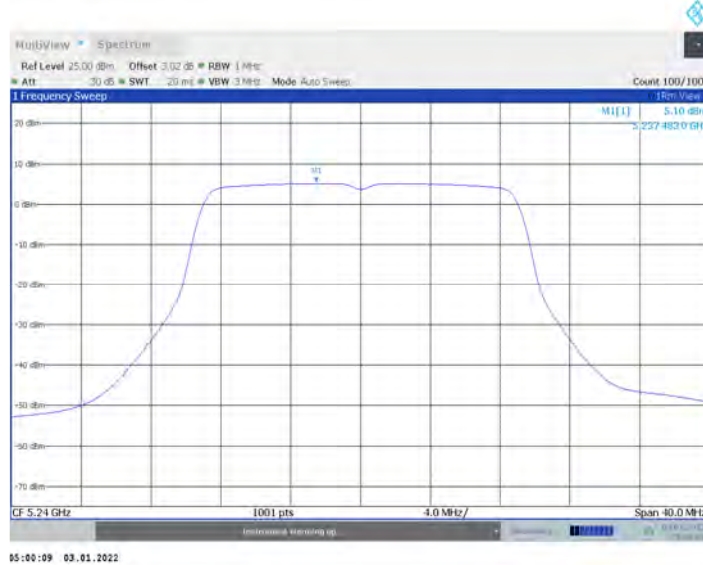
11AC20MIMO_Ant17_5240
