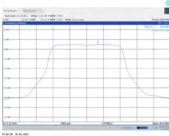
11A-CDD_Ant17_5220
