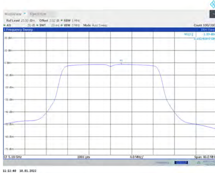
11AC20MIMO_Ant17_5180
