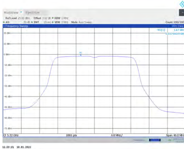
11AC20MIMO_Ant17_5320
