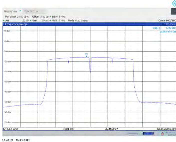
11AC160MIMO_Ant17_5570
