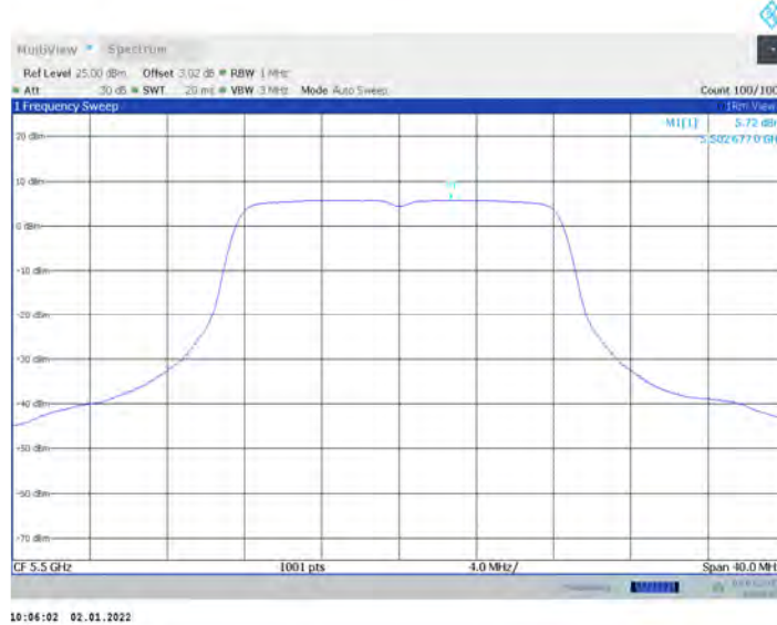
11A-CDD_Ant17_5500
