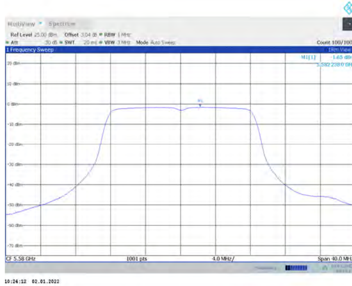
11A-CDD_Ant17_5580
