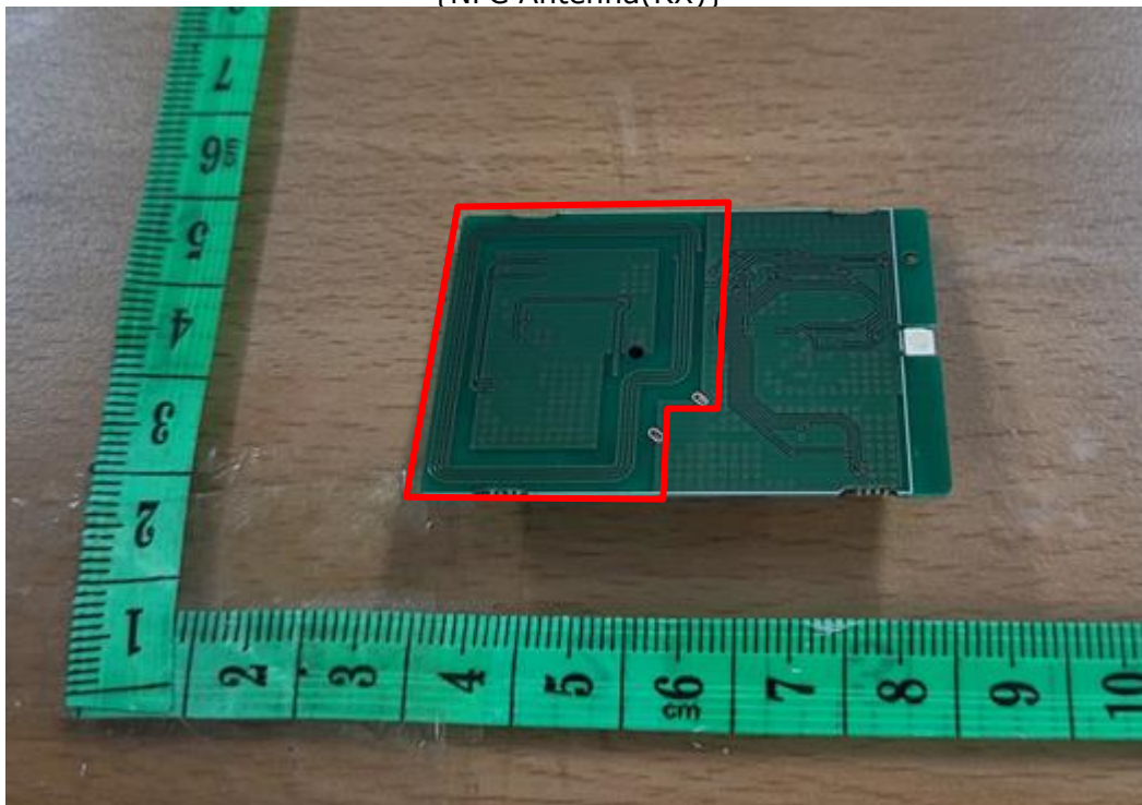
{NFC Antenna(RX)}
