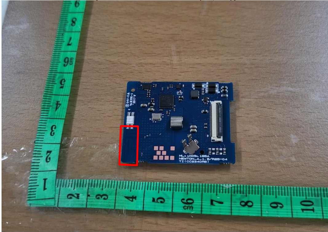
{NFC Antenna(RX)}
