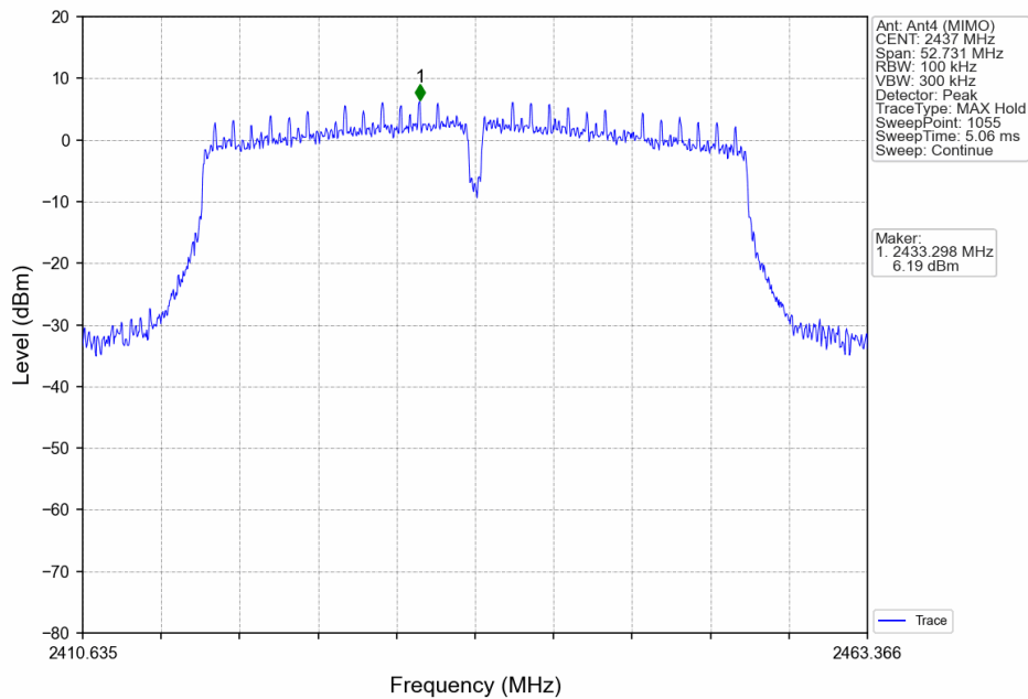
802.11n(HT40)_MCH_2437MHz_Ant4 (MIMO)_NTNV
