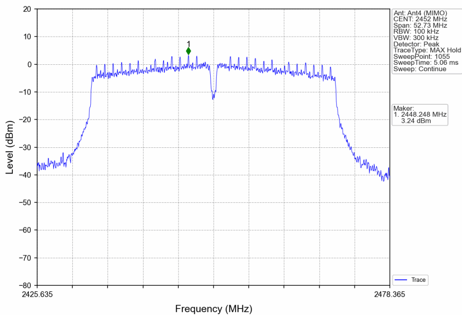
802.11n(HT40)_HCH_2452MHz_Ant4 (MIMO)_NTNV
