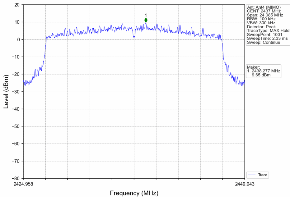
802.11ax(HEW20)_MCH_2437MHz_RU242_Left_Ant4 (MIMO)_NTNV
