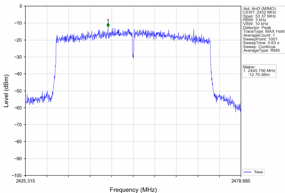
802.11ax(HEW40)_HCH_2452MHz_RU484_Left_Ant3 (MIMO)_NTNV
