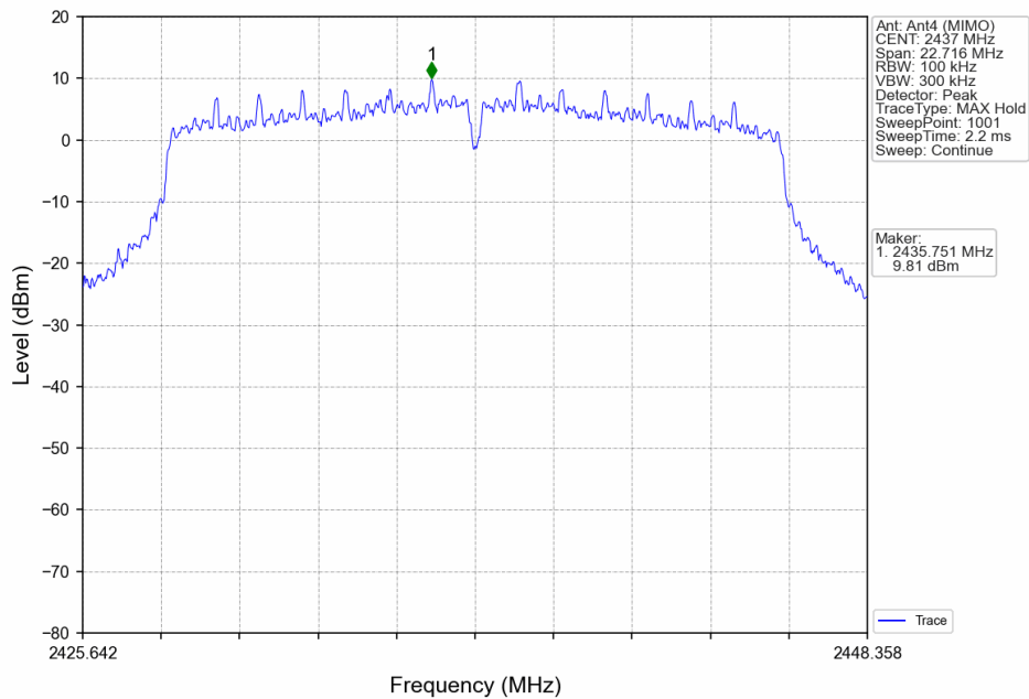
802.11n(HT20)_MCH_2437MHz_Ant4 (MIMO)_NTNV
