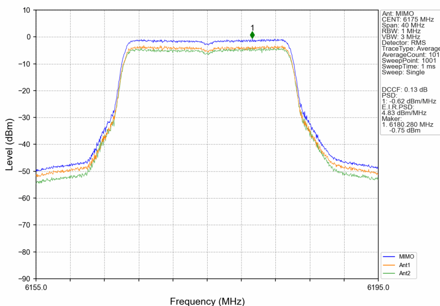
802.11be(EHT20)_MCH_6175MHz_RU242_Left_MIMO_NTNV
