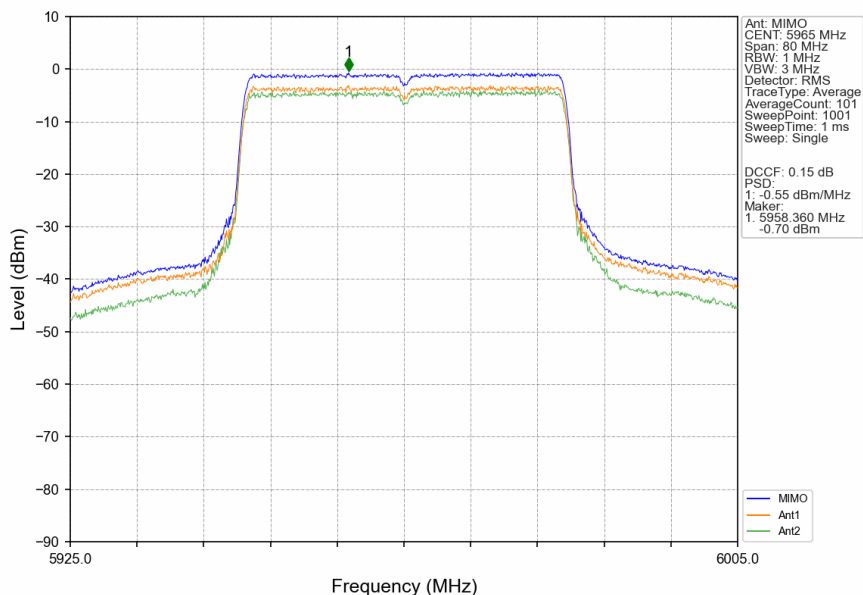
802.11be(EHT40)_LCH_5965MHz_RU484_Left_MIMO_NTNV
