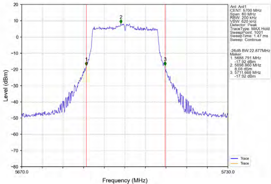
802.11be(EHT20)_HCH_5700MHz_SU_ / _Ant1_NTNV
