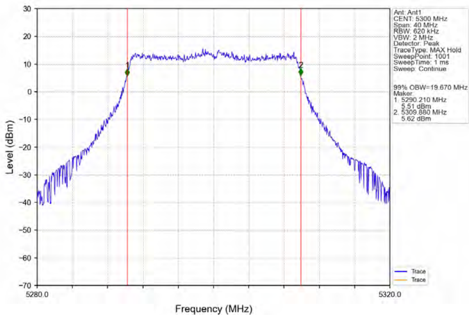
802.11be(EHT20)_MCH_5300MHz_SU_ / _Ant1_NTNV
