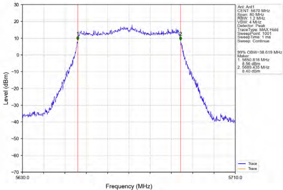
802.11be(EHT40)_HCH_5670MHz_SU_ / _Ant1_NTNV
