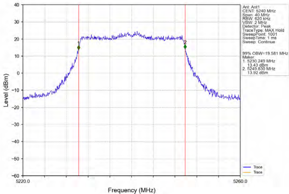
802.11be(EHT20)_HCH_5240MHz_SU_ / _Ant1_NTNV
