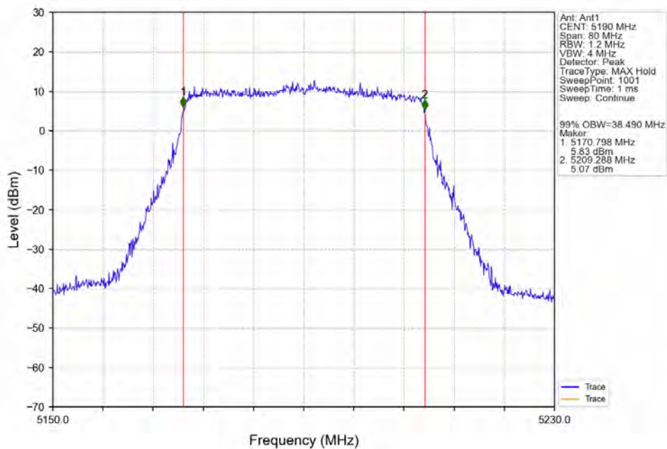
802.11be(EHT40)_LCH_5190MHz_SU_ / _Ant1_NTNV
