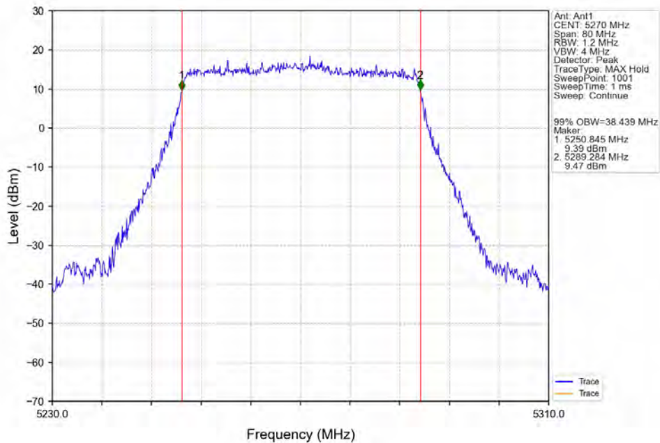
802.11be(EHT40)_LCH_5270MHz_SU_ / _Ant1_NTNV
