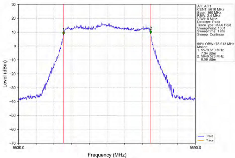
802.11be(EHT80)_HCH_5610MHz_SU_ / _Ant1_NTNV
