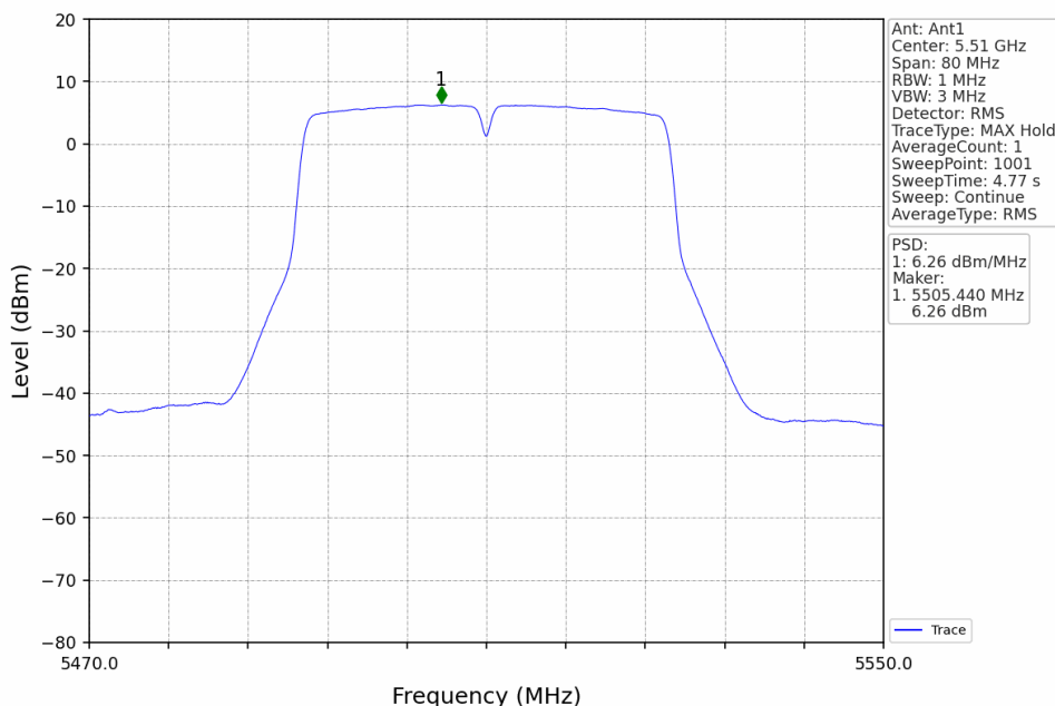
802.11n(HT40)_LCH_5510MHz_Ant1_NTNV
