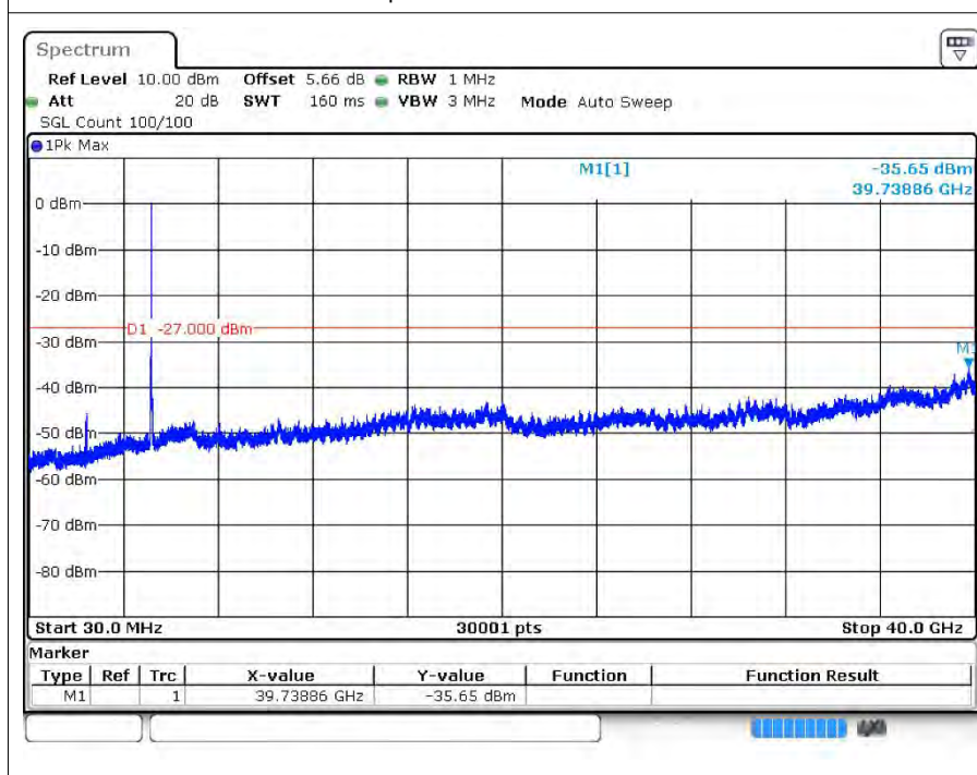
Tx. Spurious n20 5200MHz Ant1
