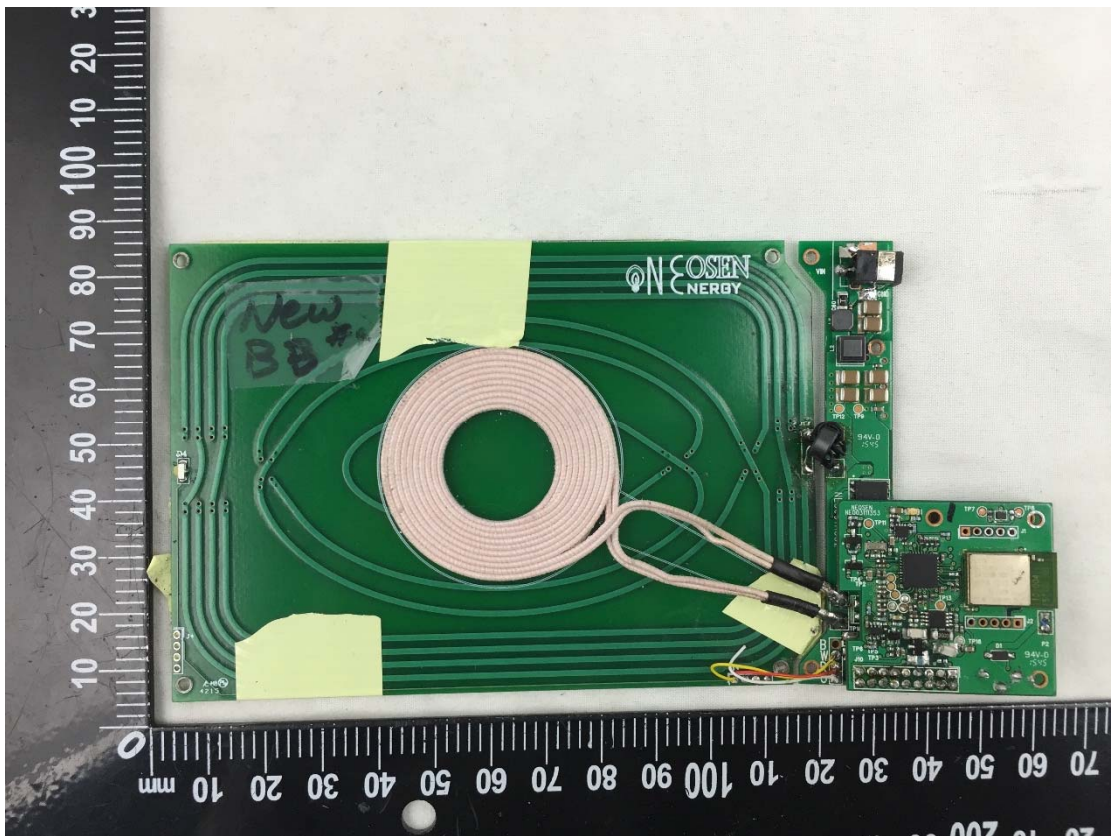
EUT Photo 4
