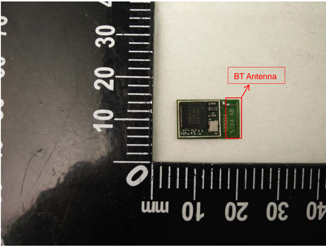
EUT Photo 11
