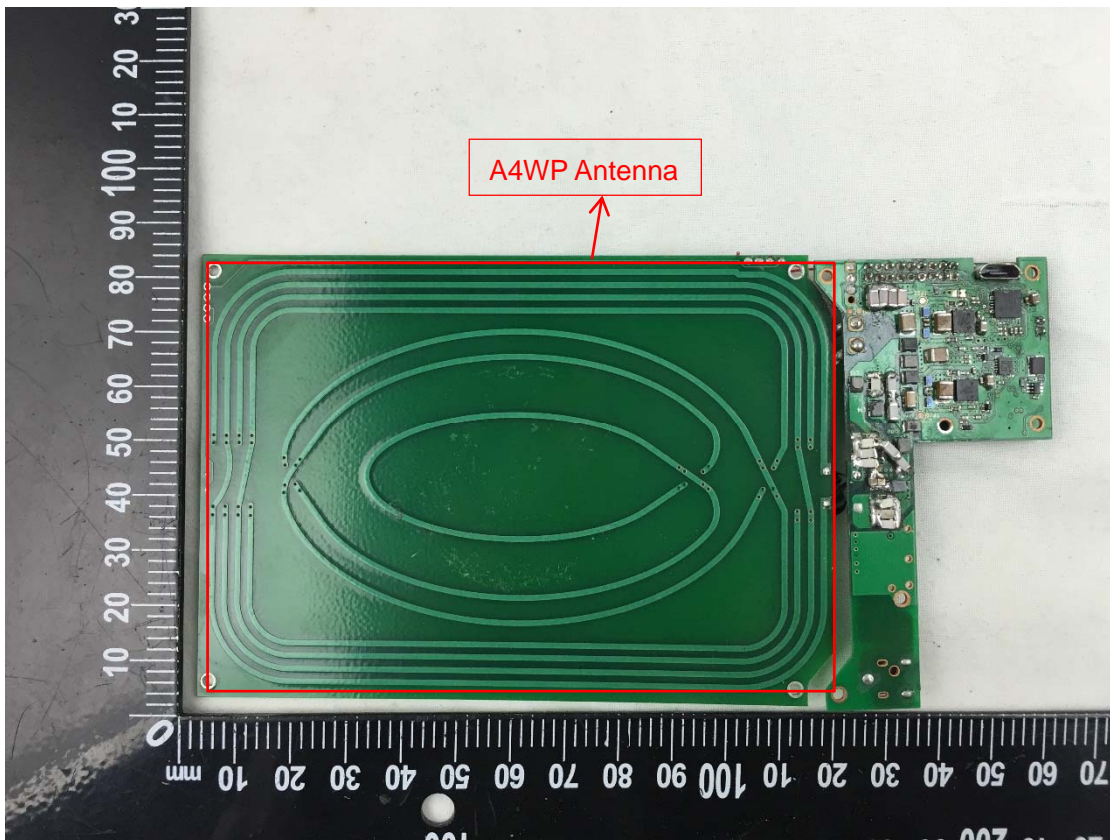
EUT Photo 6
