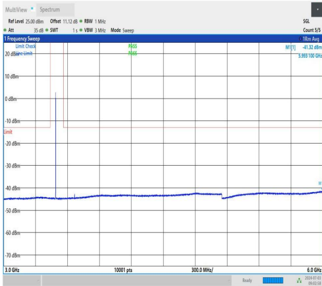
NTNV_DC_26A_n77A-3450-3550_PC2_30_5+40_M+L_TID2_NS_01_3000_6000_#1
