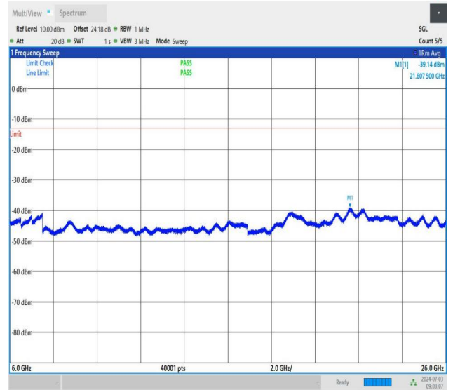
NTNV_DC_26A_n77A-3450-3550_PC2_30_5+40_M+L_TID2_NS_01_6000_26000_#1
