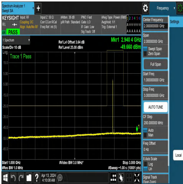
NTNV-N41-PC3-30-40-M-DFT-QPSK-Edge_1RB_Left-1000-3000- Ant1-PASS
