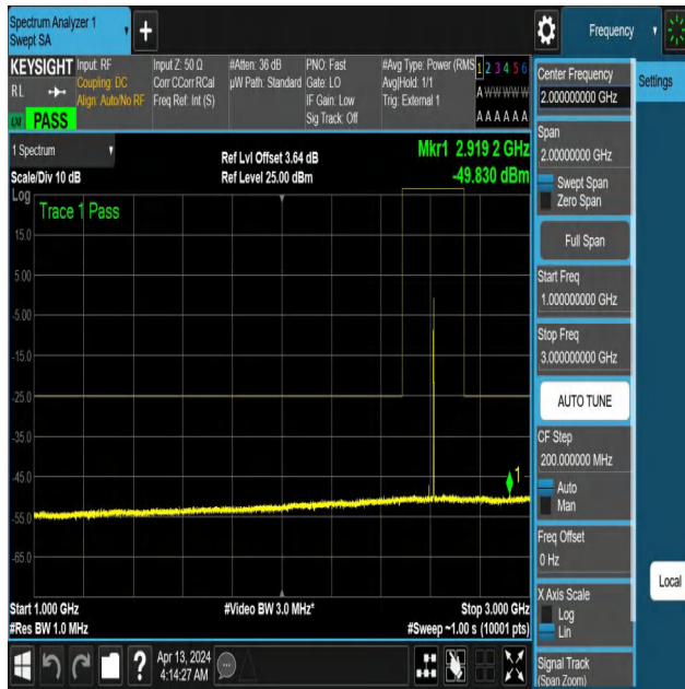
NTNV-N41-PC3-30-40-M-DFT-QPSK-Edge_1RB_Right-1000-300 0-Ant1-PASS
