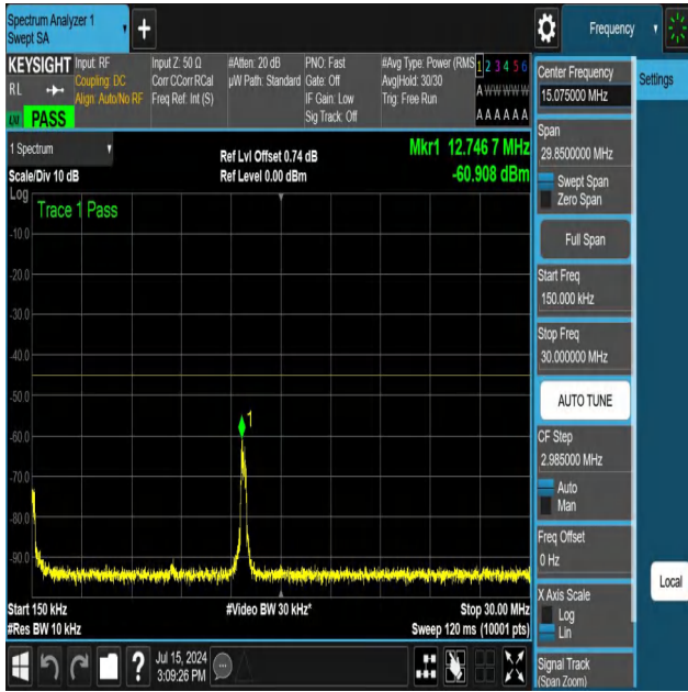
NTNV-N41-PC3-30-40-M-DFT-QPSK-Edge_1RB_Left-0.15-30-Ant 1-PASS
