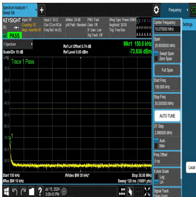
NTNV-N41-PC3-30-40-L-DFT-QPSK-Edge_1RB_Right-0.15-30-A nt1-PASS
