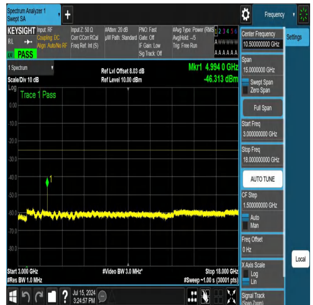
NTNV-N41-PC3-30-40-L-DFT-QPSK-Edge_1RB_Left-3000-1800 0-Ant1-PASS
