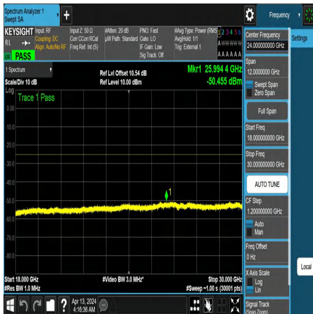
NTNV-N41-PC3-30-40-M-DFT-QPSK-Edge_1RB_Right-18000-30 000-Ant1-PASS
