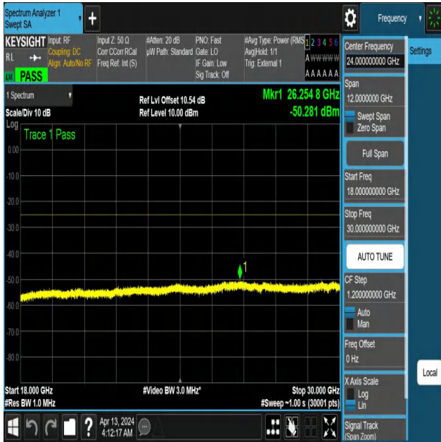
NTNV-N41-PC3-30-40-M-DFT-QPSK-Edge_1RB_Left-18000-300 00-Ant1-PASS
