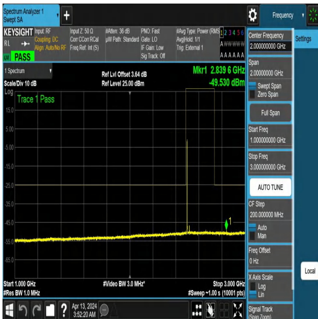
NTNV-N41-PC3-30-40-L-DFT-QPSK-Edge_1RB_Left-1000-3000- Ant1-PASS
