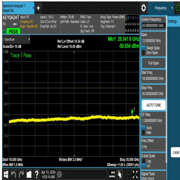
NTNV-N41-PC3-30-40-M-DFT-P12BPSK-Edge_1RB_Left-18000-3 0000-Ant1-PASS
