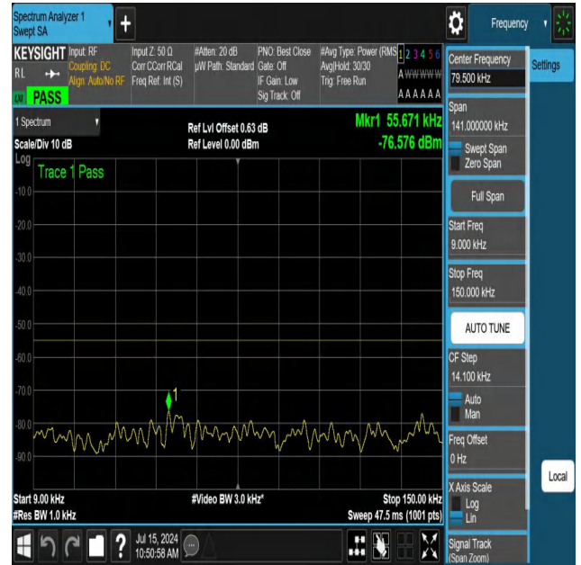
NTNV-N41-PC3-30-40-M-DFT-QPSK-Edge_1RB_Right-0.009-0. 15-Ant1-PASS
