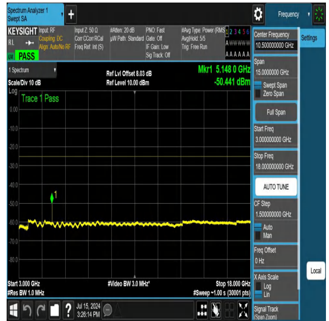
NTNV-N41-PC3-30-40-M-DFT-QPSK-Edge_1RB_Left-3000-1800 0-Ant1-PASS
