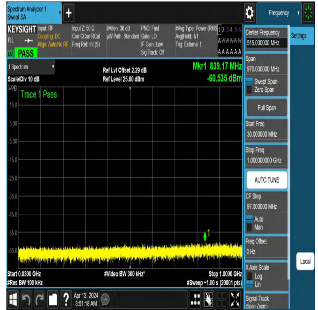
NTNV-N41-PC3-30-40-L-DFT-QPSK-Edge_1RB_Left-30-1000-A nt1-PASS
