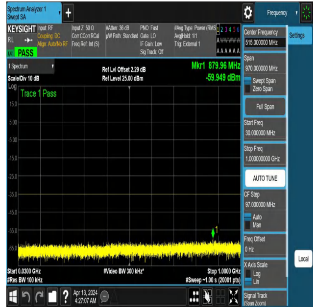
NTNV-N41-PC3-30-40-H-DFT-QPSK-Edge_1RB_Left-30-1000-A nt1-PASS
