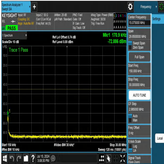
NTNV-N41-PC3-30-40-L-DFT-QPSK-Edge_1RB_Left-0.15-30-Ant 1-PASS
