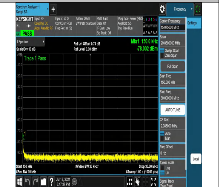
NTNV-N26-824-849-PC3-15-15-L-DFT-QPSK-Edge_1RB_Right-0. 15-30-Ant1-PASS
