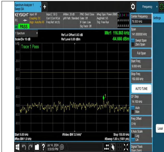
NTNV-N26-824-849-PC3-15-15-H-DFT-QPSK-Edge_1RB_Left-0.
