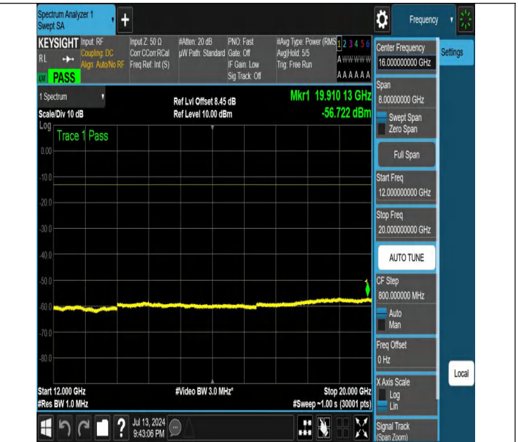
NTNV-N26-824-849-PC3-15-15-M-DFT-QPSK-Edge_1RB_Left-12 000-20000-Ant1-PASS
