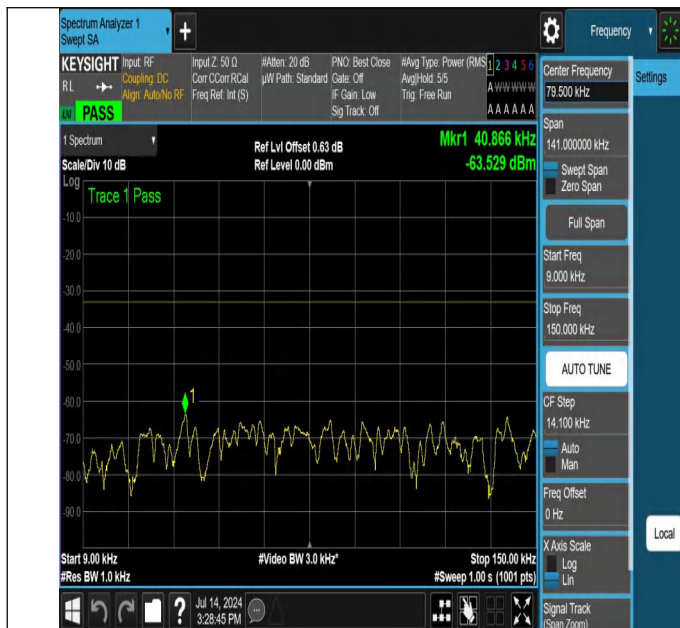
NTNV-N26-824-849-PC3-15-15-L-DFT-QPSK-Edge_1RB_Left-0. 009-0.15-Ant1-PASS
