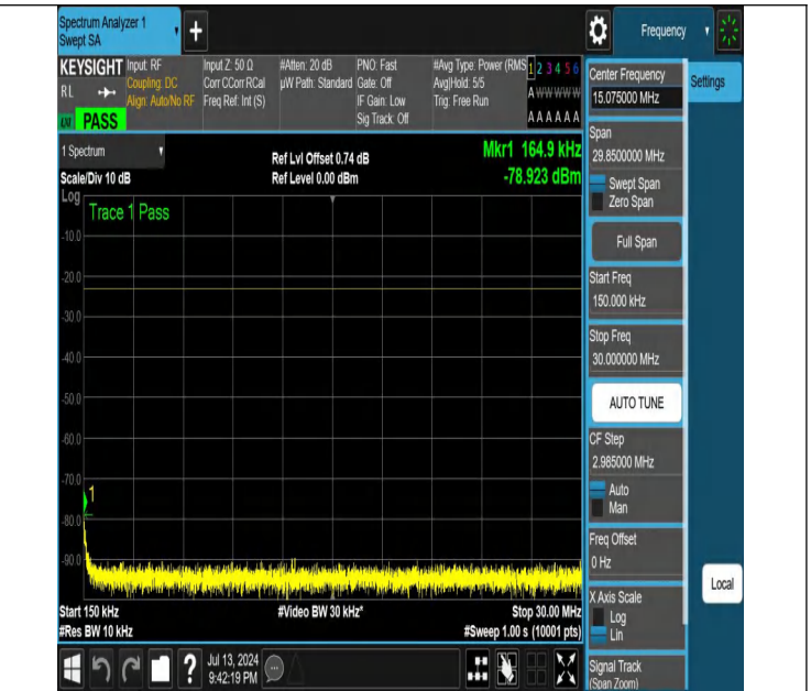
NTNV-N26-824-849-PC3-15-15-M-DFT-QPSK-Edge_1RB_Left-0. 15-30-Ant1-PASS
