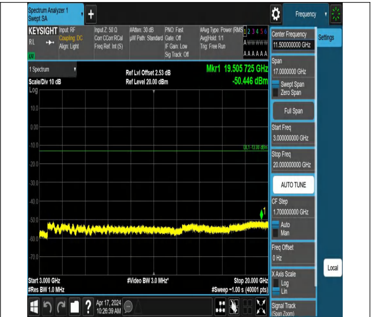
66-66-5MHz-20MHz-QPSK-QPSK-132027-132171-1RB#0-1RB# 99-3000~20000MHz-PASS
