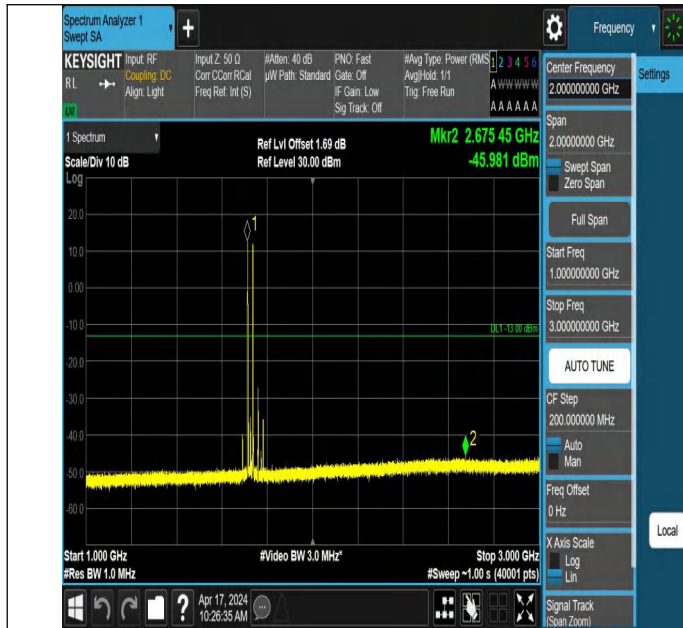
66-66-5MHz-20MHz-QPSK-QPSK-132027-132171-1RB#0-1RB#9 9-1000~3000MHz-PASS
