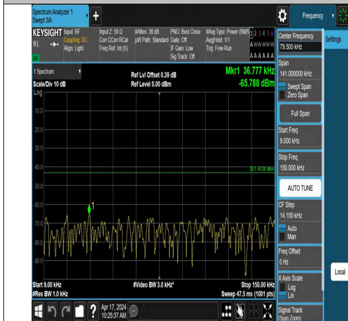
66-66-5MHz-20MHz-QPSK-QPSK-132027-132171-1RB#24-0RB# 0-0.009~0.15MHz-PASS
