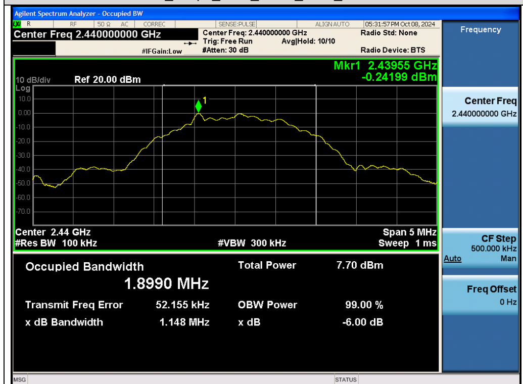
Test_Graph_2.4G_ANT1_2440_DTBSW
