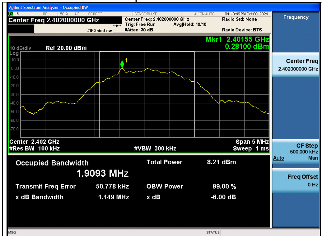
Test_Graph_2.4G_ANT1_2402_DTBSW
