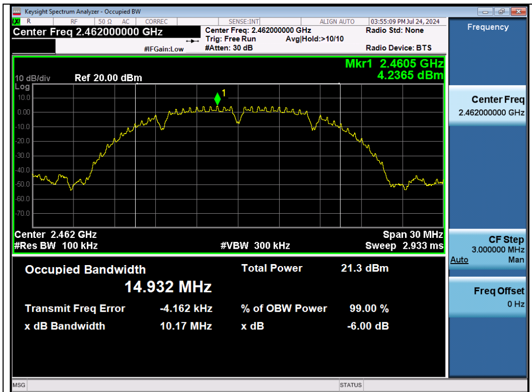
Test_Graph_802.11b_Chain B_2462_1Mbps_DTSSBW
