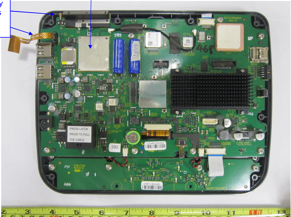
RF Module Circuit
