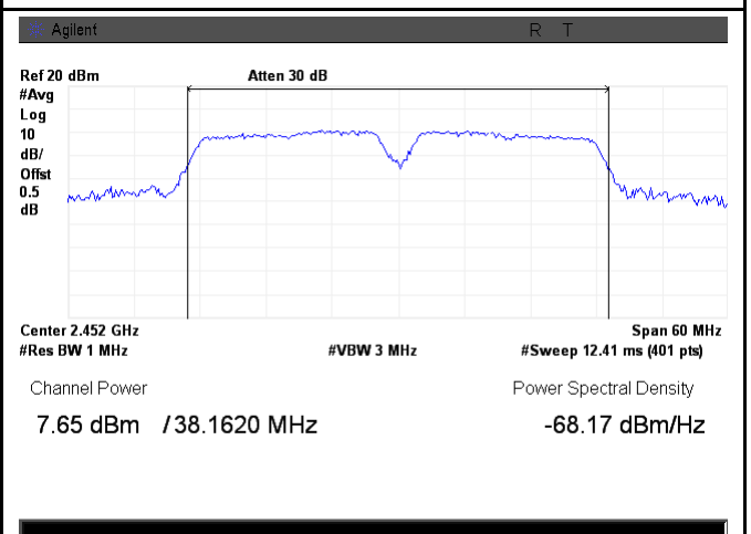
802.11n40 - AV Output power - High CH 2452
