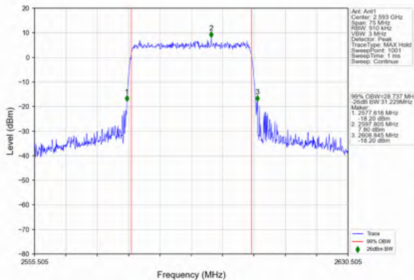
n41_15kHz_SISO_NTNV_30MHz_DFT-s-OFDM_256_QAM_2593.005MHz_Outer_Full
