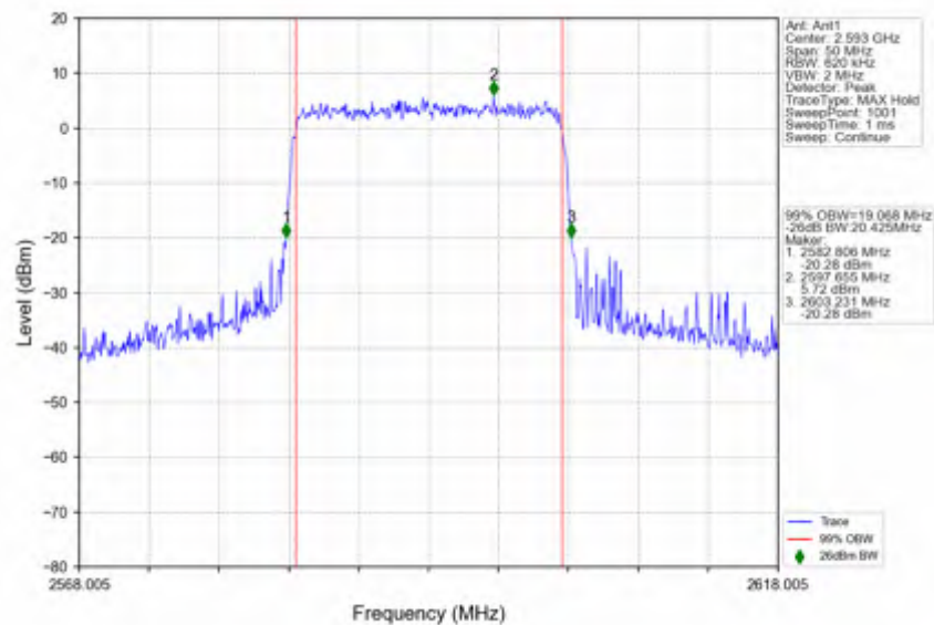
n41_15kHz_SISO_NTNV_20MHz_CP-OFDM_256_QAM_2593.005MHz_Outer_Full
