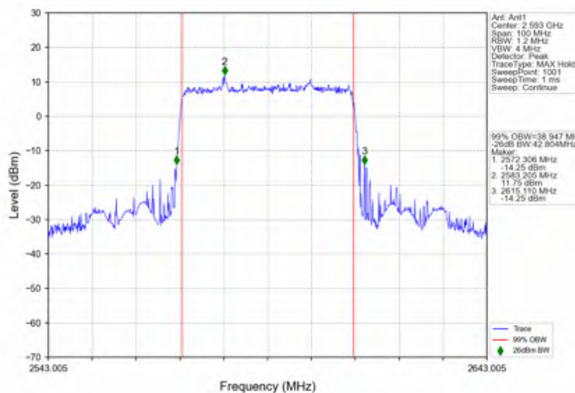
n41_15kHz_SISO_NTNV_40MHz_DFT-s-OFDM_PI/2_BPSK_2593.005MHz_Outer_Full
