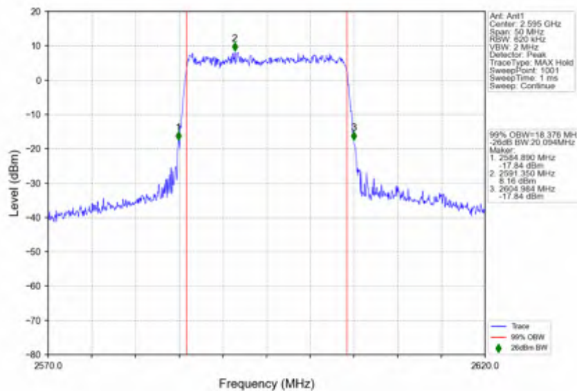
n38 30kHz SISO NTNV 20MHz CP-OFDM 256 QAM 2595MHz Outer Full
