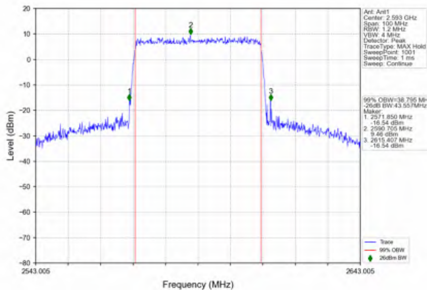
n41_15kHz_SISO_NTNV_40MHz_DFT-s-OFDM_16_QAM_2593.005MHz_Outer_Full
