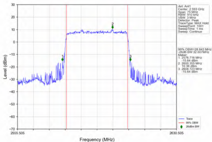
n41_15kHz_SISO_NTNV_30MHz_DFT-s-OFDM_PI/2_BPSK_2593.005MHz_Outer_Full
