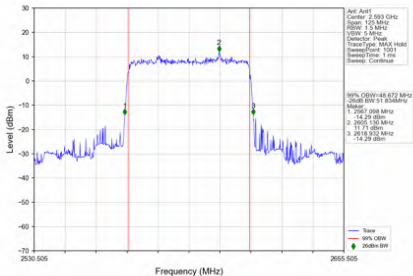
n41_15kHz_SISO_NTNV_50MHz_DFT-s-OFDM_PI/2_BPSK_2593.005MHz_Outer_Full
