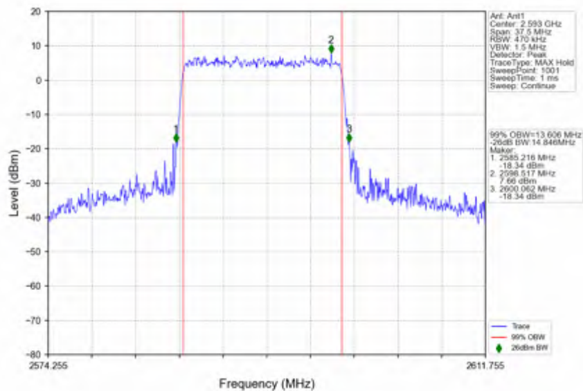
n41_15kHz_SISO_NTNV_15MHz_DFT-s-OFDM_256_QAM_2593.005MHz_Outer_Full
