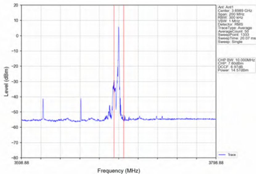
n78d 30kHz SISO NTN 80MHz CP-OFDM 16 QAM 3660MHz Edge 1RB Right
