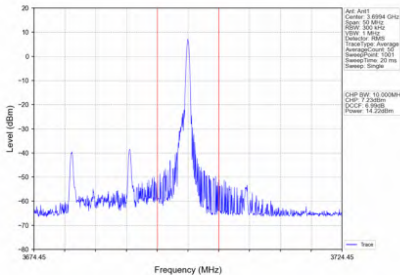
n78d 15kHz SISO NTNv 20MHz DFT-s-OFDM QPSK 3690MHz Edge 1RB Right
