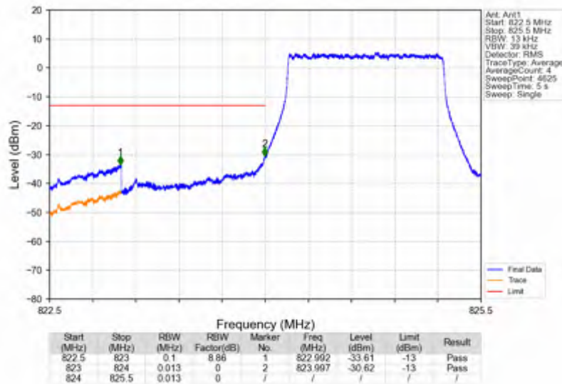
Band26b 1.4MHz QPSK LCH 824.7MHz RB 6 0 NTNV
