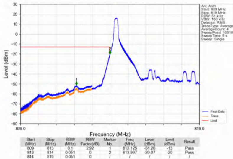
Band26a 5MHz 64QAM LCH 816.5MHz RB 25 0 NTNV
