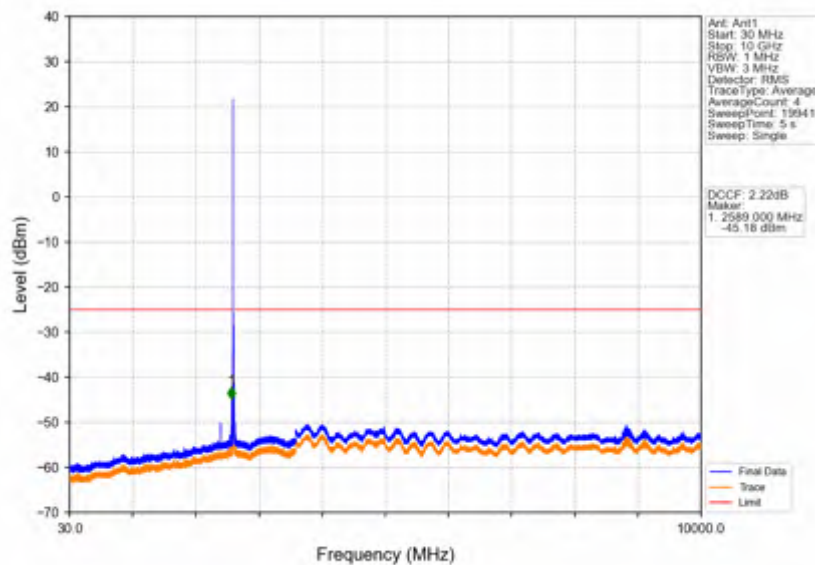
Band38_10MHz_QPSK_HCH_2615MHz_RB_1_0_NTNV
