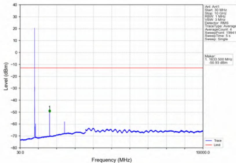
Band26a 5MHz_QPSK_MCH_819MHz_RB_1_0_NTNV
