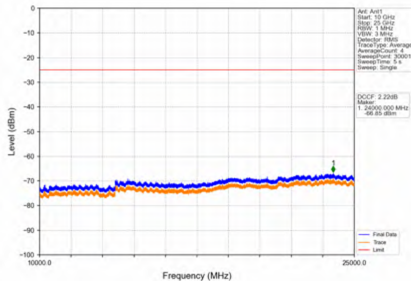
Band38_5MHz_QPSK_MCH_2595MHz_RB_1_0_NTNV
