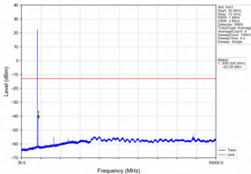
Band26b_5MHz_QPSK_HCH_846.5MHz_RB_1_24_NTNV
