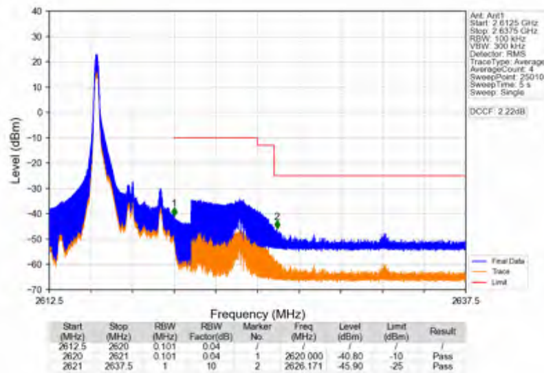
Band38_5MHz_QPSK_HCH_2617.5MHz_RB_1_24_NTNV
