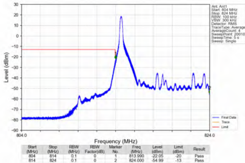
Band26a 10MHz QPSK LCH 819MHz RB 50 0 NTNV
