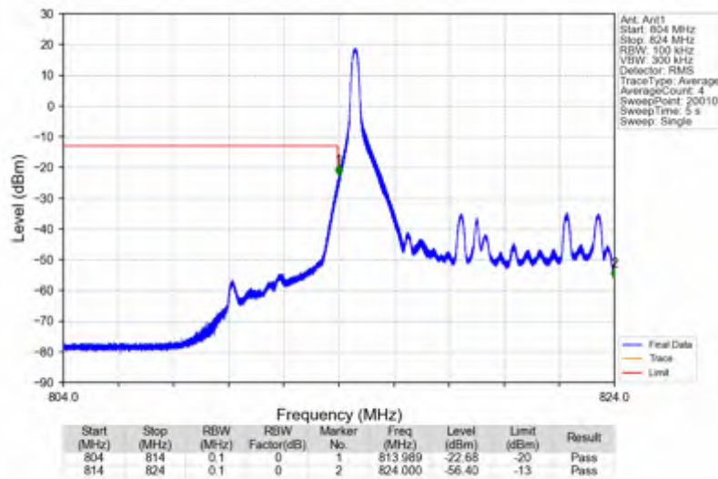
Band26a_10MHz_QPSK_LCH_819MHz_RB_1_0_NTNV
