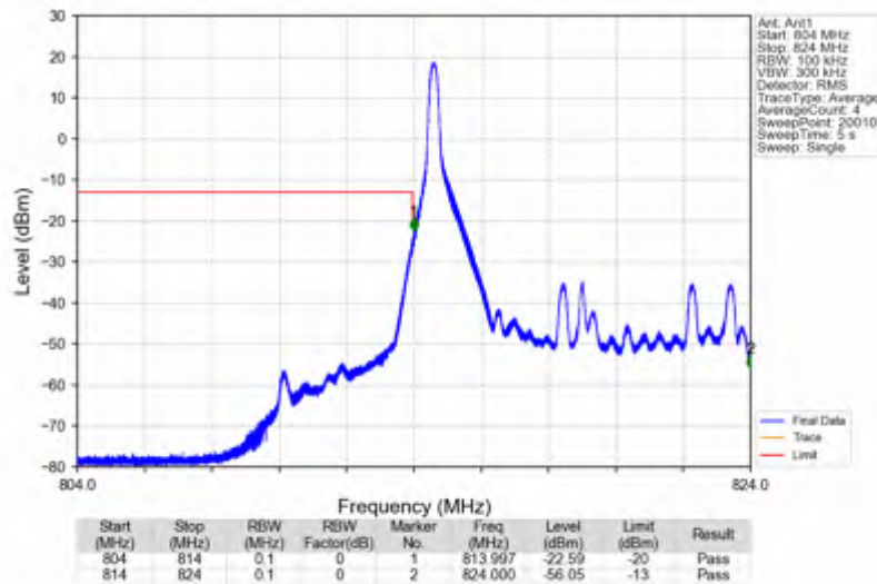
Band26a 10MHz 64QAM LCH 819MHz RB 1 0 NTNV
