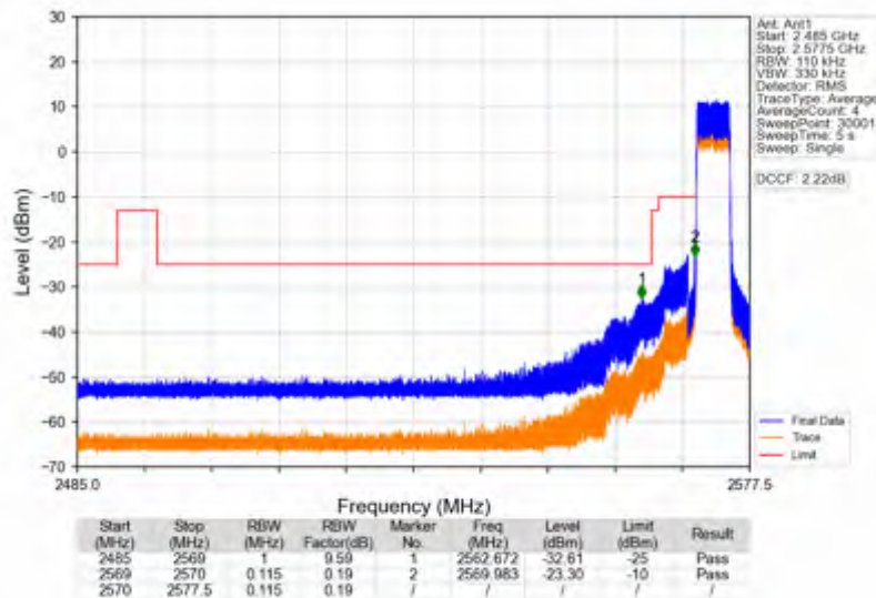
Band38_5MHz_QPSK_LCH_2572.5MHz_RB_1_0_NTNV
