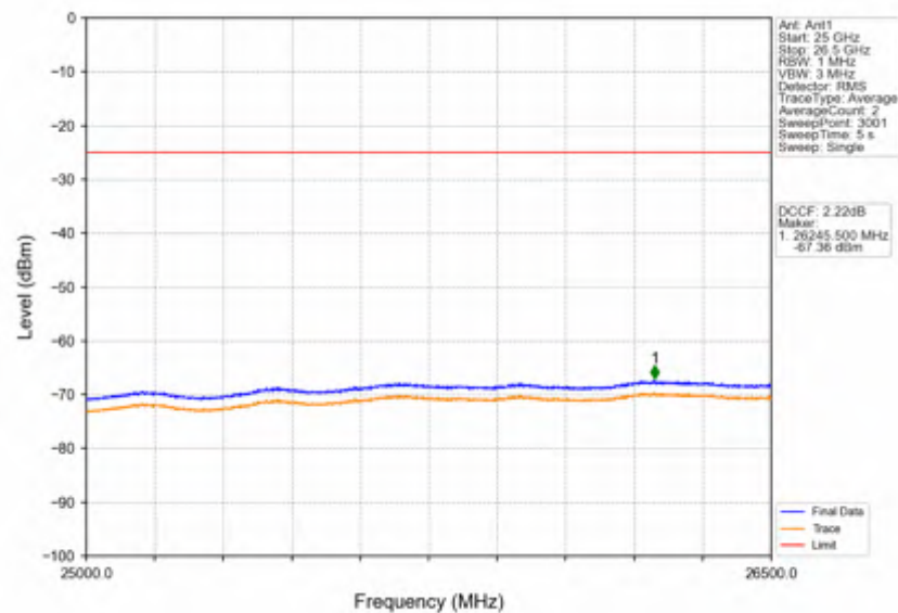
Band38_5MHz_QPSK_HCH_2617.5MHz_RB_1_24_NTNV
