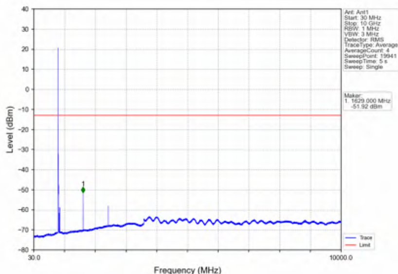
Band26a 10MHz 16QAM HCH 819MHz RB 1 0 NTNV
