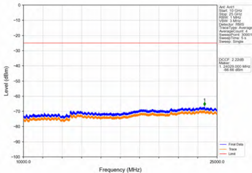
Band38_10MHz_QPSK_HCH_2615MHz_RB_1_0_NTNV
