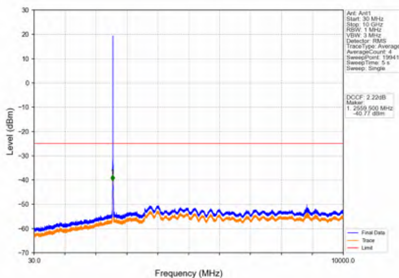
Band38_5MHz_QPSK_LCH_2572.5MHz_RB_1_0_NTNV
