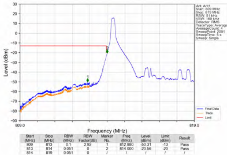
Band26a 5MHz 64QAM LCH 816.5MHz RB 1 0 NTNV
