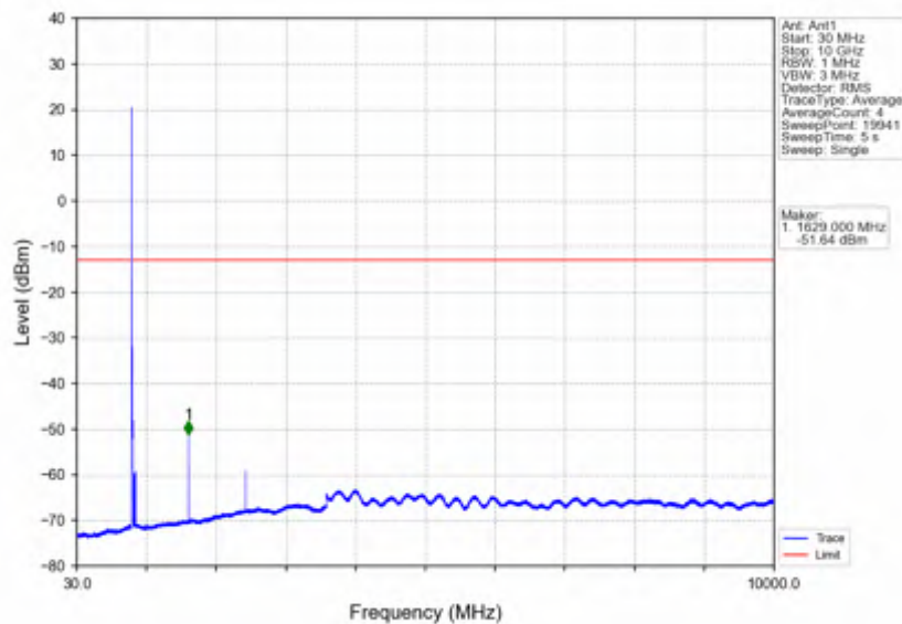
Band26a_10MHz_QPSK_HCH_819MHz_RB_1_49_NTNV
