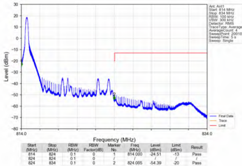
Band26a_10MHz_QPSK_HCH_819MHz_RB_1_49_NTNV
