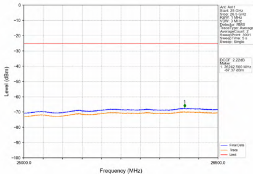
Band38_5MHz_QPSK_LCH_2572.5MHz_RB_1_0_NTNV
