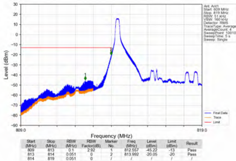
Band26a 5MHz QPSK LCH 816.5MHz RB 25 0 NTNV
