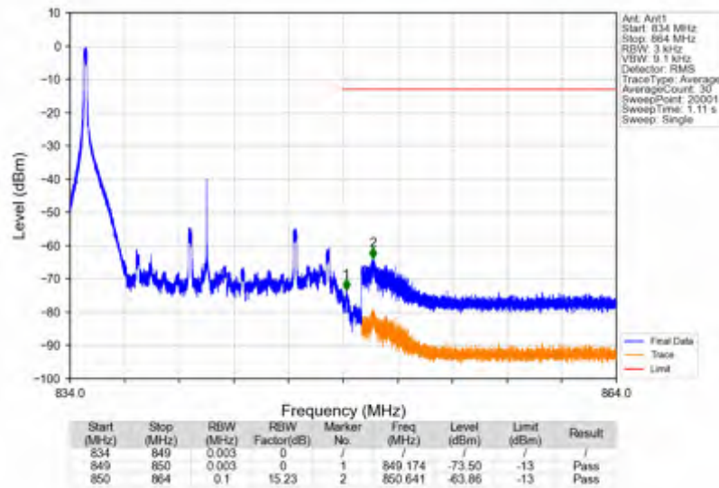
Band26c_15MHz_16QAM_HCH_841.5MHz_RB_1_74_NTNV
