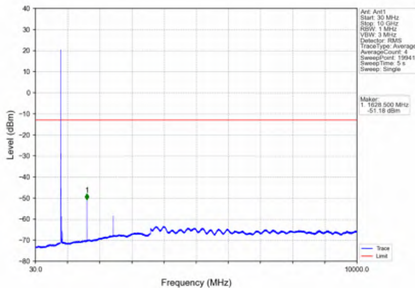
Band26a 5MHz 64QAM LCH 816.5MHz RB 1 0 NTNV
