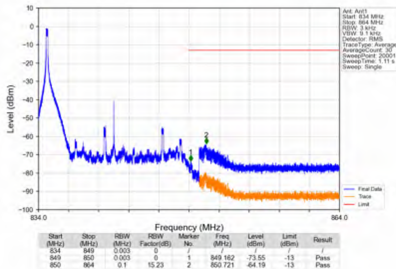
Band26c_15MHz_QPSK_HCH_841.5MHz_RB_1_74_NTNV
