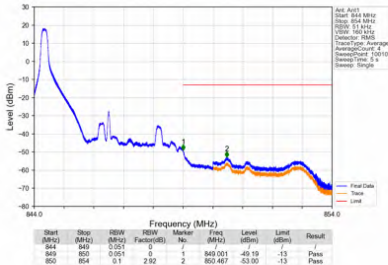
Band26b_5MHz_QPSK_HCH_846.5MHz_RB_1_24_NTNV
