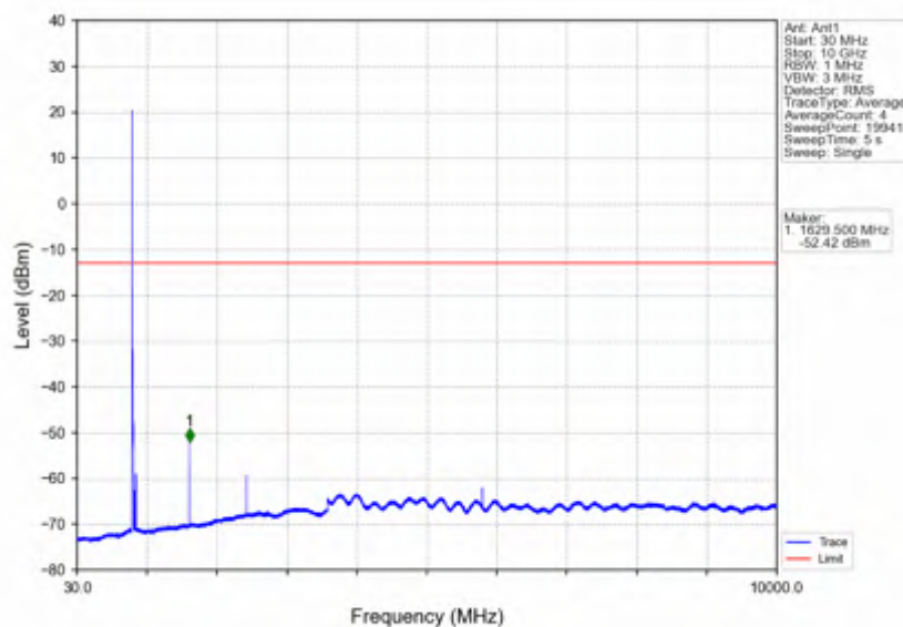
Band26a_10MHz_QPSK_LCH_819MHz_RB_1_0_NTNV
