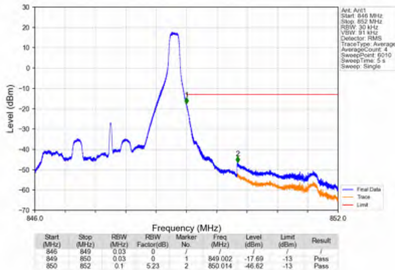
Band26b_3MHz_QPSK_HCH_847.5MHz_RB_1_14_NTNV
