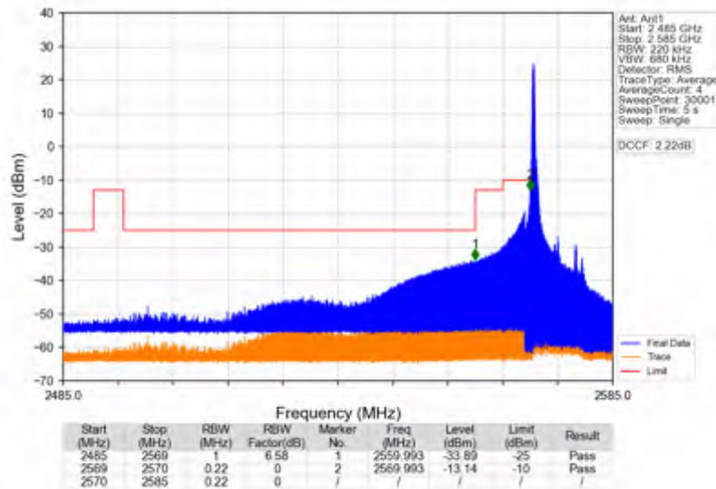
Band38_10MHz_QPSK_LCH_2575MHz_RB_50_0_NTNV
