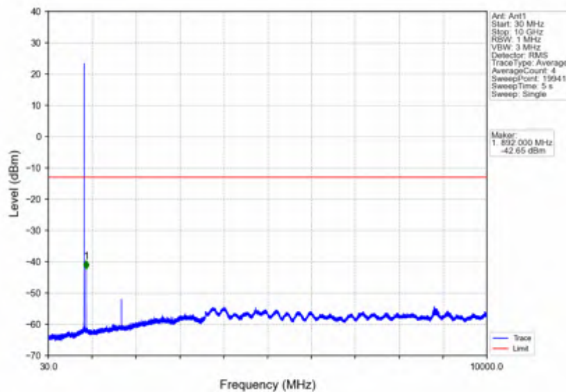
Band26b_3MHz_QPSK_HCH_847.5MHz_RB_1_14_NTNV
