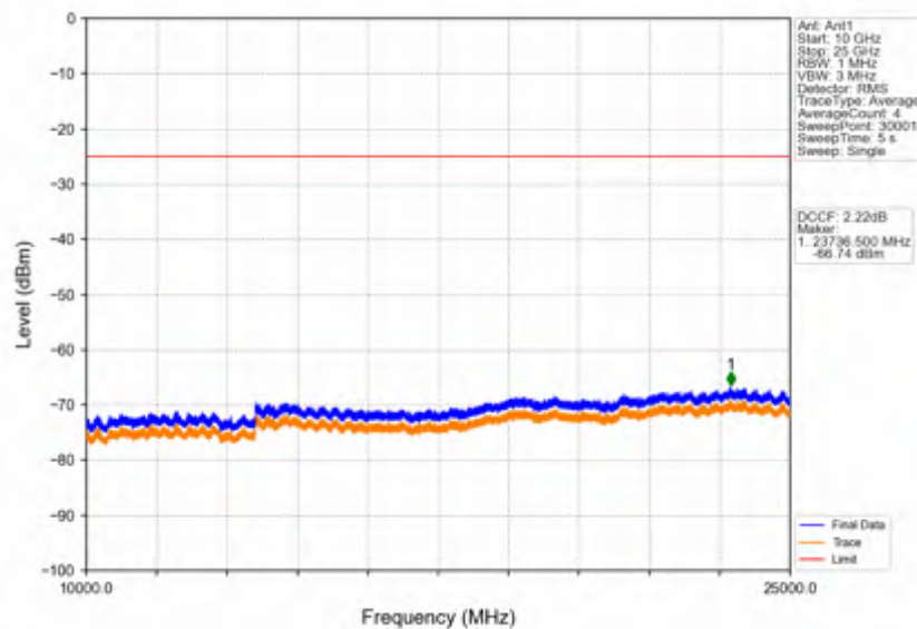
Band38_10MHz_QPSK_MCH_2595MHz_RB_1_0_NTNV
