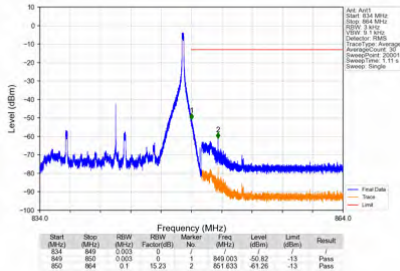
Band26c_15MHz_256QAM_HCH_841.5MHz_RB_1_74_NTNV
