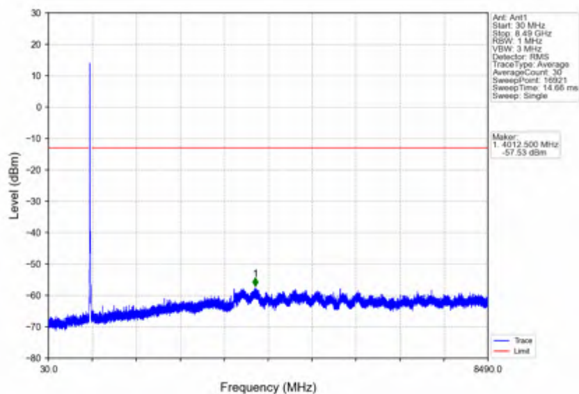
Band26c_15MHz_QPSK_LCH_831.5MHz_RB_1_0_NTNV
