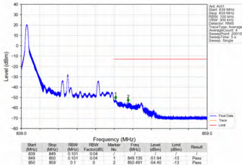
Band26b_10MHz_QPSK_HCH_844MHz_RB_1_49_NTNV
