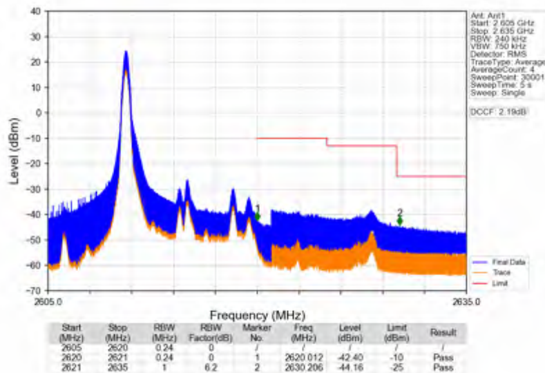
Band38_10MHz_QPSK_HCH_2615MHz_RB_1_49_NTNV
