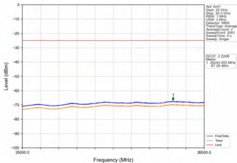
Band38_10MHz_QPSK_HCH_2615MHz_RB_1_49_NTNV
