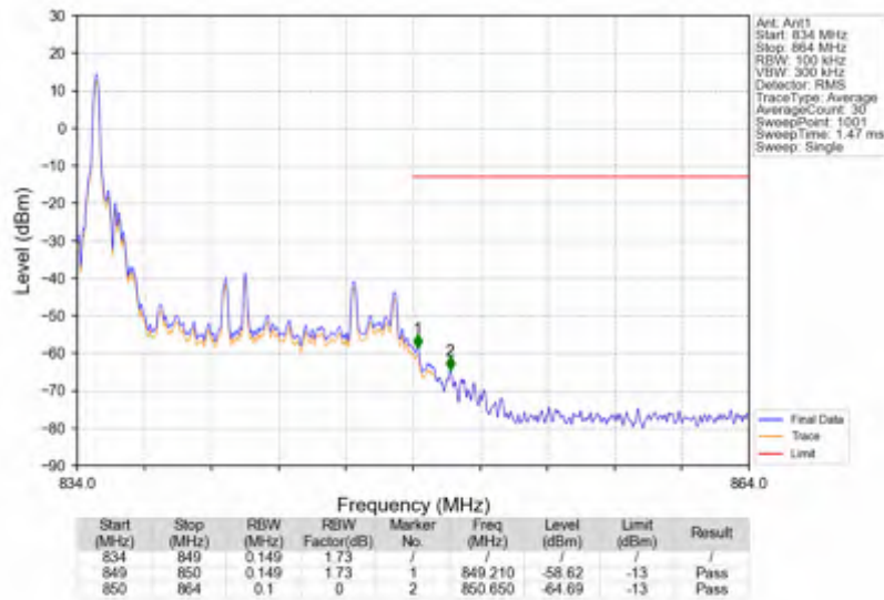
Band26c_15MHz_QPSK_HCH_841.5MHz_RB_75_0_NTNV
