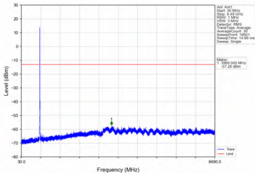
Band26c_15MHz_QPSK_HCH_841.5MHz_RB_1_74_NTNV
