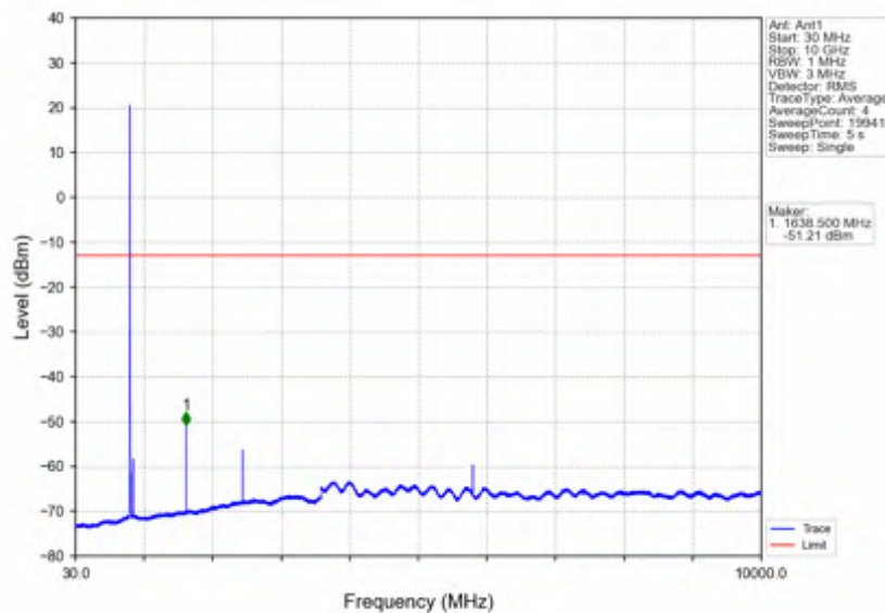
Band26a 5MHz 16QAM HCH 821.5MHz RB 1 0 NTNV
