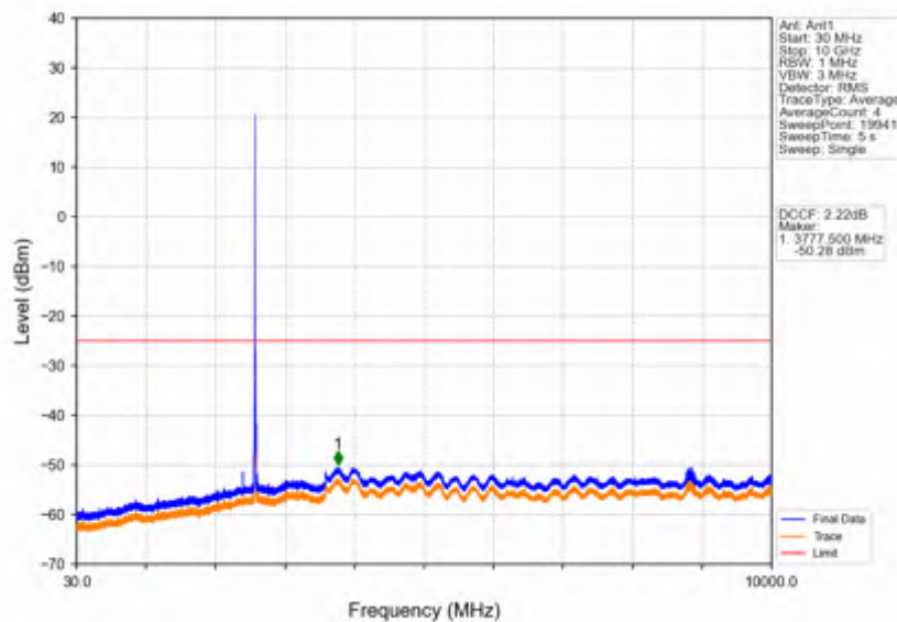
Band38_10MHz_QPSK_MCH_2595MHz_RB_1_0_NTNV
