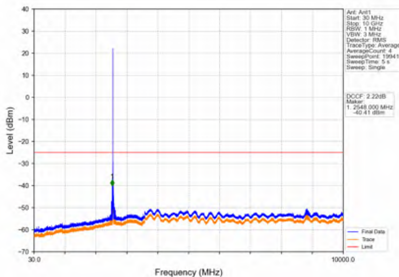
Band38_10MHz_QPSK_LCH_2575MHz_RB_1_0_NTNV
