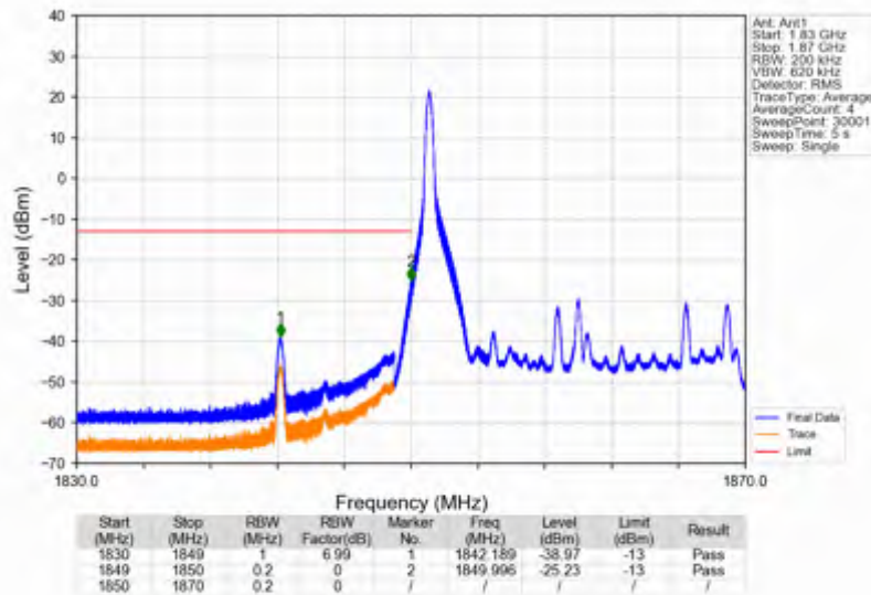
Band25 20MHz 64QAM LCH 1860MHz RB 1 0 NTNV
