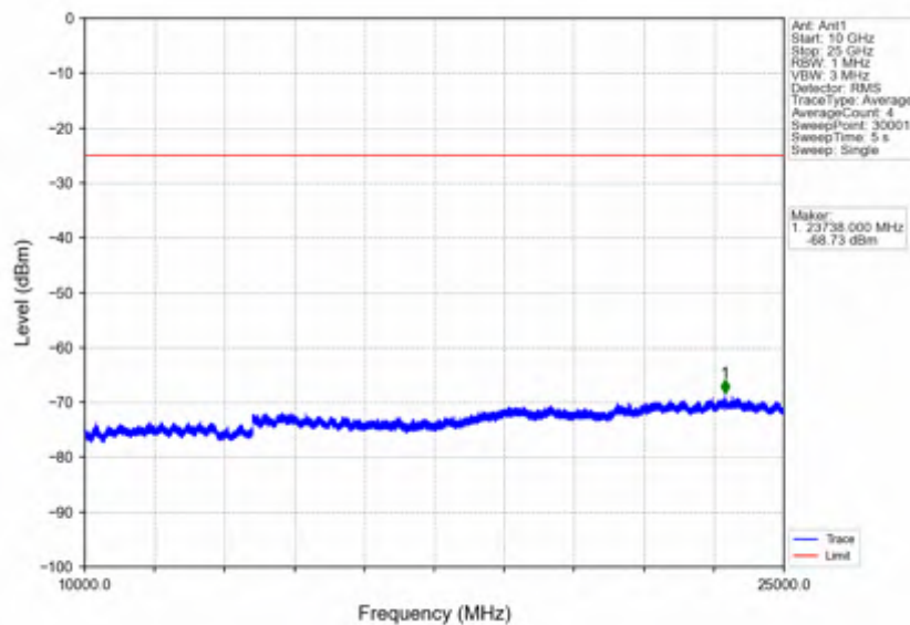
Band7_20MHz_256QAM_MCH_2535MHz_RB_1_0_NTNV
