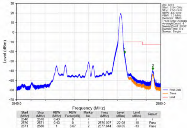
Band7_20MHz_256QAM_HCH_2560MHz_RB_1_99_NTNV
