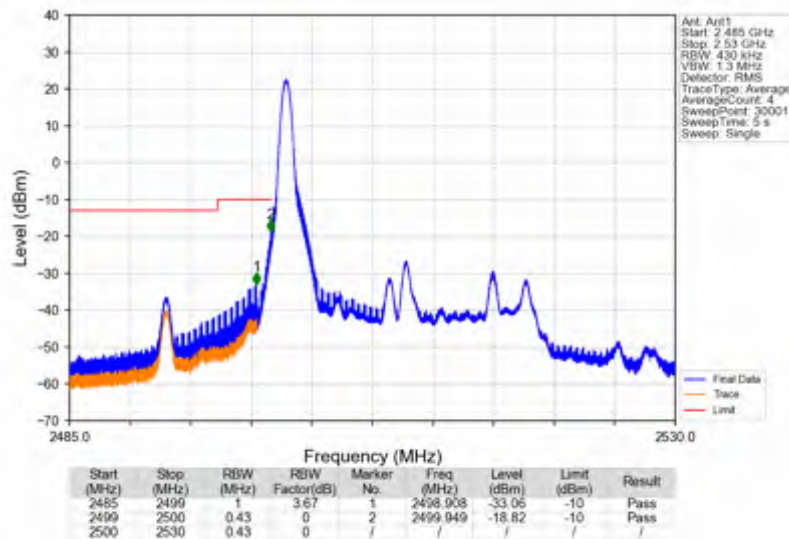
Band7_20MHz_QPSK_LCH_2510MHz_RB_1_0_NTNV
