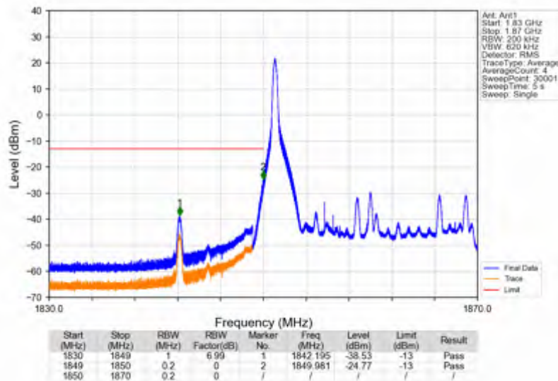
Band25 20MHz QPSK LCH 1860MHz RB 1 0 NTNV
