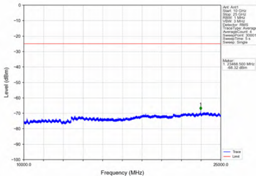
Band7_20MHz_256QAM_LCH_2510MHz_RB_1_0_NTNV
