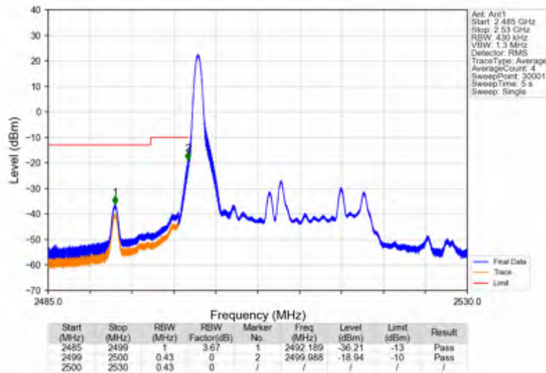
Band7 20MHz 64QAM LCH 2510MHz RB 100 0 NTNV
