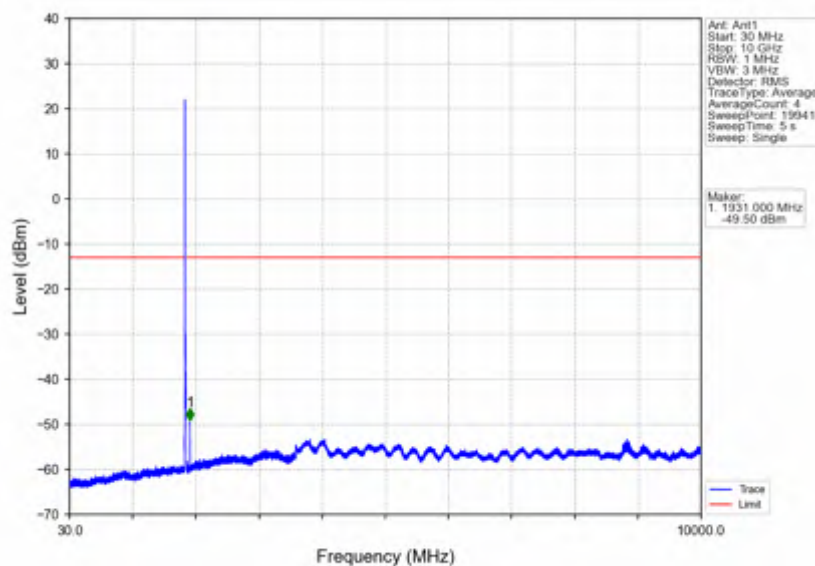
Band25 10MHz QPSK LCH 1855MHz RB 1 0 NTNV
