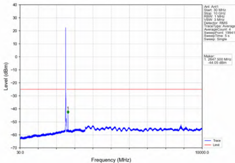
Band7 20MHz 64QAM MCH 2535MHz RB 1 0 NTNV
