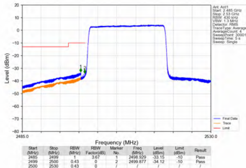
Band7_20MHz_256QAM_LCH_2510MHz_RB_100_0_NTNV
