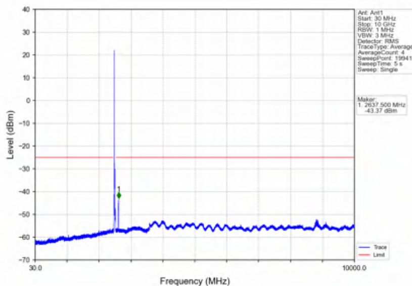
Band7_20MHz_QPSK_LCH_2510MHz_RB_1_0_NTNV
