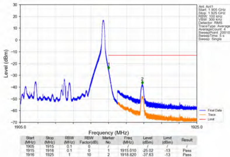
Band25 10MHz 256QAM HCH 1910MHz RB 1 49 NTNV
