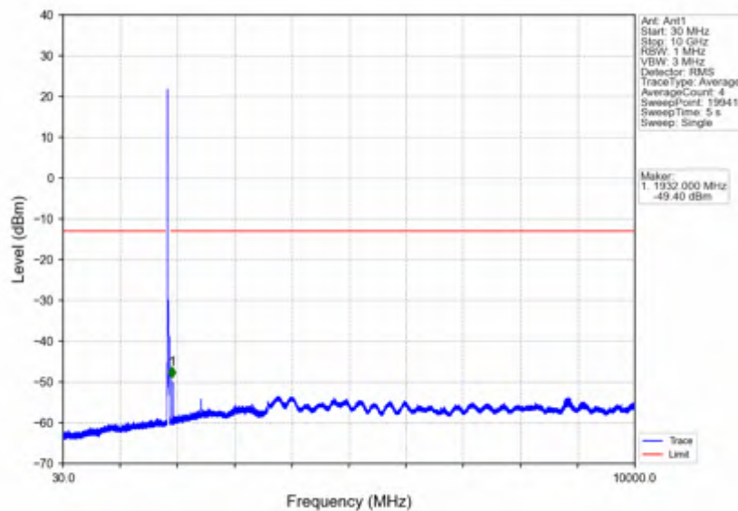
Band25 20MHz 64QAM LCH 1860MHz RB 1 0 NTNV
