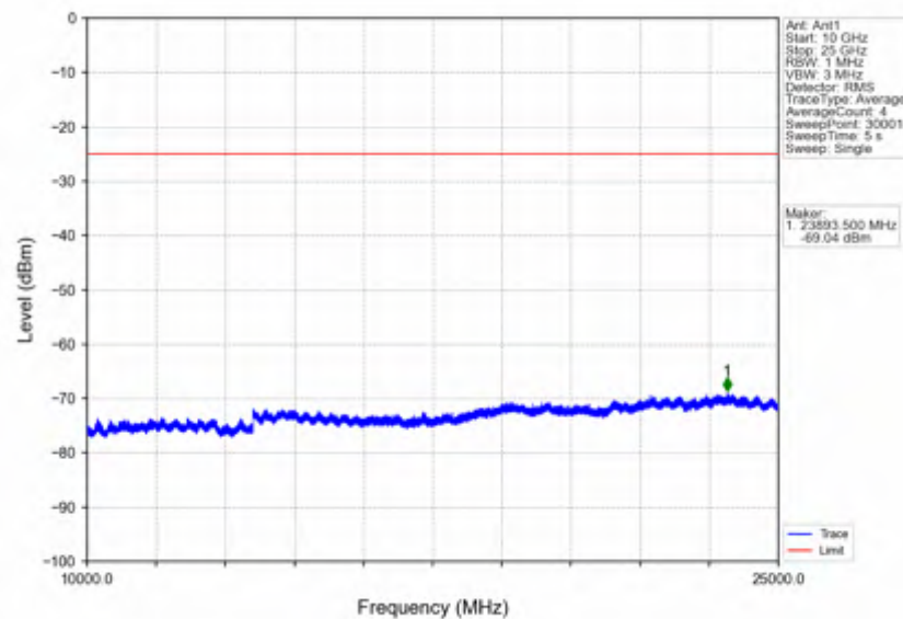
Band7_20MHz_QPSK_MCH_2535MHz_RB_1_0_NTNV
