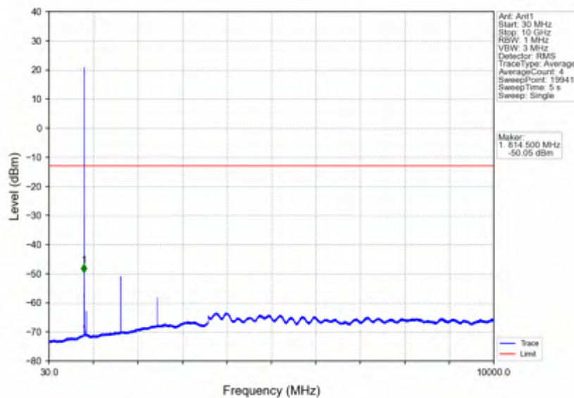
Band26a 1.4MHz QPSK MCH 819MHz RB 1 0 NTNV
