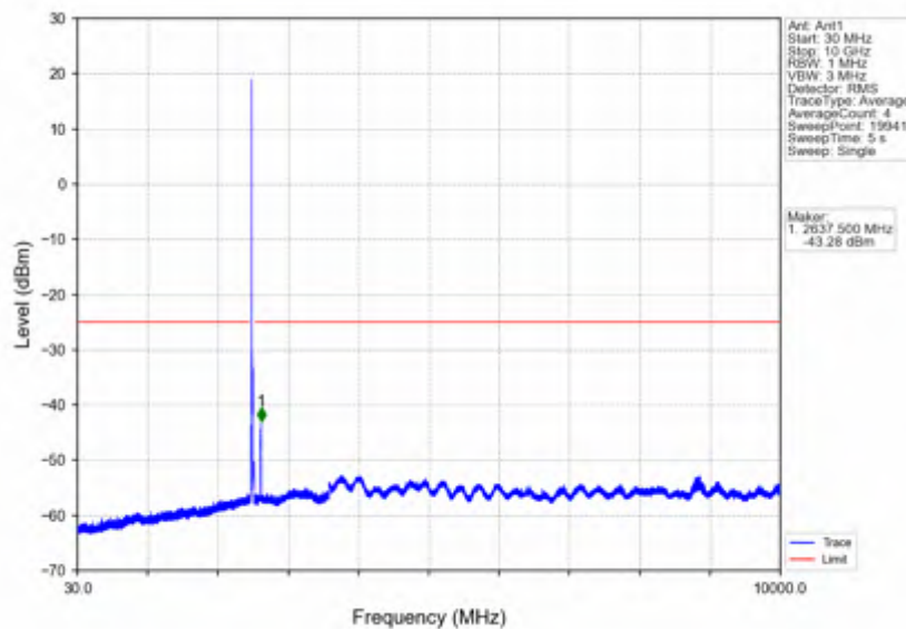
Band7_20MHz_256QAM_LCH_2510MHz_RB_1_0_NTNV
