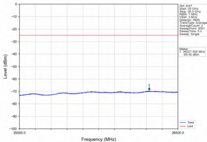
Band7_20MHz_256QAM_HCH_2560MHz_RB_1_0_NTNV
