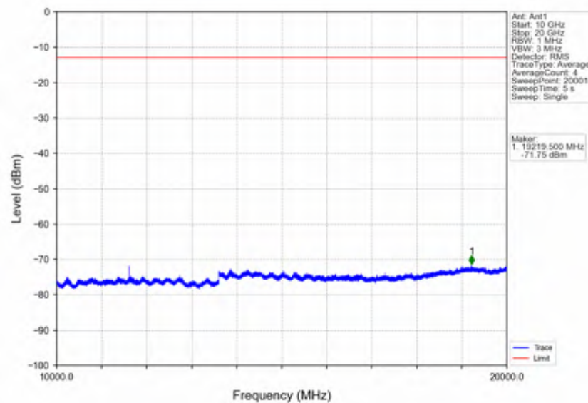
Band25 20MHz QPSK LCH 1860MHz RB 100 0 NTN
