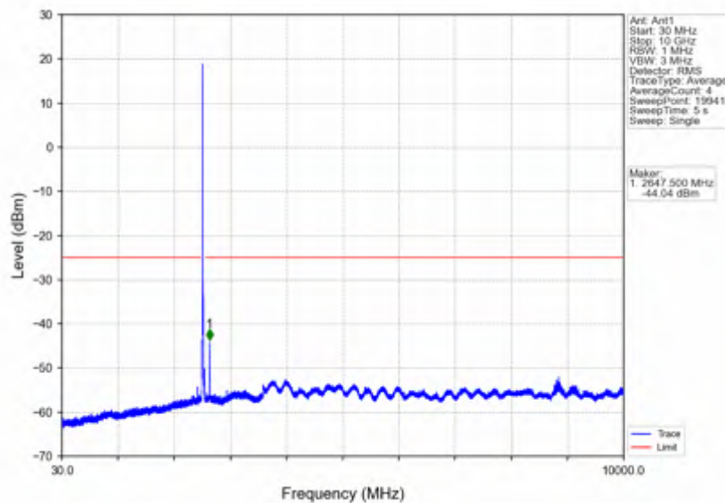
Band7_20MHz_256QAM_MCH_2535MHz_RB_1_0_NTNV
