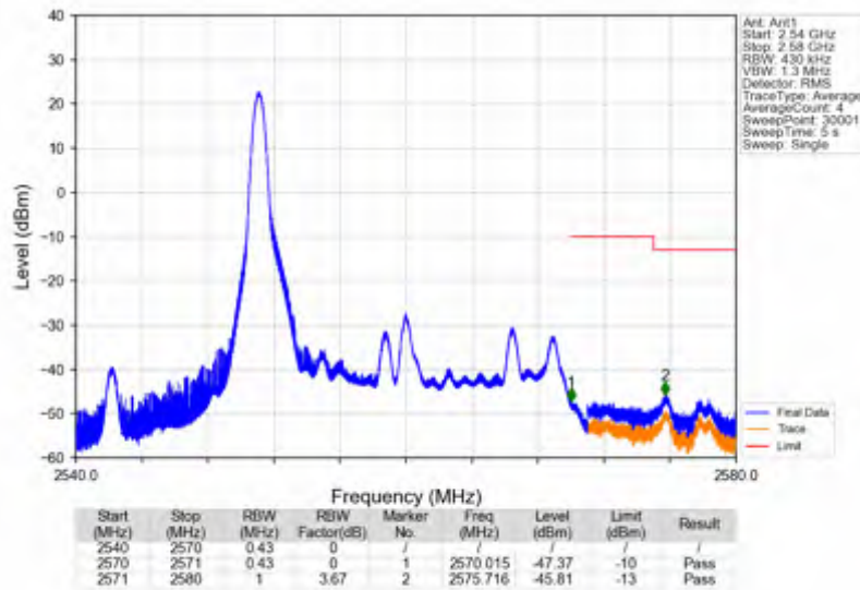
Band7_20MHz_QPSK_HCH_2560MHz_RB_100_0_NTNV
