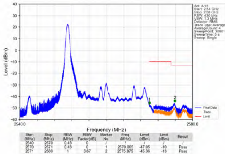
Band7_20MHz_QPSK_HCH_2560MHz_RB_1_99_NTNV
