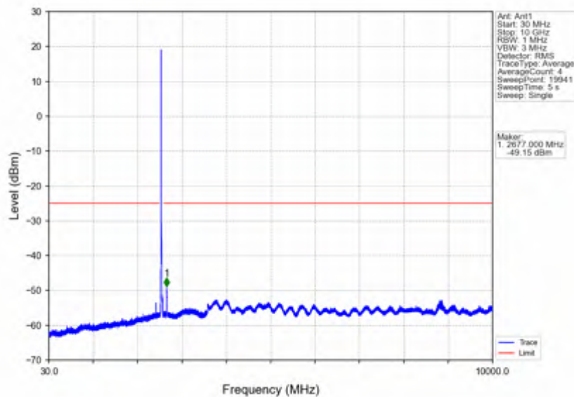
Band7_20MHz_256QAM_HCH_2560MHz_RB_1_0_NTNV
