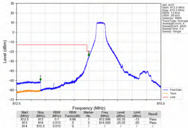
Band26a 1.4MHz QPSK LCH 814.7MHz RB 6 0 NTNV
