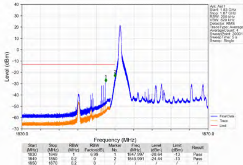
Band25 20MHz QPSK LCH 1860MHz RB 100 0 NTN
