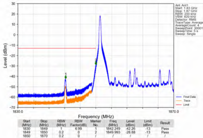
Band25 20MHz 256QAM LCH 1860MHz RB 1 0 NTNV
