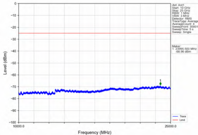
Band7_20MHz_256QAM_HCH_2560MHz_RB_1_0_NTV
