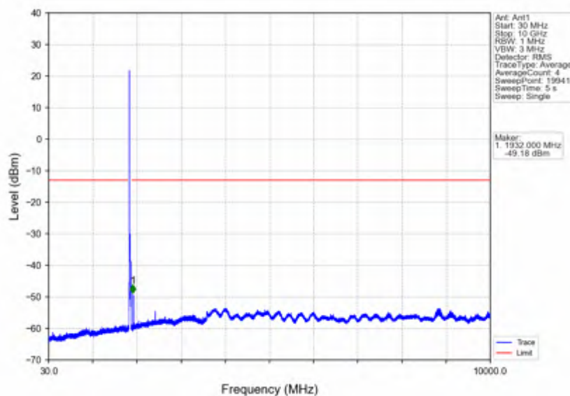
Band25 20MHz QPSK LCH 1860MHz RB 1 0 NTNV
