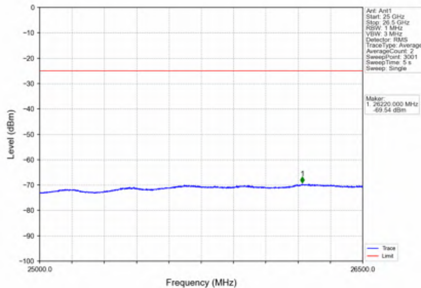
Band7_20MHz_QPSK_LCH_2510MHz_RB_1_0_NTNV
