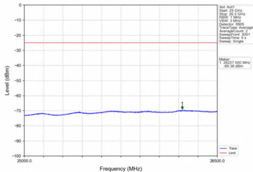
Band7_20MHz_64QAM_HCH_2560MHz_RB_1_99_NTNV
