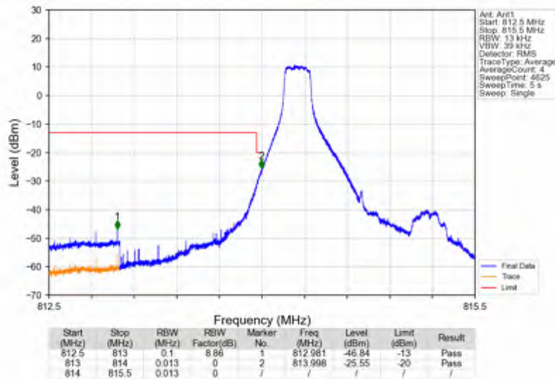
Band26a 1.4MHz 64QAM LCH 814.7MHz RB 1 0 NTNV
