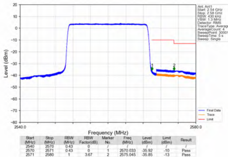
Band7_20MHz_256QAM_HCH_2560MHz_RB_100_0_NTNV
