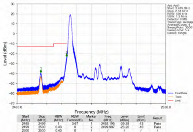
Band7_20MHz_256QAM_LCH_2510MHz_RB_1_0_NTNV
