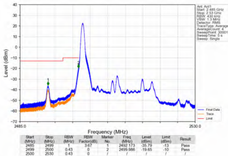
Band7_20MHz_16QAM_LCH_2510MHz_RB_1_0_NTNV
