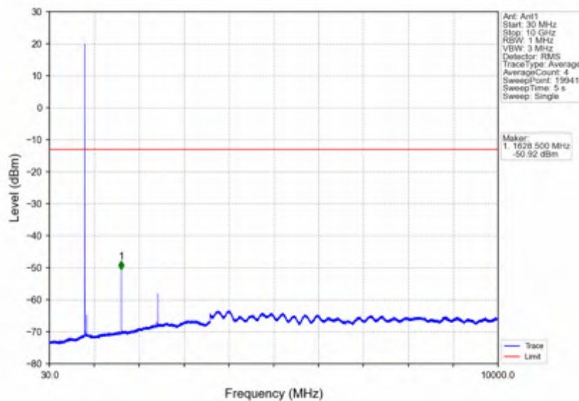
Band26a 1.4MHz 64QAM LCH 814.7MHz RB 1 0 NTNV
