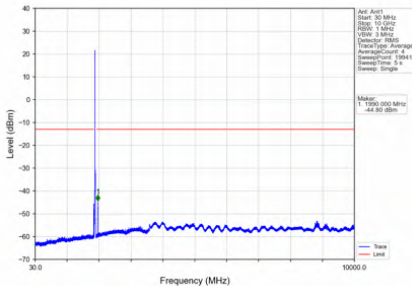
Band25_20MHz_QPSK_HCH_1905MHz_RB_1_0_NTNV
