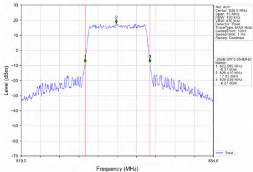
Band5 5MHz 16QAM LCH 826.5MHz RB 25 0 NTNV
