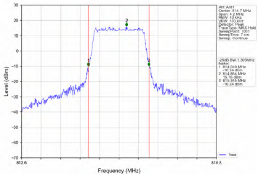
Band26a 1.4MHz 16QAM LCH 814.7MHz RB 6 0 NTNV
