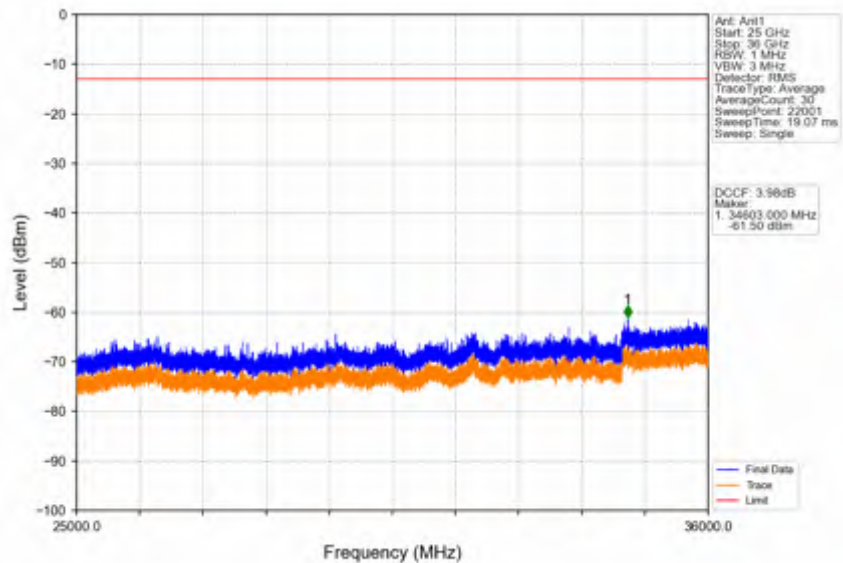
Band42c_20MHz_QPSK_MCH_3575MHz_RB_1_0_NTV
