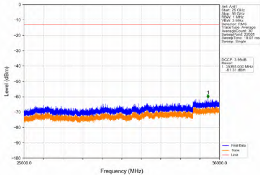
Band42c_10MHz_QPSK_HCH_3595MHz_RB_1_49_NTNV
