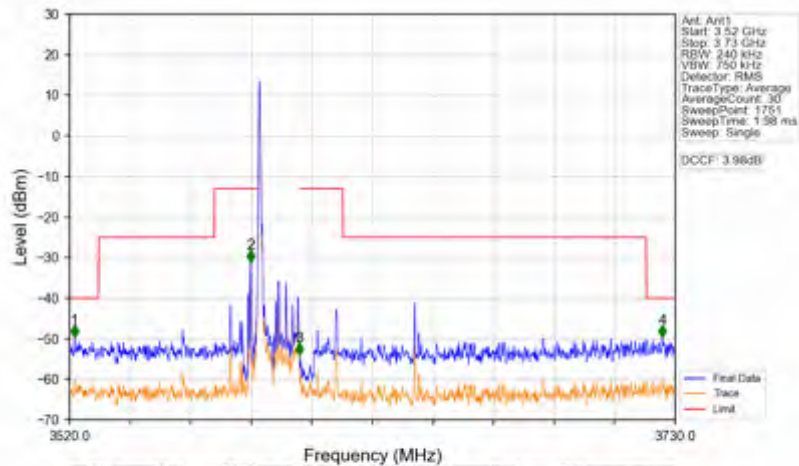
Band42c_15MHz_QPSK_HCH_3592.5MHz_RB_1_74_NTNV
