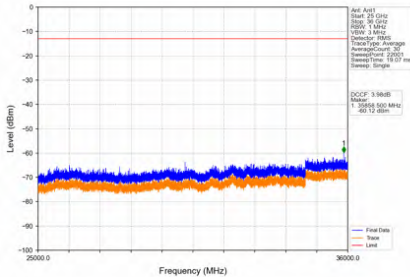
Band42c_20MHz_16QAM_LCH_3560MHz_RB_100_0_NTNV
