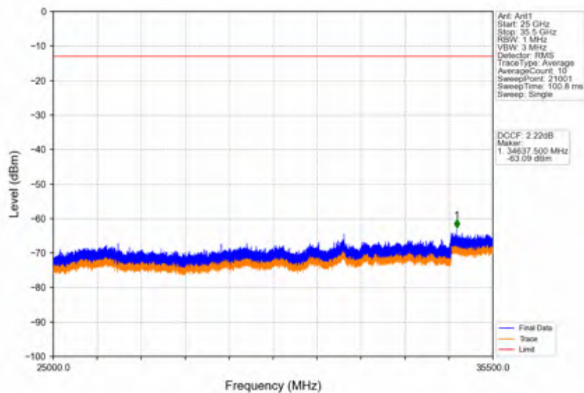
Band42a_20MHz_QPSK_LCH_3460MHz_RB_1_0_NTNV
