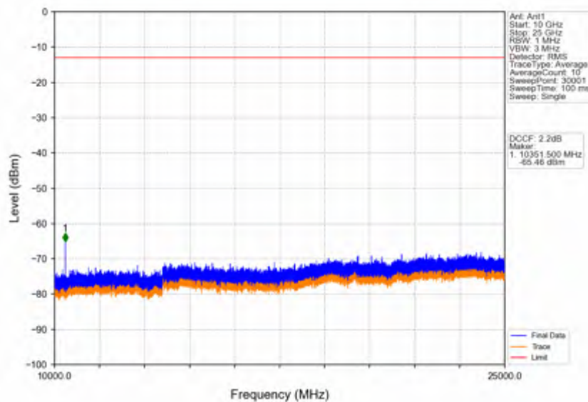
Band42a_10MHz_256QAM_LCH_3455MHz_RB_1_0_NTNV
