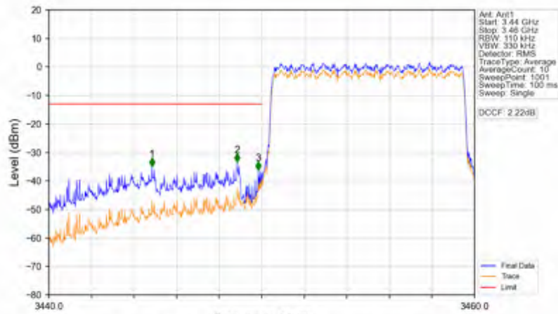
Band42a_10MHz_256QAM_LCH_3455MHz_RB_50_0_NTNV
