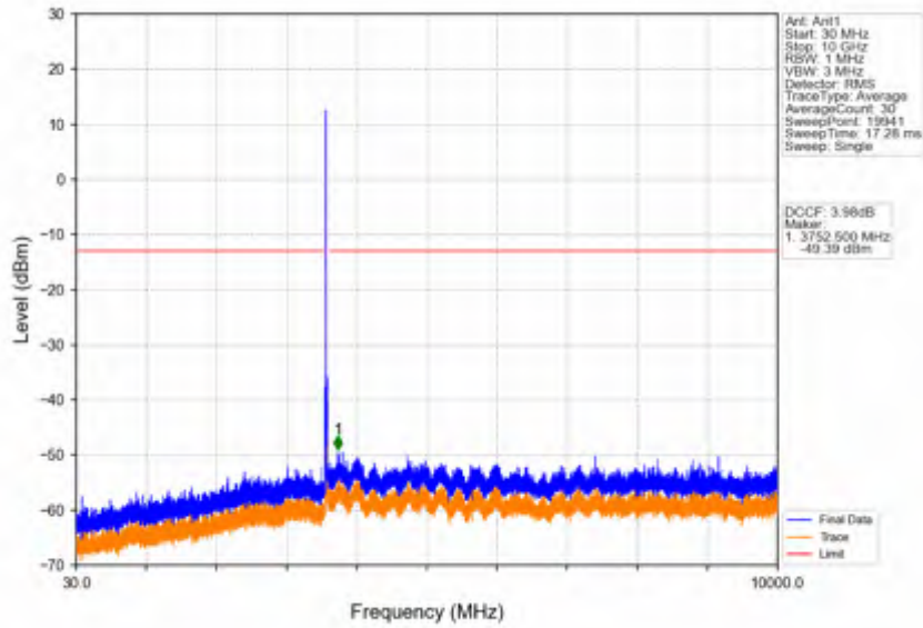
Band42c_20MHz_QPSK_HCH_3590MHz_RB_1_0_NTV
