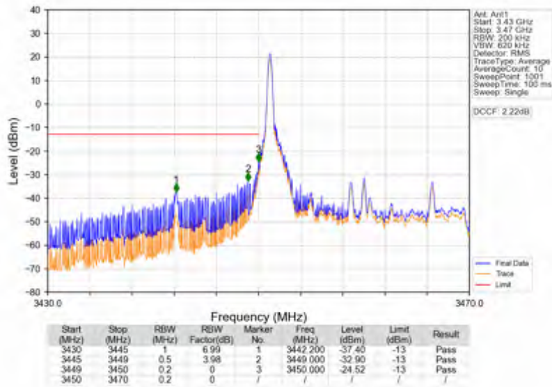
Band42a_20MHz_16QAM_LCH_3460MHz_RB_1_0_NTNV
