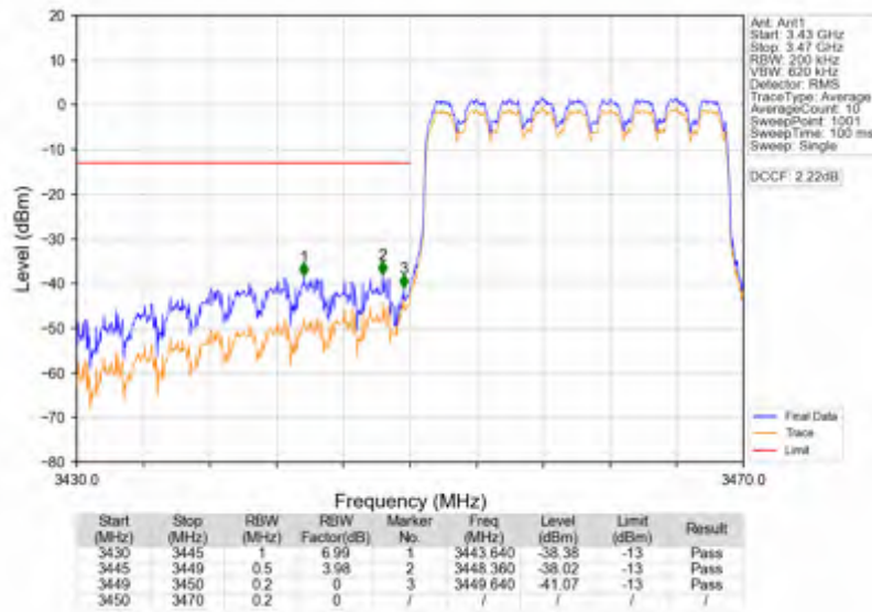
Band42a_20MHz_256QAM_LCH_3460MHz_RB_100_0_NTNV
