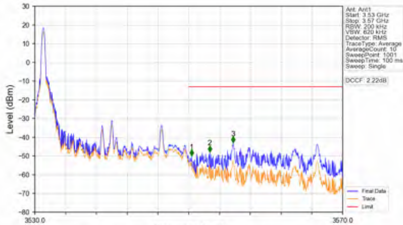
Band42a_20MHz_QPSK_HCH_3540MHz_RB_1_99_NTV
