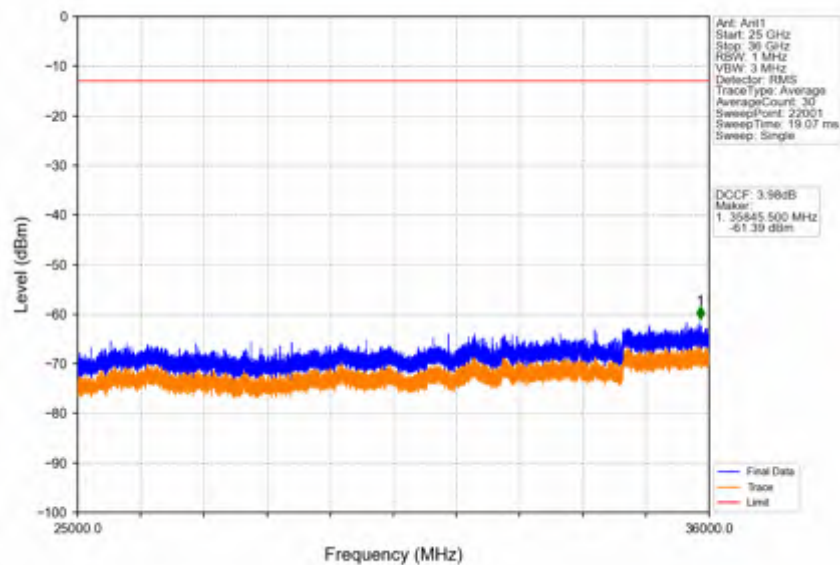
Band42c_10MHz_QPSK_LCH_3555MHz_RB_1_0_NTNV
