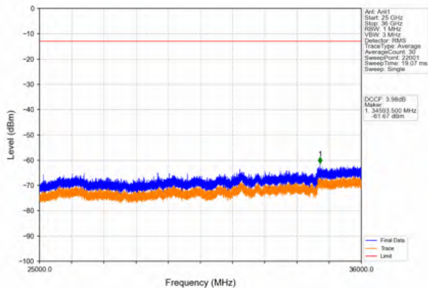
Band42c_20MHz_QPSK_LCH_3560MHz_RB_1_0_NTNV
