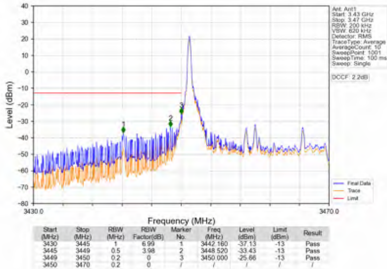
Band42a_20MHz_16QAM_LCH_3460MHz_RB_100_0_NTNV
