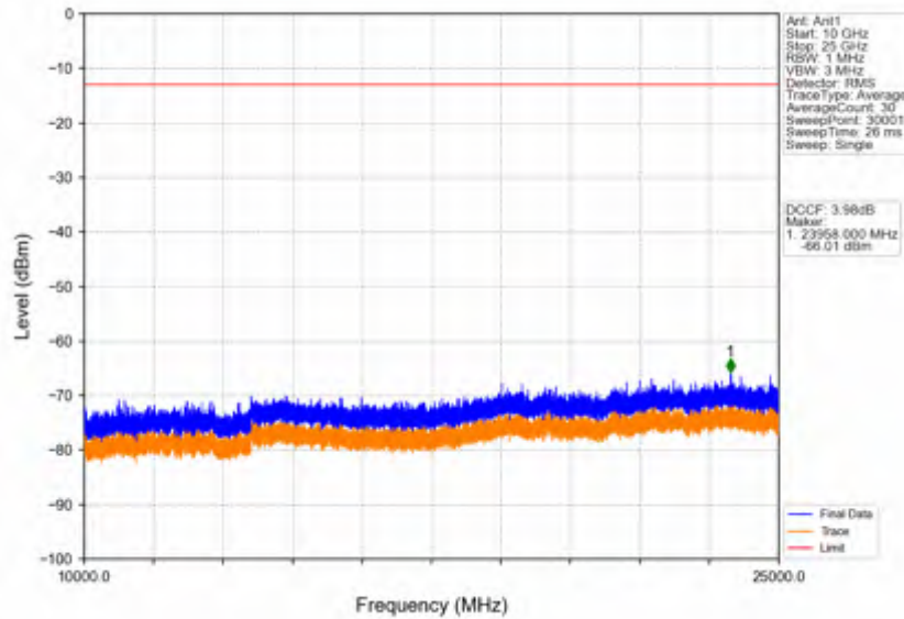
Band42c_20MHz_QPSK_HCH_3590MHz_RB_1_0_NTV
