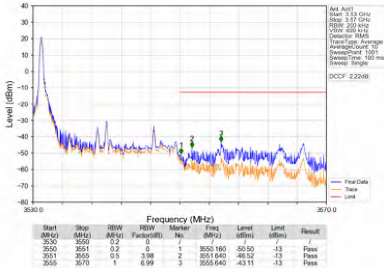
Band42a_20MHz_QPSK_HCH_3540MHz_RB_100_0_NTNV
