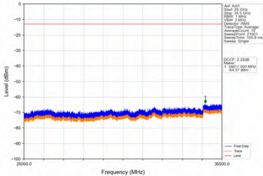
Band42a_20MHz_16QAM_LCH_3460MHz_RB_100_0_NTNV
