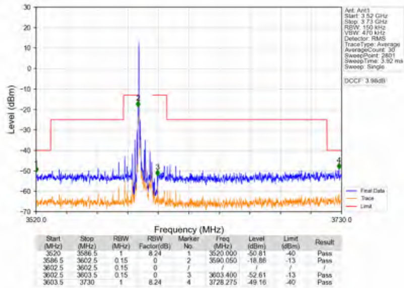
Band42c_10MHz_QPSK_HCH_3595MHz_RB_1_49_NTNV
