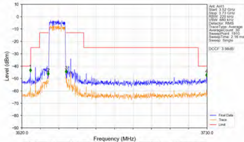
Band42c_20MHz_16QAM_LCH_3560MHz_RB_100_0_NTNV
