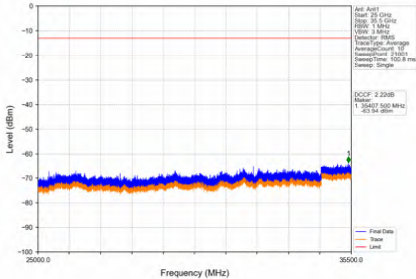
Band42a_20MHz_QPSK_HCH_3540MHz_RB_1_99_NTV
