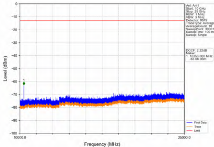
Band42a_20MHz_256QAM_LCH_3460MHz_RB_1_0_NTNV
