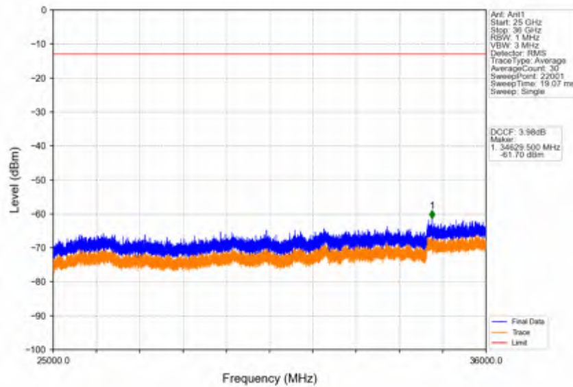
Band42c_20MHz_256QAM_LCH_3560MHz_RB_100_0_NTNV
