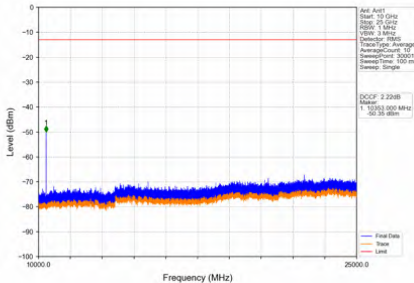
Band42a_20MHz_16QAM_LCH_3460MHz_RB_1_0_NTNV
