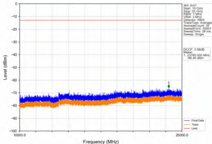
Band42c_20MHz_QPSK_MCH_3575MHz_RB_1_0_NTV
