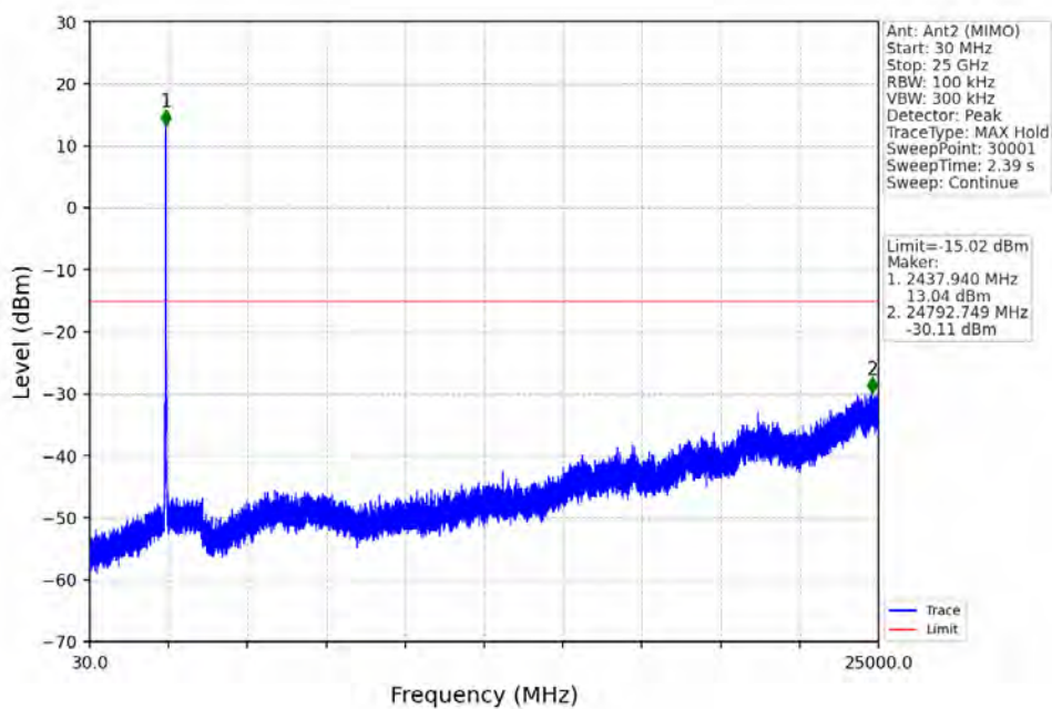
802.11b_MCH_2437MHz_Ant2 (MIMO)_NTNV
