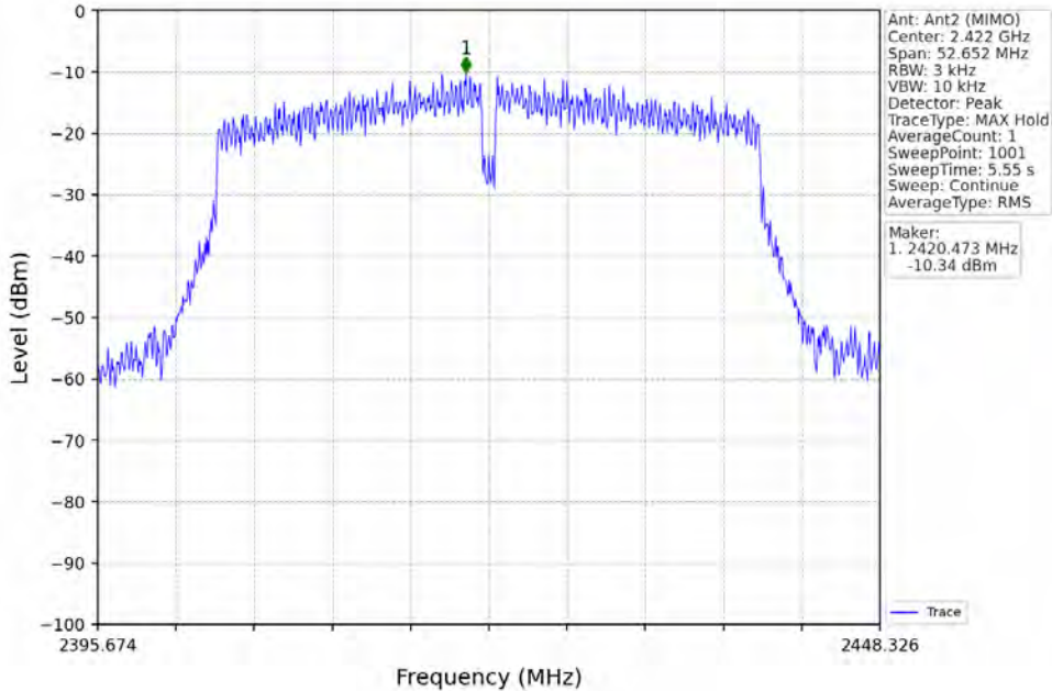
802.11n(HT40)_LCH_2422MHz_MIMO_NTNV
