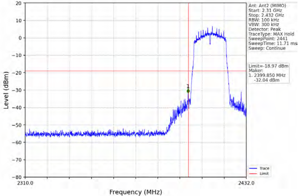
802.11n(HT20)_LCH_2412MHz_Ant2 (MIMO)_NTNV
