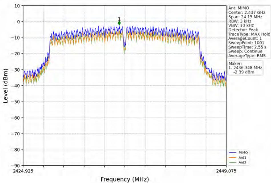
802.11n(HT20)_MCH_2437MHz_MIMO_NTNV
