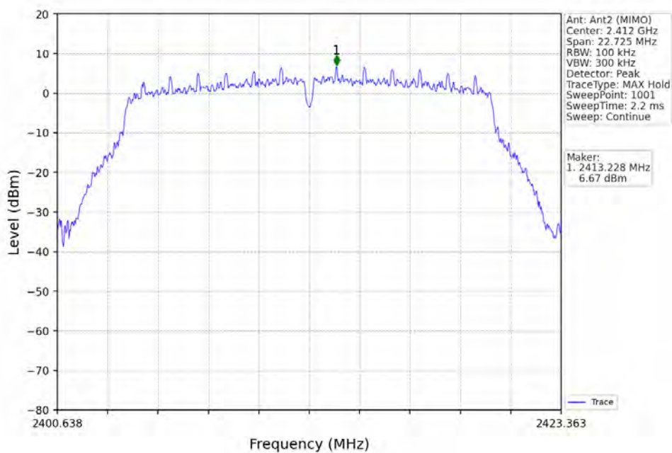
802.11g_LCH_2412MHz_Ant2 (MIMO)_NTNV
