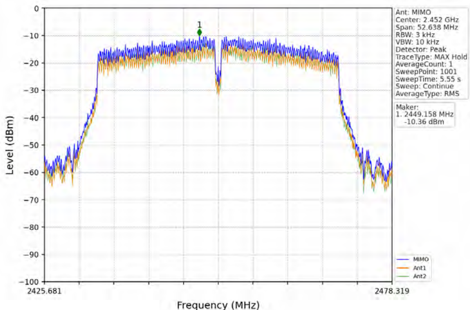
802.11n(HT40)_HCH_2452MHz_MIMO_NTNV
