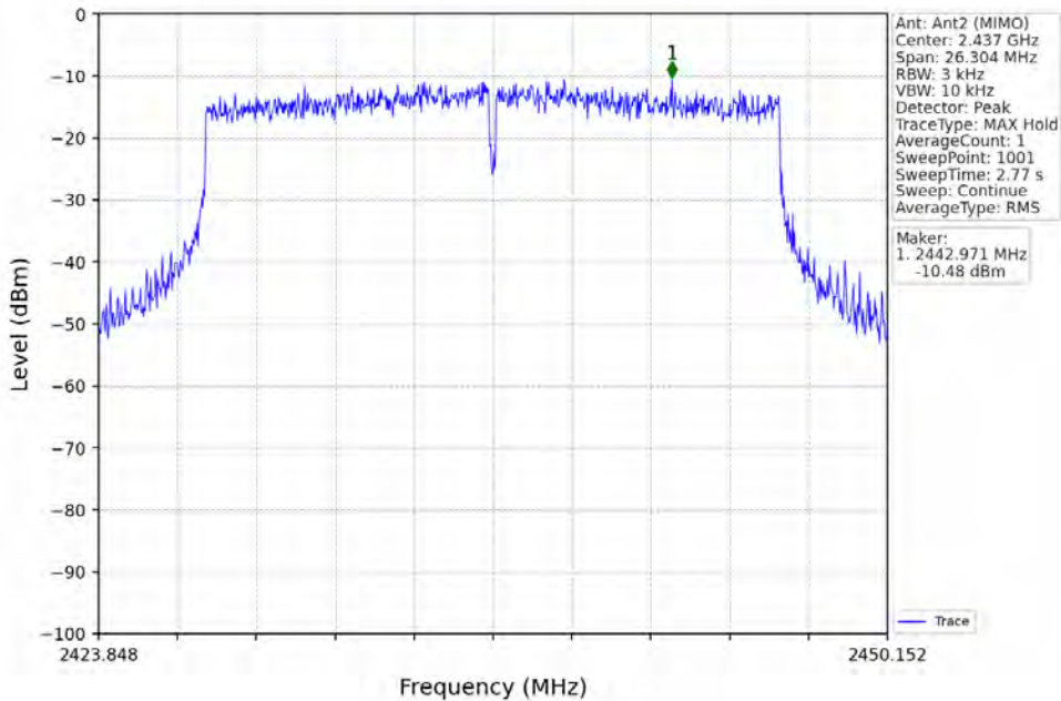
802.11ax(HEW20)_MCH_2437MHz_RU242_Left_MIMO_NTNV
