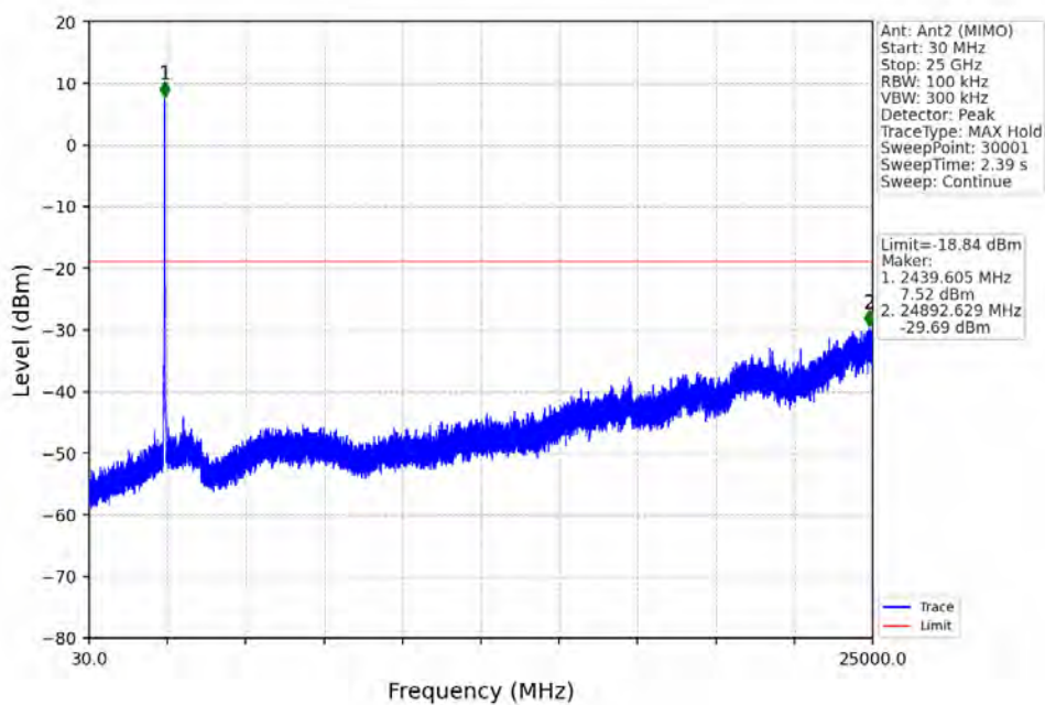
802.11g_MCH_2437MHz_Ant2 (MIMO)_NTNV
