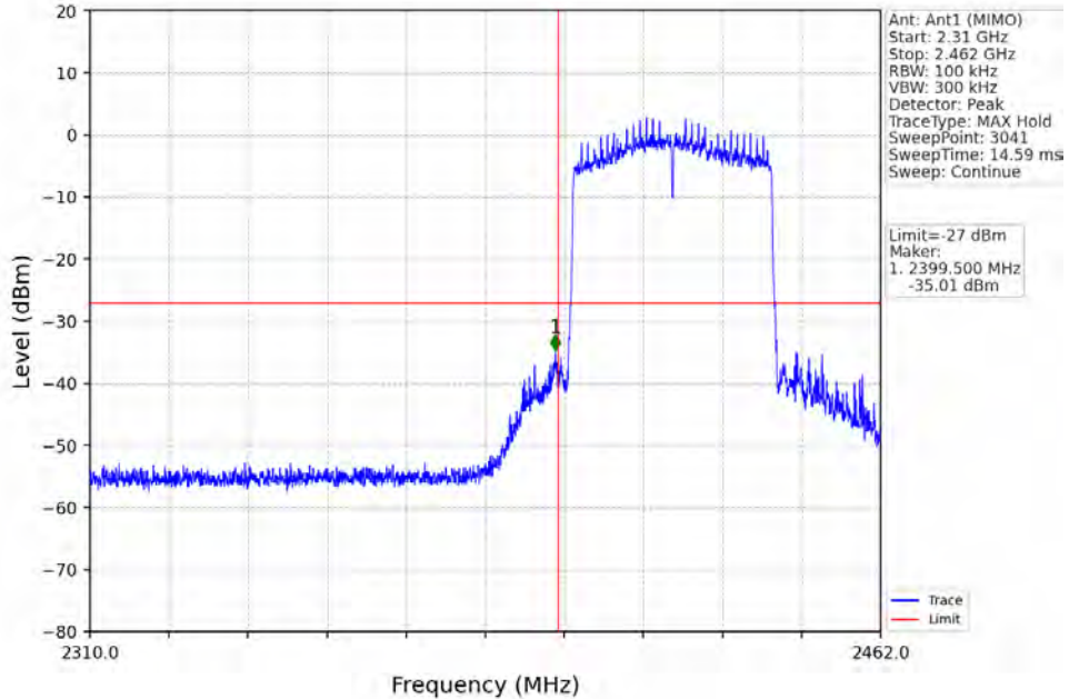
802.11ax(HEW40)_LCH_2422MHz_RU484_Left_Ant1 (MIMO)_NTNV
