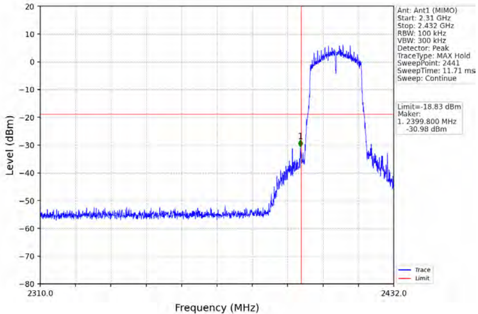
802.11n(HT20)_LCH_2412MHz_Ant1 (MIMO)_NTNV
