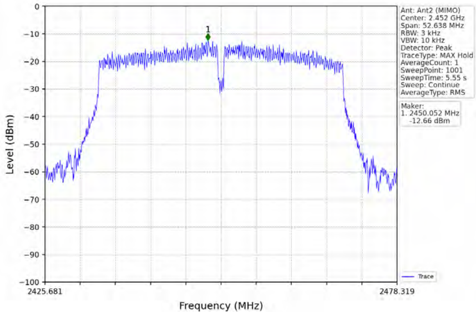
802.11n(HT40)_HCH_2452MHz_MIMO_NTNV
