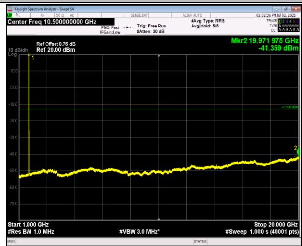
66-66-20MHz-20MHz-QPSK-QPSK-132072-132270-1RB#0 -1RB#99-1000~20000MHz-PASS
