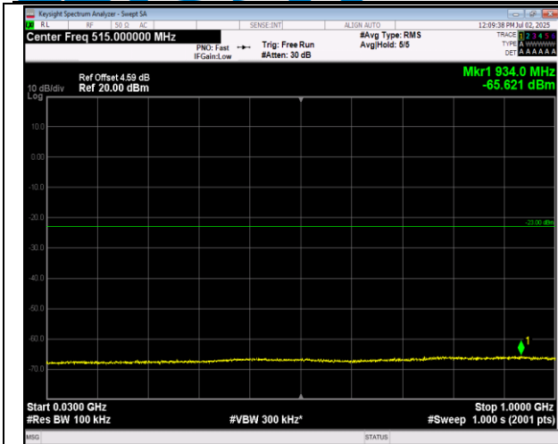
66-66-20MHz-5MHz-QPSK-QPSK-132072-132189-100R B#0-25RB#0-30~1000MHz-PASS
