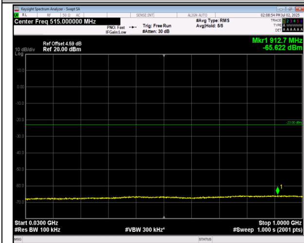
66-66-20MHz-20MHz-QPSK-QPSK-132323-132521-100 RB#0-100RB#0-30~1000MHz-PASS
