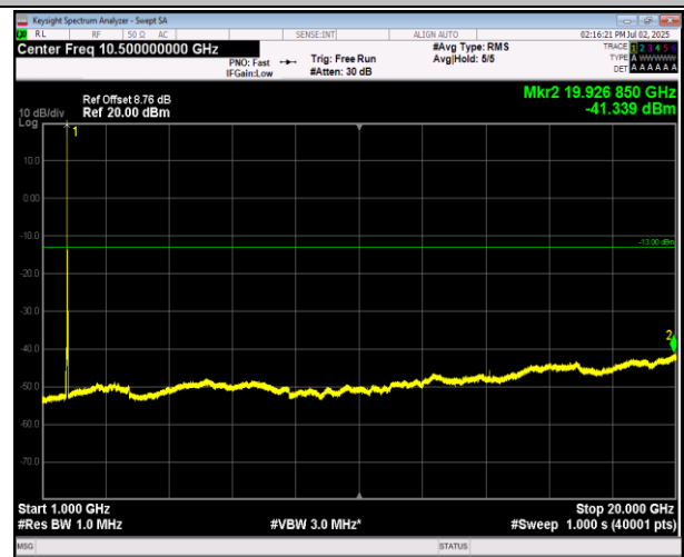
66-66-20MHz-20MHz-16QAM-16QAM-132374-132572-1R B#99-0RB#0-1000~20000MHz-PASS
