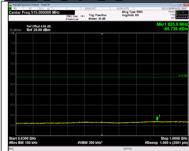
66-66-20MHz-20MHz-16QAM-16QAM-132323-132521-1 RB#0-ORB#0-30~1000MHz-PASS
