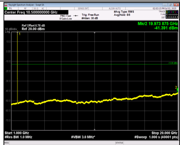
66-66-20MHz-20MHz-16QAM-16QAM-132072-132270-1RB#0-1RB#99-1000~20000MHz-PASS
