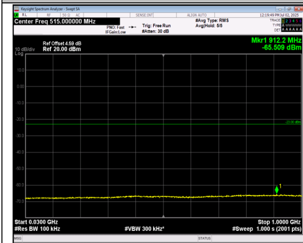
66-66-20MHz-5MHz-QPSK-QPSK-132522-132639-1RB# 0-ORB#0-30~1000MHz-PASS
