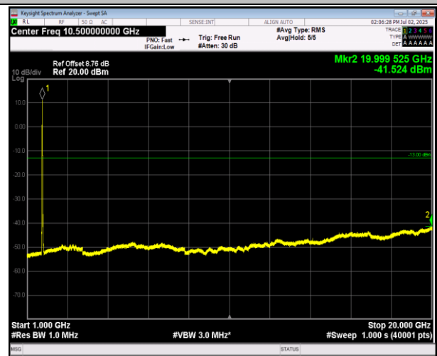
66-66-20MHz-20MHz-16QAM-16QAM-132072-132270-1RB#0-0RB#0-1000~20000MHz-PASS
