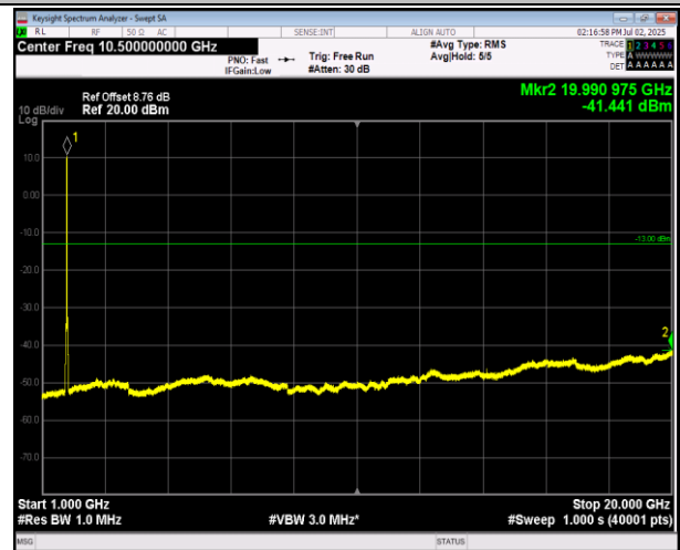
66-66-20MHz-20MHz-16QAM-16QAM-132374-132572-1R B#0-ORB#0-1000~20000MHz-PASS
