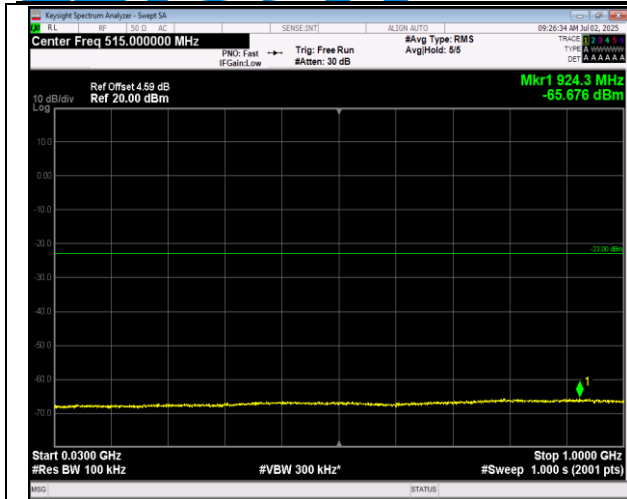
66-66-5MHz-20MHz-16QAM-16QAM-132455-132572-1R B#0-1RB#99-30~1000MHz-PASS
