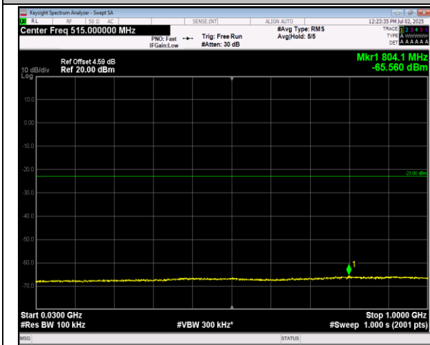
66-66-20MHz-5MHz-QPSK-QPSK-132522-132639-100RB# B#0-25RB#0-30~1000MHz-PASS
