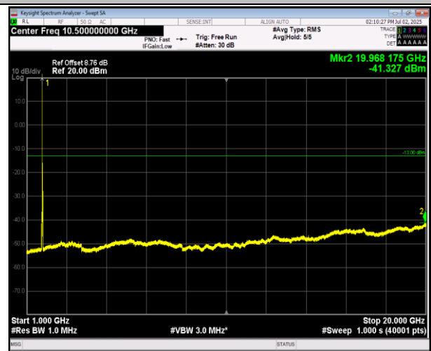
66-66-20MHz-20MHz-QPSK-QPSK-132323-132521-1RB#9 9-0RB#0-1000~20000MHz-PASS
