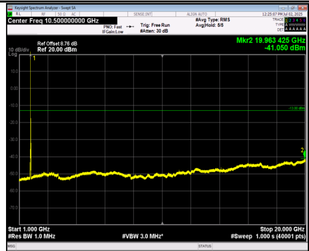
66-66-20MHz-5MHz-QPSK-QPSK-132522-132639-1RB#99 -ORB#0-1000~20000MHz-PASS
