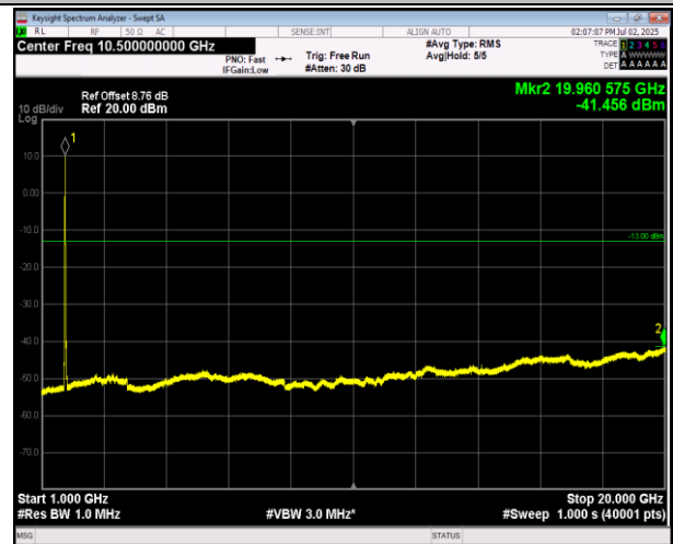
66-66-20MHz-20MHz-QPSK-QPSK-132323-132521-1RB#0 -ORB#0-1000~20000MHz-PASS
