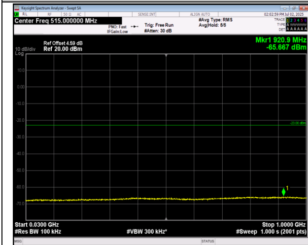
66-66-20MHz-20MHz-16QAM-16QAM-132072-132270-1RB#0-1RB#99-30~1000MHz-PASS
