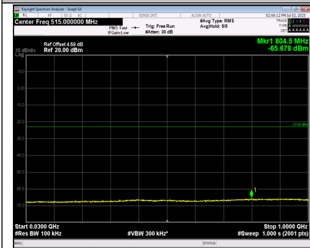
66-66-20MHz-20MHz-16QAM-16QAM-132072-132270-1RB#0-0RB#0-30~1000MHz-PASS
