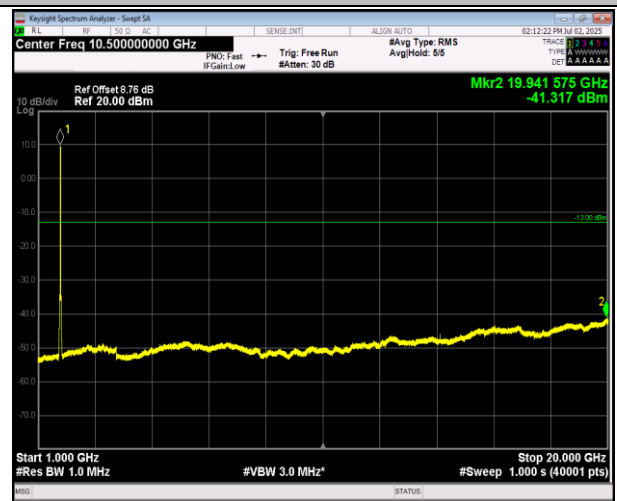
66-66-20MHz-20MHz-QPSK-QPSK-132374-132572-1RB#0-0RB#0-1000~20000MHz-PASS
