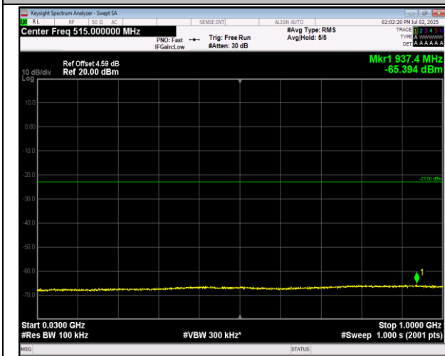
66-66-20MHz-20MHz-QPSK-QPSK-132072-132270-1RB #0-1RB#99-30~1000MHz-PASS
