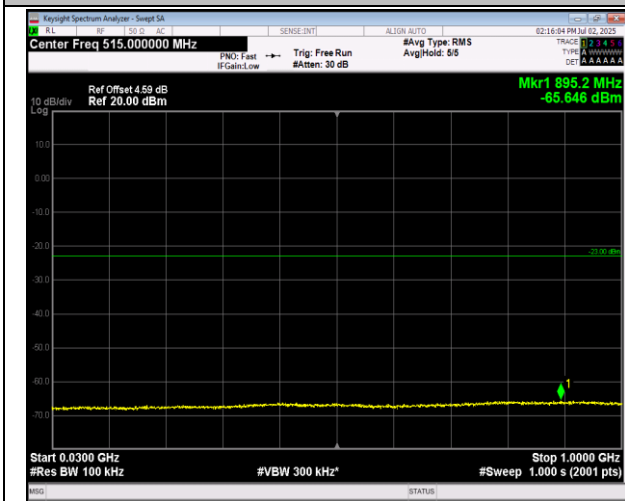
66-66-20MHz-20MHz-16QAM-16QAM-132374-132572-1 RB#99-0RB#0-30~1000MHz-PASS
