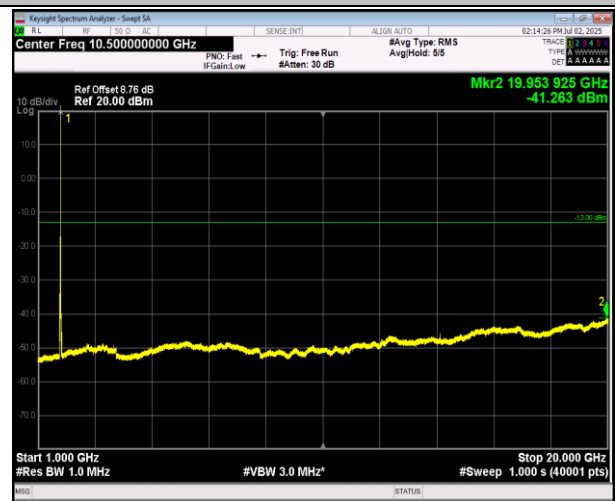
66-66-20MHz-20MHz-QPSK-QPSK-132374-132572-100RB #0-100RB#0-1000~20000MHz-PASS
