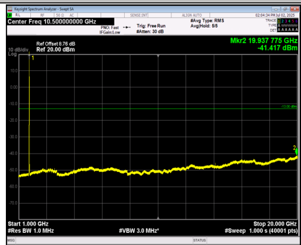
66-66-20MHz-20MHz-16QAM-16QAM-132072-132270-100 RB#0-100RB#0-1000~20000MHz-PASS
