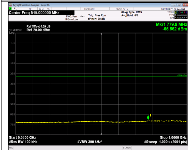
66-66-20MHz-20MHz-QPSK-QPSK-132072-132270-1RB #99-ORB#0-30~1000MHz-PASS
