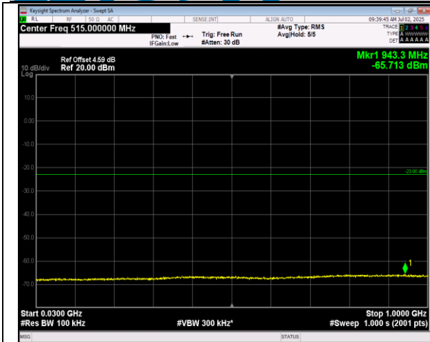
66-66-20MHz-5MHz-QPSK-QPSK-132072-132189-1RB# 0-0RB#0-30~1000MHz-PASS
