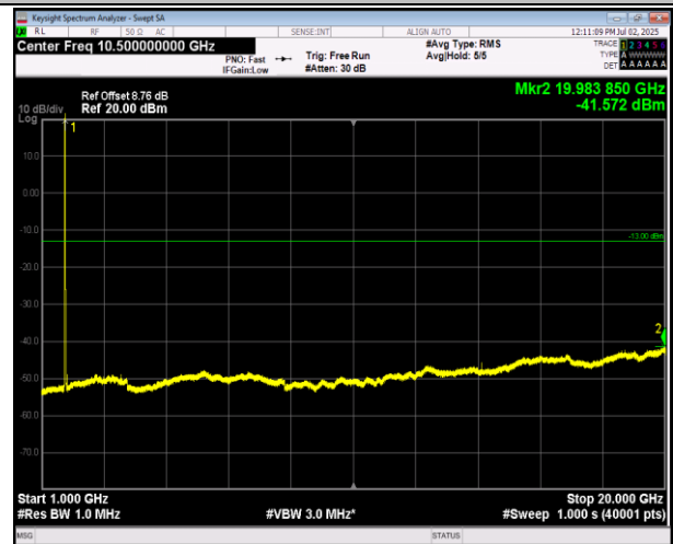
66-66-20MHz-5MHz-QPSK-QPSK-132072-132189-1RB#99 -0RB#0-1000~20000MHz-PASS
