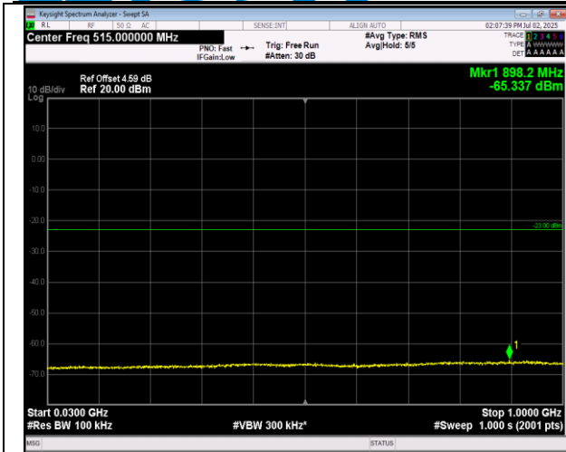
66-66-20MHz-20MHz-QPSK-QPSK-132323-132521-1RB #0-1RB#99-30~1000MHz-PASS
