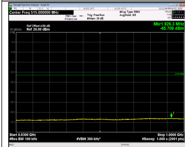
66-66-20MHz-5MHz-QPSK-QPSK-132397-132514-1RB# 0-ORB#0-30~1000MHz-PASS
