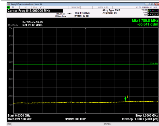
66-66-20MHz-20MHz-QPSK-QPSK-132323-132521-1RB #0-ORB#0-30~1000MHz-PASS
