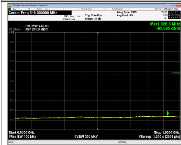
66-66-20MHz-20MHz-QPSK-QPSK-132323-132521-1RB #99-0RB#0-30~1000MHz-PASS
