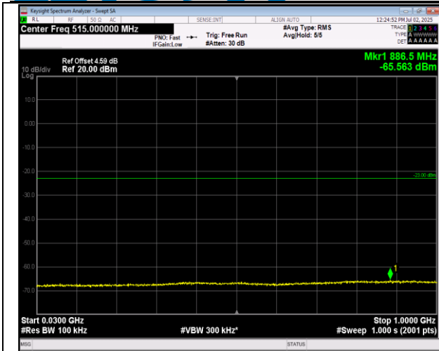
66-66-20MHz-5MHz-QPSK-QPSK-132522-132639-1RB# 99-ORB#0-30~1000MHz-PASS
