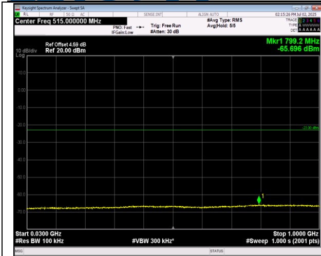
66-66-20MHz-20MHz-QPSK-QPSK-132374-132572-1RB #99-ORB#0-30~1000MHz-PASS
