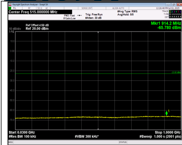
66-66-20MHz-20MHz-QPSK-QPSK-132072-132270-1RB #0-ORB#0-30~1000MHz-PASS
