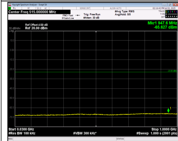
66-66-20MHz-20MHz-16QAM-16QAM-132374-132572-1 RB#0-ORB#0-30~1000MHz-PASS
