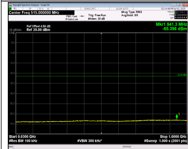
66-66-20MHz-20MHz-16QAM-16QAM-132374-132572-1 00RB#0-100RB#0-30~1000MHz-PASS
