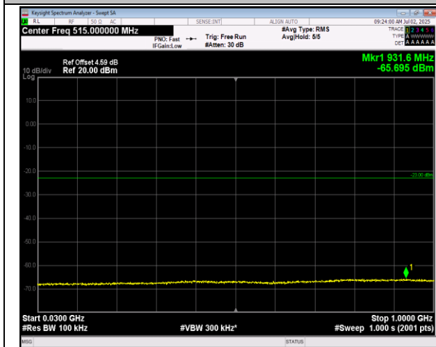
66-66-5MHz-20MHz-QPSK-QPSK-132455-132572-1RB# 0-1RB#99-30~1000MHz-PASS
