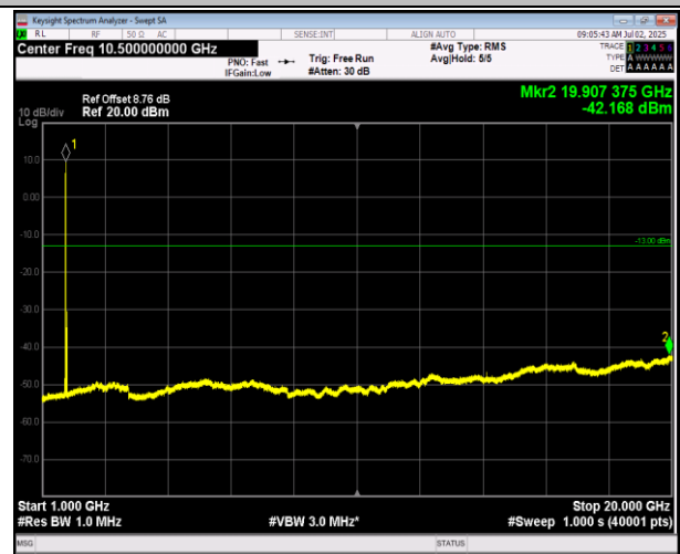
66-66-5MHz-20MHz-QPSK-QPSK-132005-132122-1RB#0- 1RB#99-1000~20000MHz-PASS
