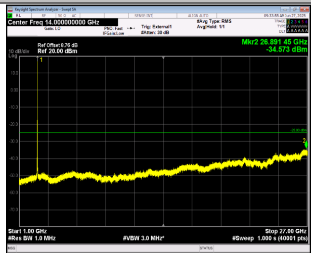
41(2555-2655)-41(2555-2655)-20MHz-5MHz-QPSK-QPSK- 41090-41207-100RB#0-25RB#0-1000~27000MHz-PASS
