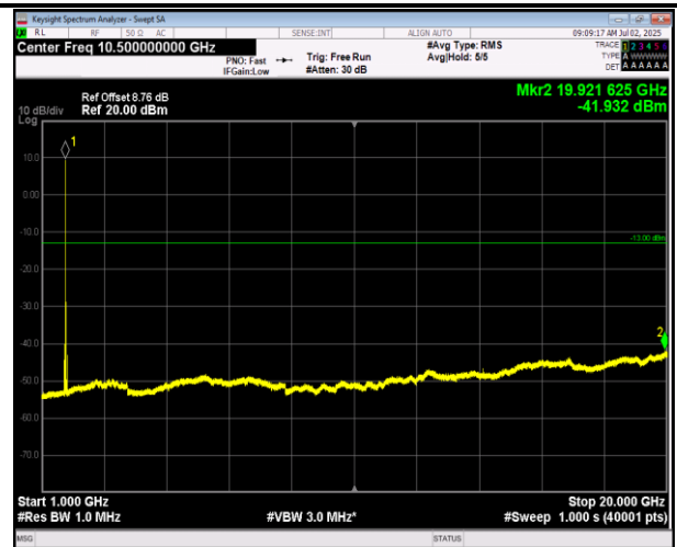
66-66-5MHz-20MHz-QPSK-QPSK-132005-132122-25RB#0 -100RB#0-1000~20000MHz-PASS
