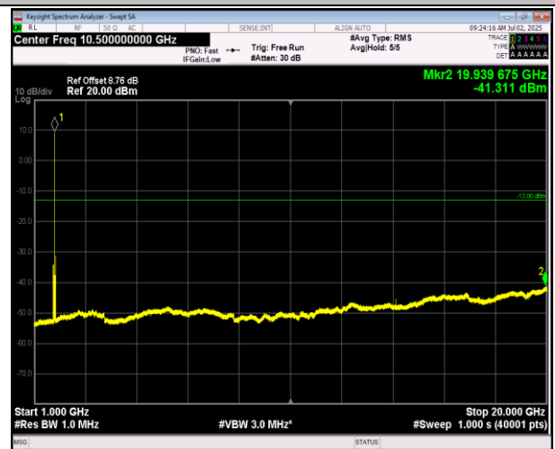
66-66-5MHz-20MHz-QPSK-QPSK-132455-132572-1RB#0- 1RB#99-1000~20000MHz-PASS
