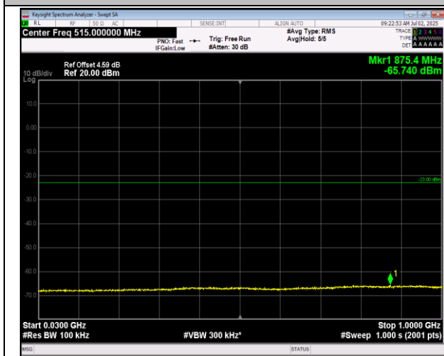
66-66-5MHz-20MHz-QPSK-QPSK-132455-132572-1RB# 0-0RB#0-30~1000MHz-PASS
