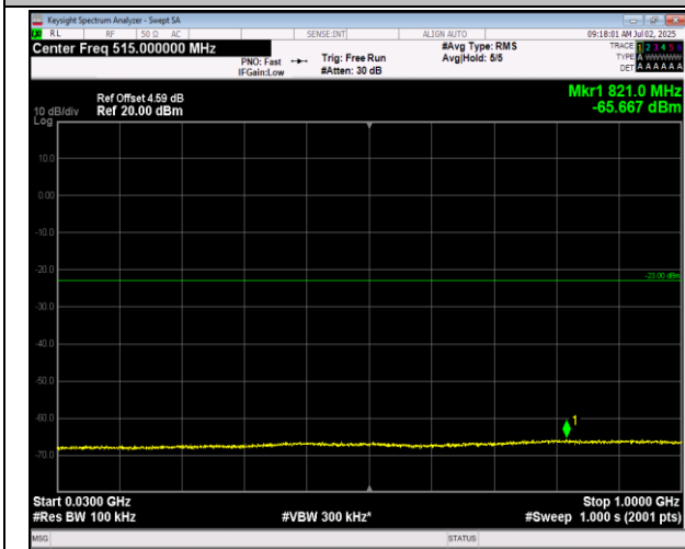
66-66-5MHz-20MHz-16QAM-16QAM-132330-132447-1R B#0-1RB#99-30~1000MHz-PASS
