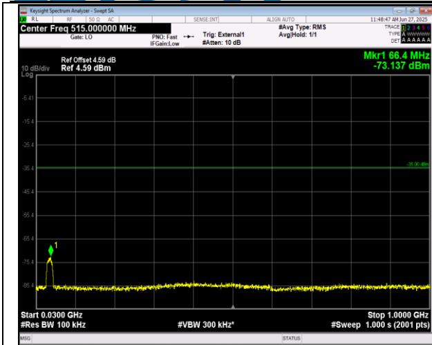
66-66-5MHz-20MHz-QPSK-QPSK-132005-132122-1RB# 0-0RB#0-30~1000MHz-PASS
