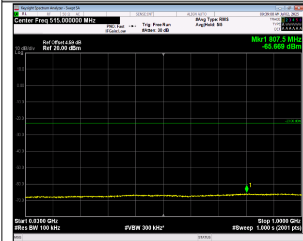
66-66-5MHz-20MHz-16QAM-16QAM-132455-132572-1R B#0-ORB#0-30~1000MHz-PASS
