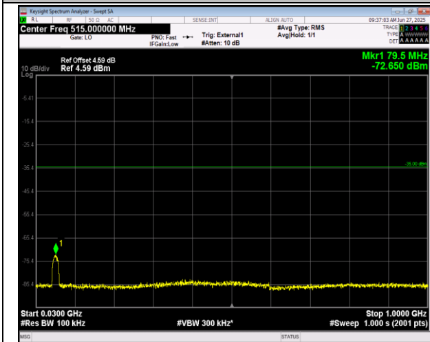
41(2555-2655)-41(2555-2655)-20MHz-5MHz-16QAM-16 QAM-41090-41207-1RB#0-0RB#0-30~1000MHz-PASS
