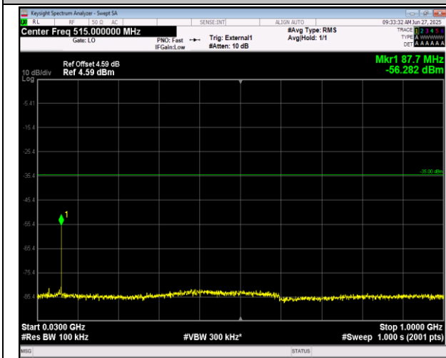
41(2555-2655)-41(2555-2655)-20MHz-5MHz-QPSK-QPSK K-41090-41207-100RB#0-25RB#0-30~1000MHz-PASS
