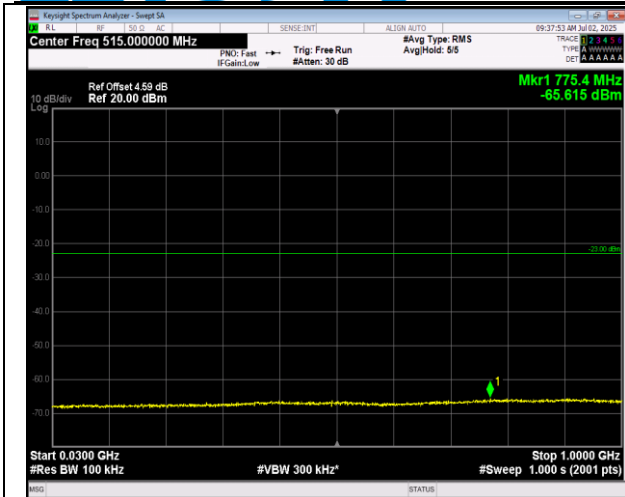
66-66-5MHz-20MHz-QPSK-QPSK-132455-132572-1RB# 24-ORB#0-30~1000MHz-PASS
