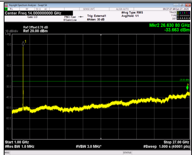
41(2555-2655)-41(2555-2655)-20MHz-5MHz-16QAM-16QA M-41090-41207-1RB#0-0RB#0-1000~27000MHz-PASS
