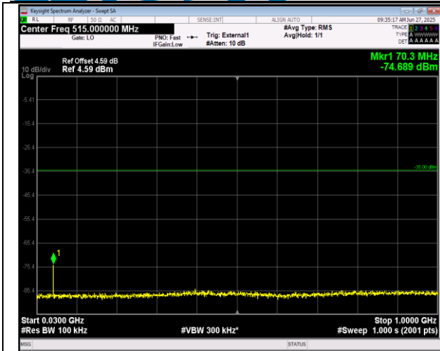
41(2555-2655)-41(2555-2655)-20MHz-5MHz-QPSK-QPSK K-41090-41207-1RB#99-0RB#0-30~1000MHz-PASS
