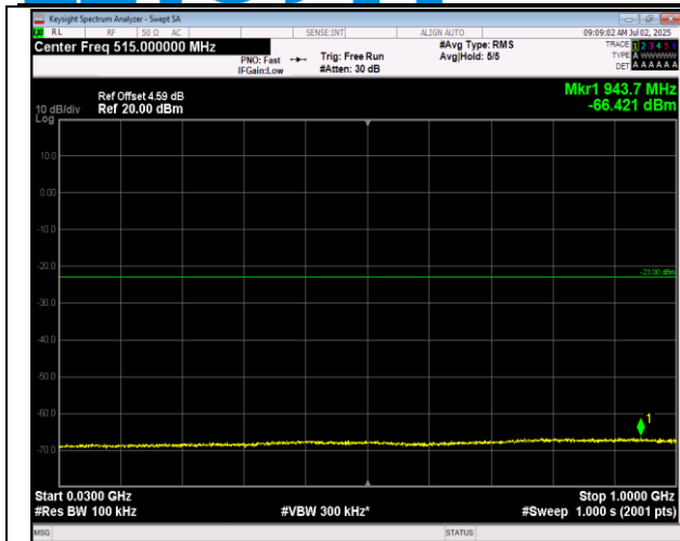
66-66-5MHz-20MHz-QPSK-QPSK-132005-132122-25RB #0-100RB#0-30~1000MHz-PASS
