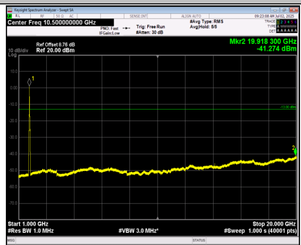
66-66-5MHz-20MHz-QPSK-QPSK-132455-132572-1RB#0- 0RB#0-1000~20000MHz-PASS
