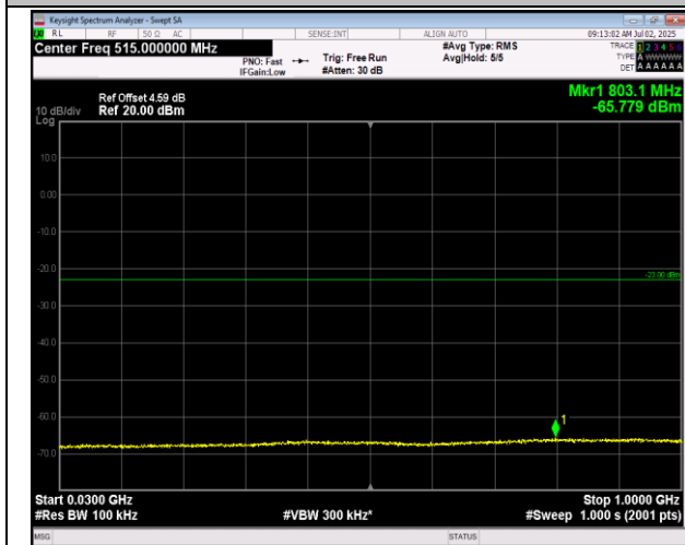
66-66-5MHz-20MHz-QPSK-QPSK-132330-132447-1RB# 0-ORB#0-30~1000MHz-PASS
