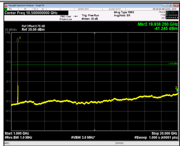
66-66-5MHz-20MHz-QPSK-QPSK-132455-132572-25RB#0 -100RB#0-1000~20000MHz-PASS
