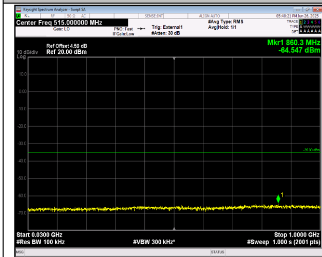
38-38-20MHz-20MHz-QPSK-QPSK-37952-38150-100RB #0-100RB#0-30~1000MHz-PASS
