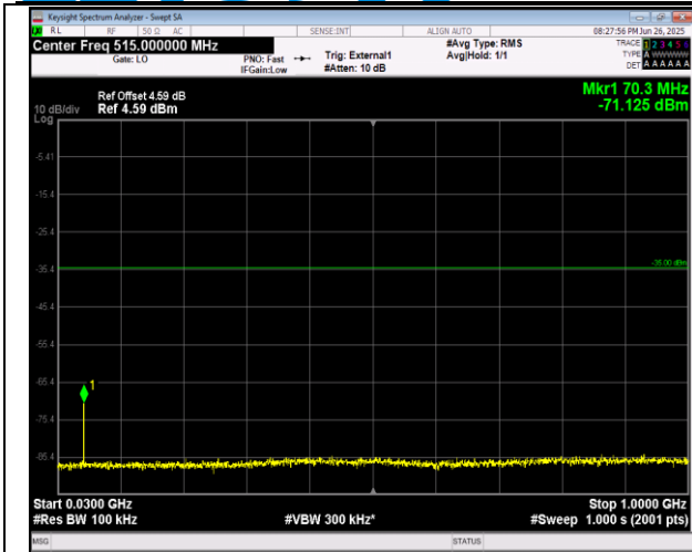
41(2555-2655)-41(2555-2655)-5MHz-20MHz-QPSK-QPS K-41023-41140-1RB#24-ORB#0-30~1000MHz-PASS
