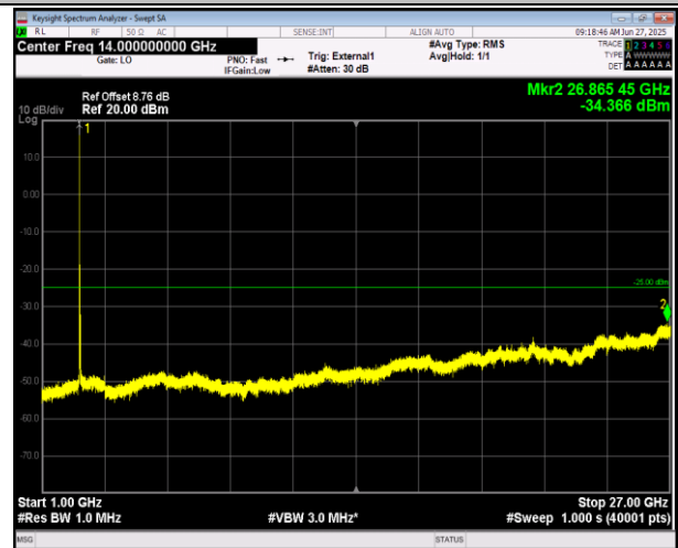
41(2555-2655)-41(2555-2655)-20MHz-5MHz-16QAM-16QA M-40340-40457-1RB#0-1RB#24-1000~27000MHz-PASS
