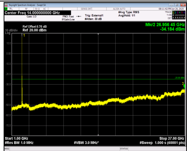
41(2555-2655)-41(2555-2655)-5MHz-20MHz-16QAM-16QA M-40273-40390-1RB#0-1RB#99-1000~27000MHz-PASS
