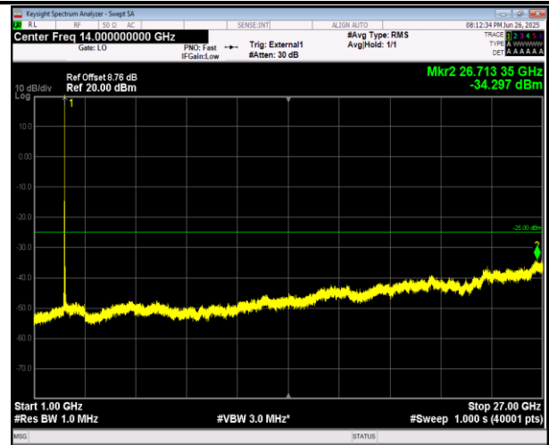
41(2555-2655)-41(2555-2655)-5MHz-20MHz-QPSK-QPSK- 40273-40390-25RB#0-100RB#0-1000~27000MHz-PASS
