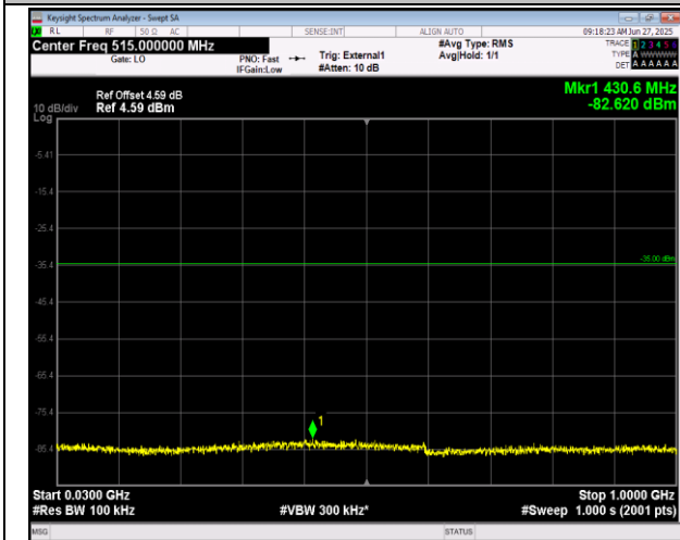
41(2555-2655)-41(2555-2655)-20MHz-5MHz-16QAM-16 QAM-40340-40457-1RB#0-1RB#24-30~1000MHz-PASS
