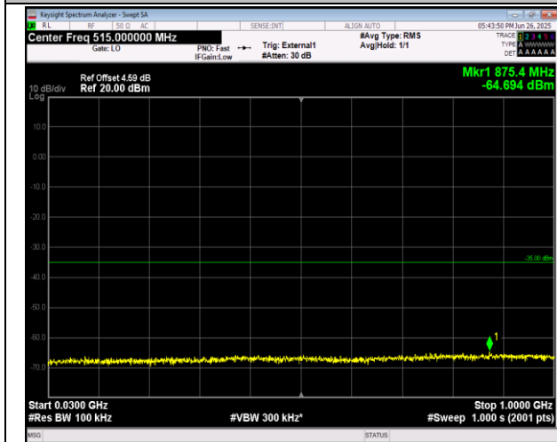
38-38-20MHz-20MHz-16QAM-16QAM-37952-38150-1RB #0-0RB#0-30~1000MHz-PASS
