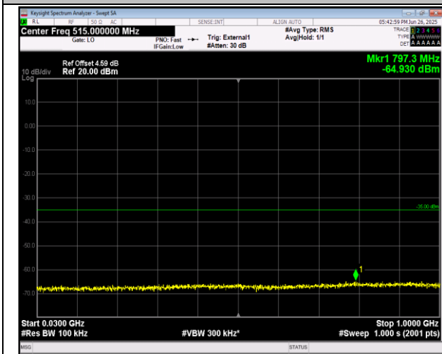
38-38-20MHz-20MHz-16QAM-16QAM-37952-38150-1RB #99-0RB#0-30~1000MHz-PASS
