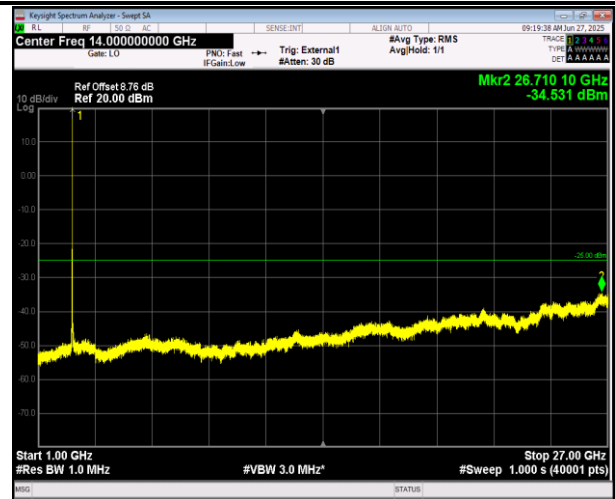
41(2555-2655)-41(2555-2655)-20MHz-5MHz-QPSK-QPSK- 40340-40457-100RB#0-25RB#0-1000~27000MHz-PASS
