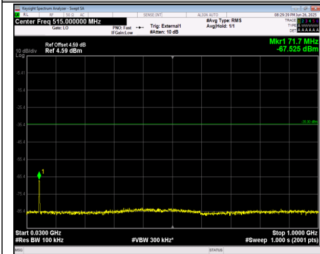
41(2555-2655)-41(2555-2655)-5MHz-20MHz-16QAM-16 QAM-41023-41140-1RB#0-ORB#0-30~1000MHz-PASS
