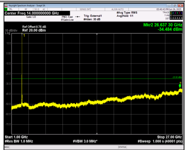
38-38-20MHz-20MHz-QPSK-QPSK-37952-38150-100RB#0 -100RB#0-1000~27000MHz-PASS
