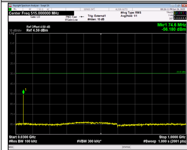
41(2555-2655)-41(2555-2655)-5MHz-20MHz-QPSK-QPS K-41023-41140-25RB#0-100RB#0-30~1000MHz-PASS
