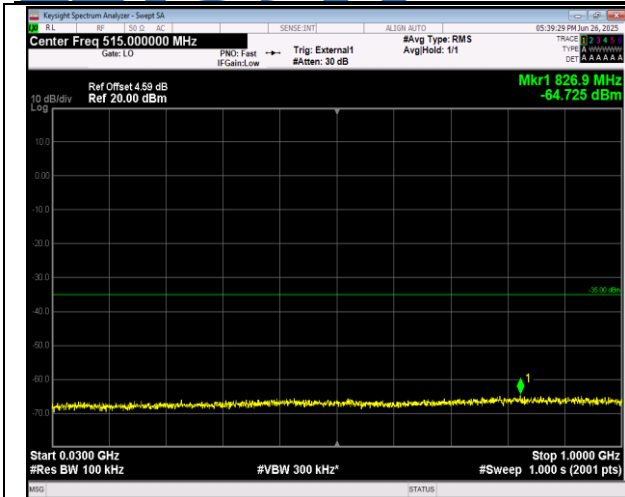
38-38-20MHz-20MHz-16QAM-16QAM-37952-38150-1RB #0-1RB#99-30~1000MHz-PASS
