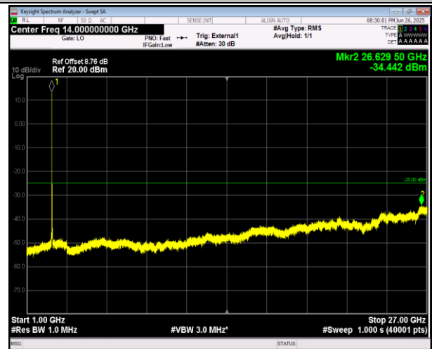
41(2555-2655)-41(2555-2655)-5MHz-20MHz-16QAM-16QA M-41023-41140-1RB#0-ORB#0-1000~27000MHz-PASS
