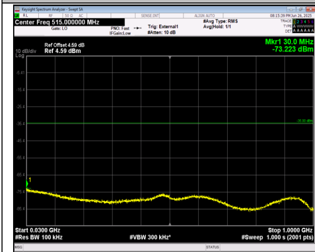
41(2555-2655)-41(2555-2655)-5MHz-20MHz-16QAM-16 QAM-40273-40390-1RB#0-0RB#0-30~1000MHz-PASS
