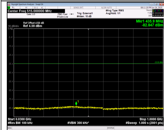
41(2555-2655)-41(2555-2655)-5MHz-20MHz-16QAM-16 QAM-40273-40390-1RB#0-1RB#99-30~1000MHz-PASS
