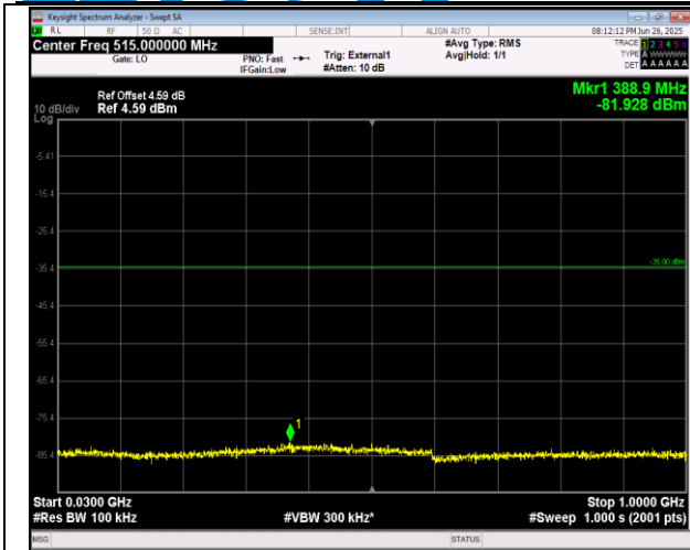
41(2555-2655)-41(2555-2655)-5MHz-20MHz-QPSK-QPS K-40273-40390-25RB#0-100RB#0-30~1000MHz-PASS
