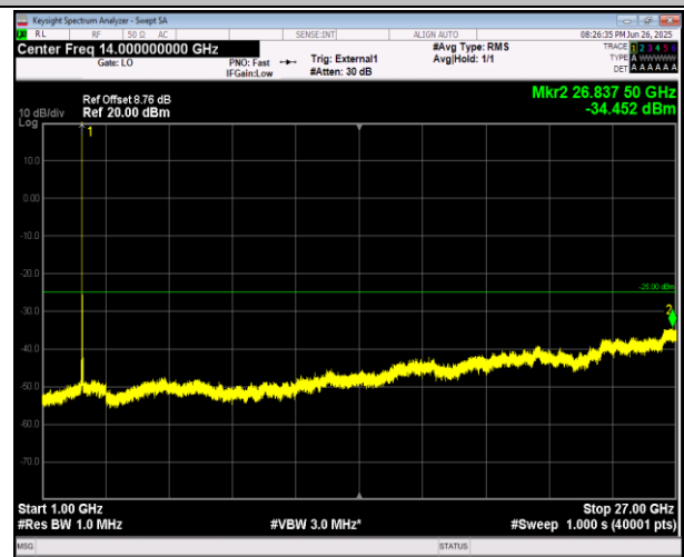
41(2555-2655)-41(2555-2655)-5MHz-20MHz-QPSK-QPSK- 41023-41140-25RB#0-100RB#0-1000~27000MHz-PASS
