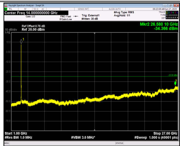
41(2555-2655)-41(2555-2655)-20MHz-5MHz-16QAM-16QA M-40340-40457-1RB#0-0RB#0-1000~27000MHz-PASS
