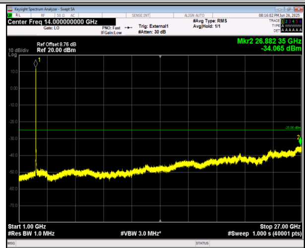
41(2555-2655)-41(2555-2655)-5MHz-20MHz-16QAM-16QA M-40273-40390-1RB#0-0RB#0-1000~27000MHz-PASS
