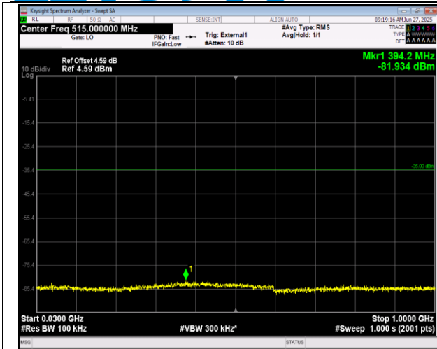
41(2555-2655)-41(2555-2655)-20MHz-5MHz-QPSK-QPS K-40340-40457-100RB#0-25RB#0-30~1000MHz-PASS
