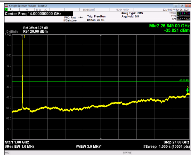
7-7-20MHz-20MHz-QPSK-QPSK-21152-21350-1RB#0-1RB #99-1000~27000MHz-PASS
