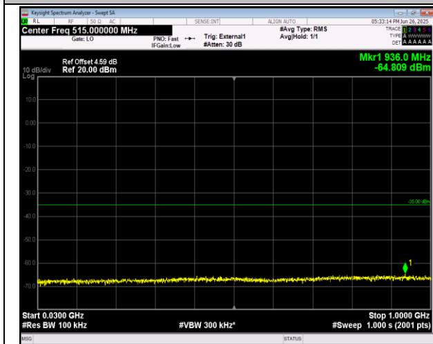
38-38-20MHz-20MHz-QPSK-QPSK-37901-38099-100RB#0-100RB#0-30~1000MHz-PASS
