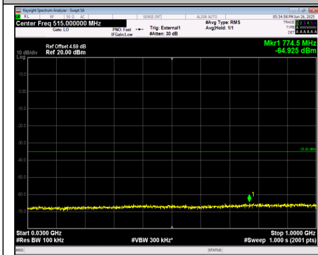
38-38-20MHz-20MHz-QPSK-QPSK-37901-38099-1RB#99-9-0RB#0-30~1000MHz-PASS
