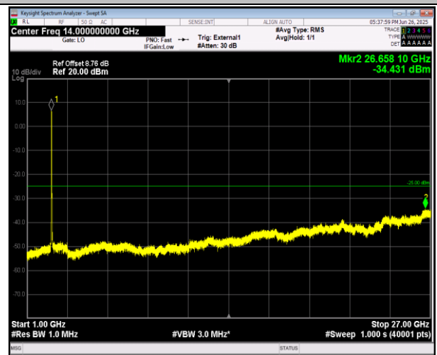
38-38-20MHz-20MHz-QPSK-QPSK-37952-38150-1RB#0-0 RB#0-1000~27000MHz-PASS
