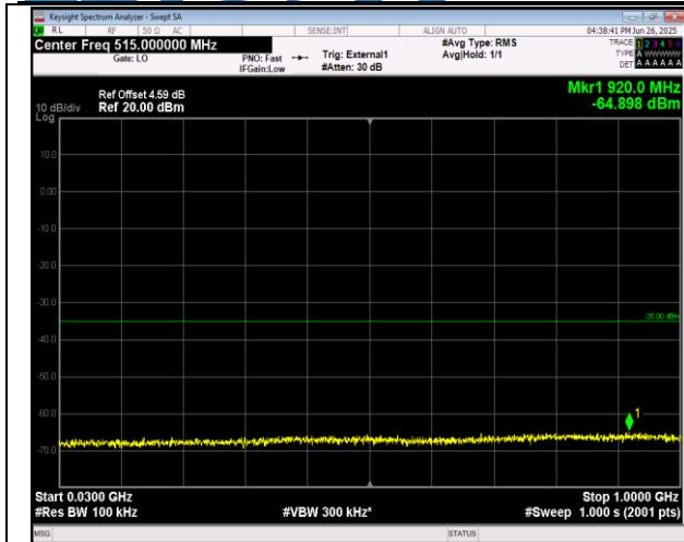
38-38-20MHz-20MHz-QPSK-QPSK-37850-38048-1RB#0-ORB#0-30~1000MHz-PASS
