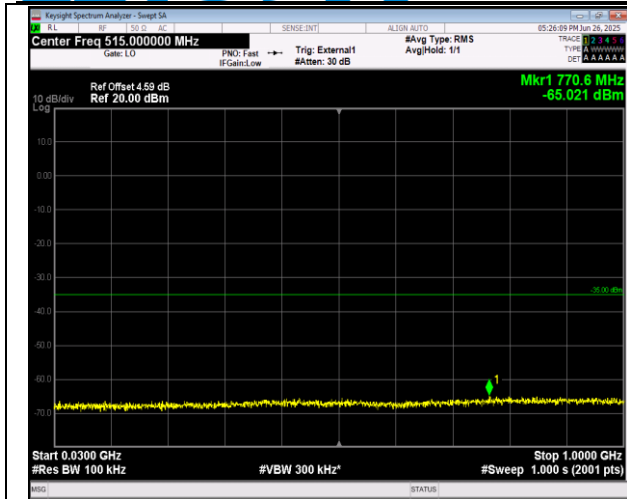
38-38-20MHz-20MHz-QPSK-QPSK-37850-38048-100RB #0-100RB#0-30~1000MHz-PASS
