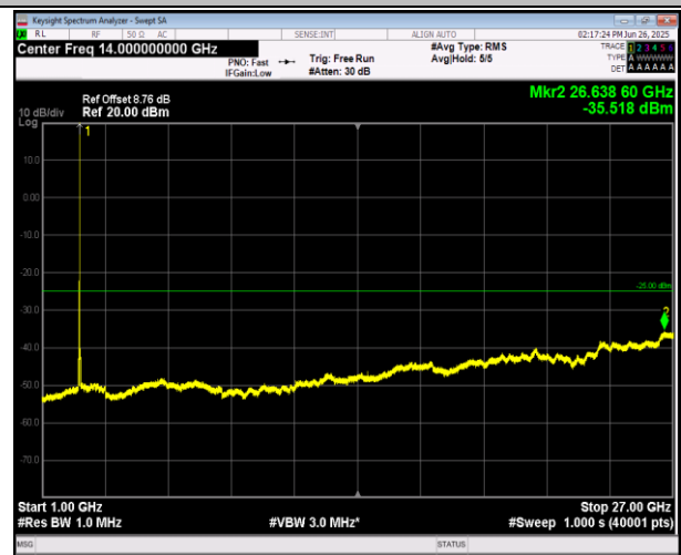
7-7-20MHz-20MHz-QPSK-QPSK-21152-21350-100RB#0-1 00RB#0-1000~27000MHz-PASS
