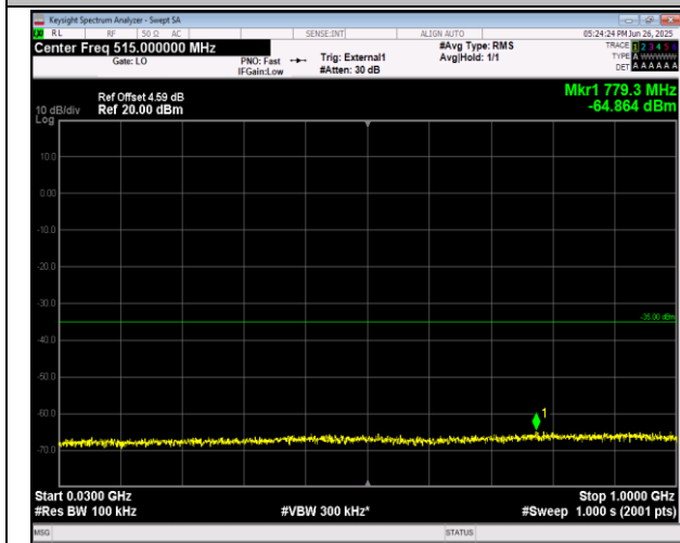
38-38-20MHz-20MHz-QPSK-QPSK-37850-38048-1RB#0-1RB#99-30~1000MHz-PASS
