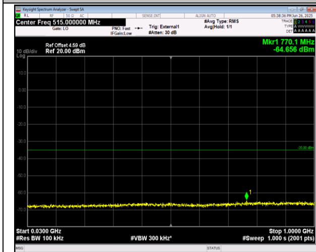
38-38-20MHz-20MHz-QPSK-QPSK-37952-38150-1RB#0- 1RB#99-30~1000MHz-PASS
