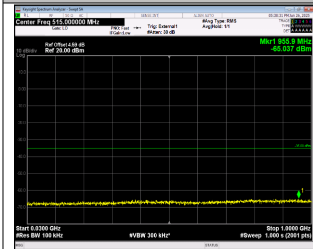
38-38-20MHz-20MHz-QPSK-QPSK-37901-38099-1RB#0- ORB#0-30~1000MHz-PASS
