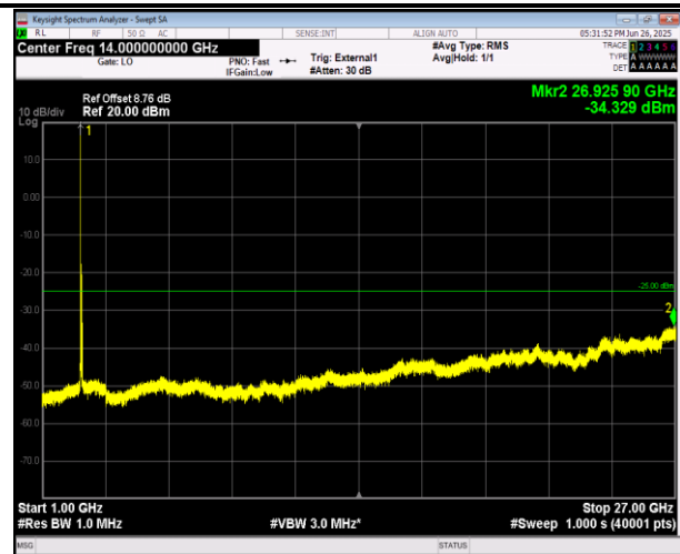
38-38-20MHz-20MHz-QPSK-QPSK-37901-38099-1RB#0-1RB#99-1000~27000MHz-PASS
