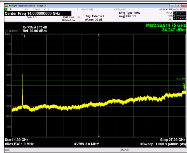
38-38-20MHz-20MHz-QPSK-QPSK-37850-38048-1RB#0-1RB#99-1000~27000MHz-PASS
