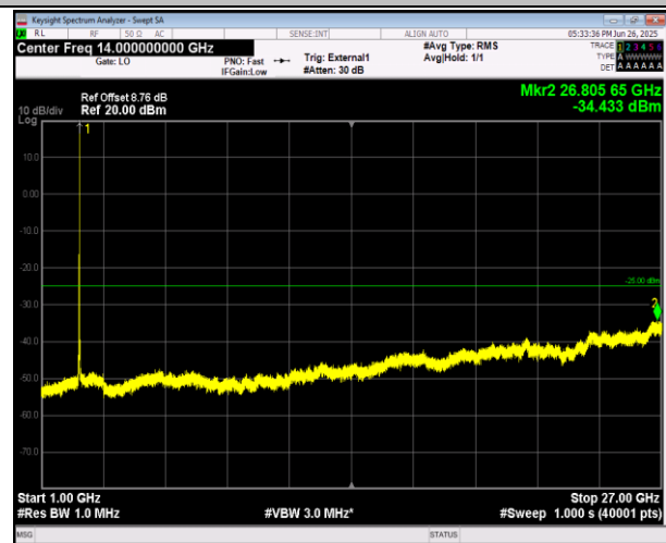
38-38-20MHz-20MHz-QPSK-QPSK-37901-38099-100RB#0-100RB#0-1000~27000MHz-PASS
