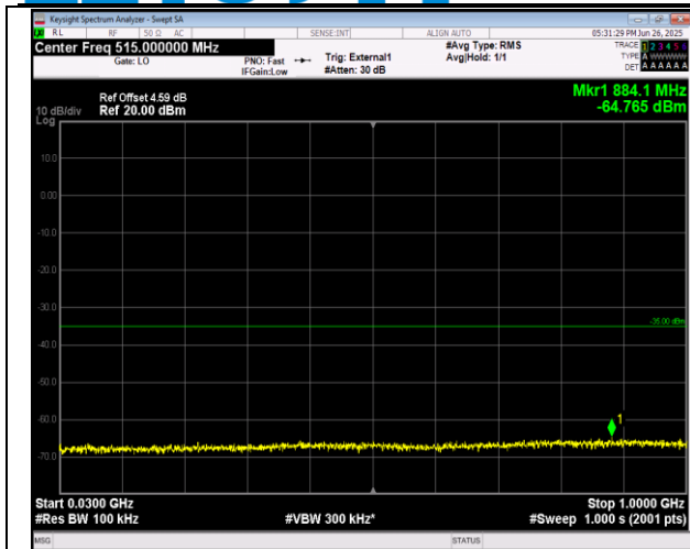
38-38-20MHz-20MHz-QPSK-QPSK-37901-38099-1RB#0-1RB#99-30~1000MHz-PASS
