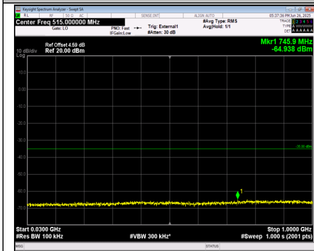
38-38-20MHz-20MHz-QPSK-QPSK-37952-38150-1RB#0- ORB#0-30~1000MHz-PASS
