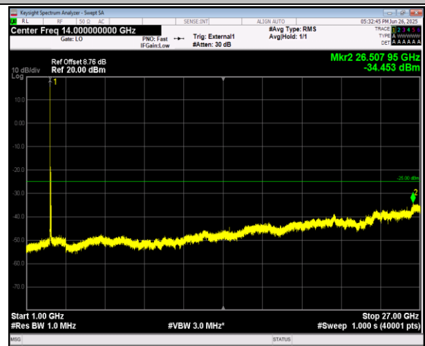
38-38-20MHz-20MHz-16QAM-16QAM-37901-38099-1RB# 0-1RB#99-1000~27000MHz-PASS
