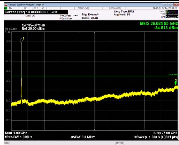
38-38-20MHz-20MHz-QPSK-QPSK-37850-38048-1RB#0-0RB#0-1000~27000MHz-PASS
