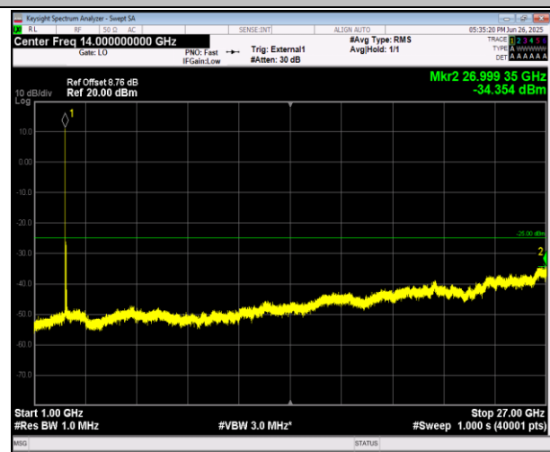
38-38-20MHz-20MHz-QPSK-QPSK-37901-38099-1RB#99-9-0RB#0-1000~27000MHz-PASS
