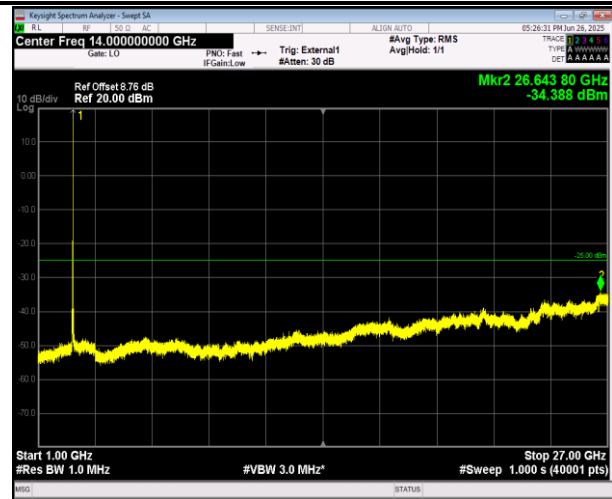
38-38-20MHz-20MHz-QPSK-QPSK-37850-38048-100RB#0 -100RB#0-1000~27000MHz-PASS
