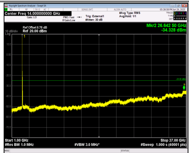
38-38-20MHz-20MHz-QPSK-QPSK-37952-38150-1RB#0-1 RB#99-1000~27000MHz-PASS
