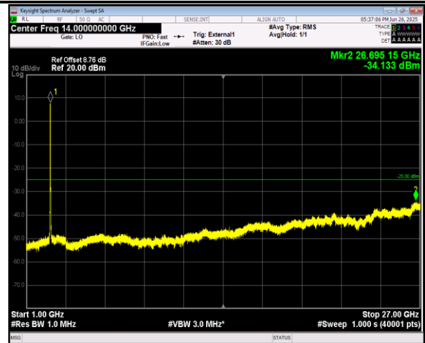
38-38-20MHz-20MHz-16QAM-16QAM-37901-38099-1RB# 0-ORB#0-1000~27000MHz-PASS
