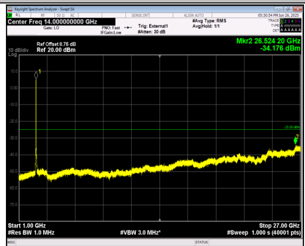
38-38-20MHz-20MHz-QPSK-QPSK-37901-38099-1RB#0-0 RB#0-1000~27000MHz-PASS
