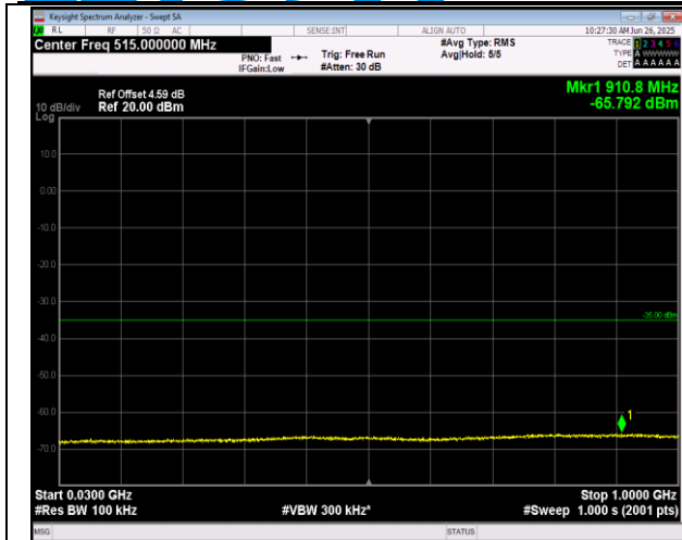
7-7-20MHz-10MHz-QPSK-QPSK-20850-20994-100RB#0-50RB#0-30~1000MHz-PASS
