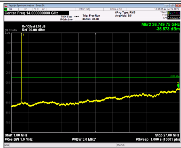
7-7-20MHz-10MHz-QPSK-QPSK-21251-21395-100RB#0-50RB#0-30~1000MHz-PASS ORB#0-1000~27000MHz-PASS
