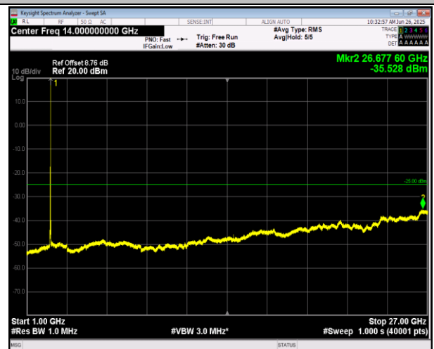
7-7-20MHz-10MHz-QPSK-QPSK-21051-21195-100RB#0-5 ORB#0-1000~27000MHz-PASS
