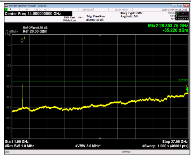
7-7-20MHz-10MHz-QPSK-QPSK-21051-21195-1RB#99-0R B#0-1000~27000MHz-PASS
