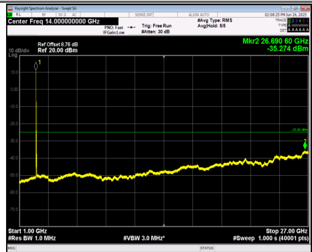
7-7-20MHz-20MHz-QPSK-QPSK-20850-21048-1RB#99-0R B#0-1000~27000MHz-PASS
