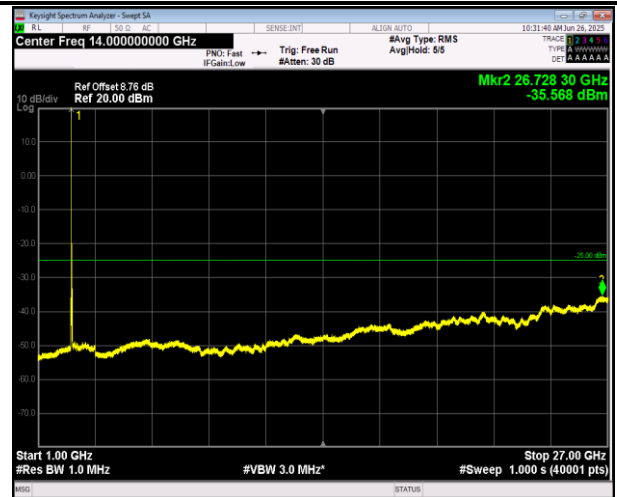
7-7-20MHz-10MHz-QPSK-QPSK-21051-21195-1RB#0-1RB #49-1000~27000MHz-PASS
