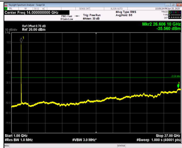
7-7-10MHz-20MHz-QPSK-QPSK-20805-20949-1RB#49-0R B#0-1000~27000MHz-PASS
