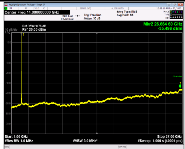
7-7-10MHz-20MHz-QPSK-QPSK-20805-20949-50RB#0-10 0RB#0-1000~27000MHz-PASS
