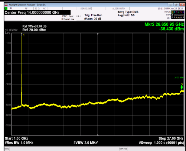
7-7-10MHz-20MHz-QPSK-QPSK-21006-21150-1RB#0-1RB #99-1000~27000MHz-PASS
