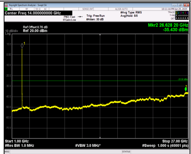
7-7-10MHz-20MHz-QPSK-QPSK-21006-21150-1RB#0-0RB #0-1000~27000MHz-PASS
