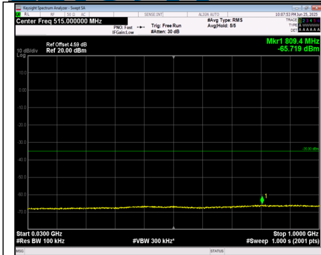
7-7-10MHz-20MHz-QPSK-QPSK-20805-20949-50RB#0-1 00RB#0-30~1000MHz-PASS
