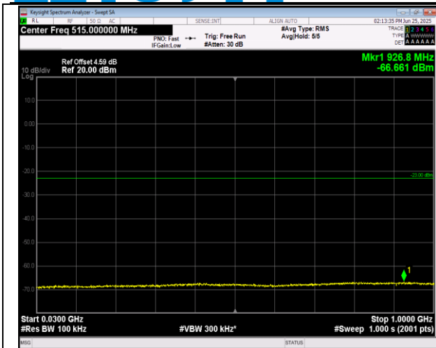
2-2-20MHz-20MHz-16QAM-16QAM-18801-18999-1RB#0 -0RB#0-30~1000MHz-PASS
