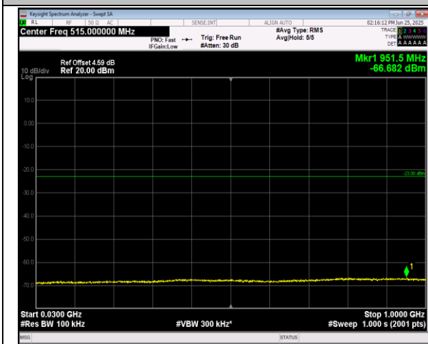
2-2-20MHz-20MHz-QPSK-QPSK-18902-19100-100RB#0- 100RB#0-30~1000MHz-PASS
