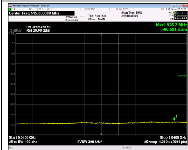
2-2-20MHz-20MHz-16QAM-16QAM-18801-18999-1RB#9 9-0RB#0-30~1000MHz-PASS
