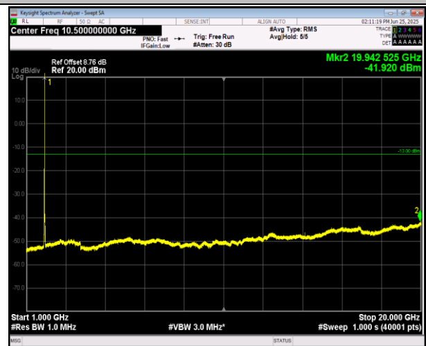
2-2-20MHz-20MHz-QPSK-QPSK-18801-18999-100RB#0-1 00RB#0-1000~20000MHz-PASS
