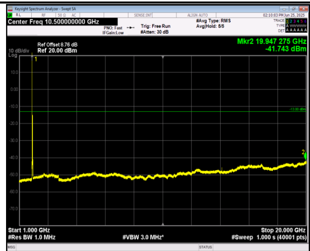
2-2-20MHz-20MHz-QPSK-QPSK-18801-18999-1RB#0-1RB #99-1000~20000MHz-PASS
