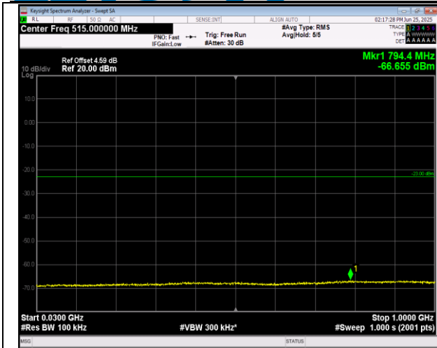
2-2-20MHz-20MHz-QPSK-QPSK-18902-19100-1RB#99-0 RB#0-30~1000MHz-PASS
