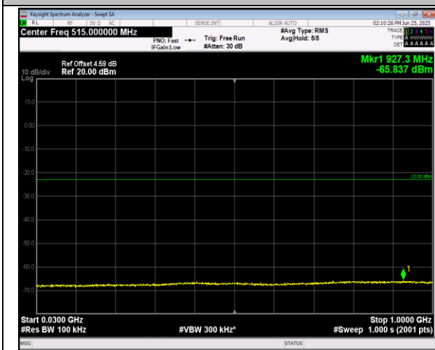
2-2-20MHz-20MHz-16QAM-16QAM-18801-18999-1RB#0 -1RB#99-30~1000MHz-PASS
