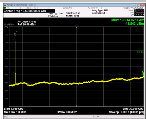
2-2-20MHz-20MHz-16QAM-16QAM-18700-18898-1RB#0-0RB#0-0-1000~20000MHz-PASS
