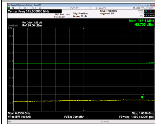
2-2-20MHz-20MHz-16QAM-16QAM-18700-18898-1RB#0-0RB#0-0-30~1000MHz-PASS
