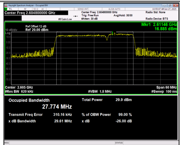
41(2555-2655)-41(2555-2655)-20MHz-10MHz-16QAM-16Q AM-41041-41185-100RB#0-50RB#0-PASS
