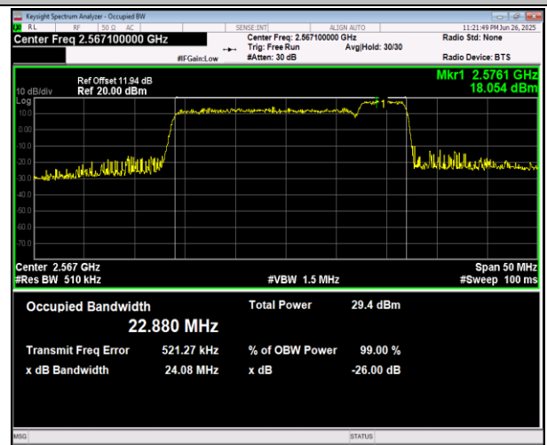
41(2555-2655)-41(2555-2655)-20MHz-5MHz-16QAM-16QA M-40715-40832-100RB#0-25RB#0-PASS
