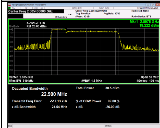
41(2555-2655)-41(2555-2655)-5MHz-20MHz-QPSK-QPS K-41023-41140-25RB#0-100RB#0-PASS
