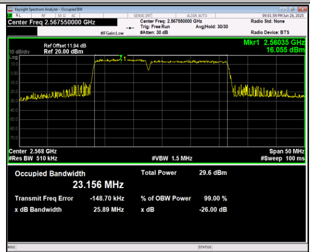
41(2555-2655)-41(2555-2655)-10MHz-15MHz-16QAM-16Q AM-40669-40789-50RB#0-75RB#0-PASS
