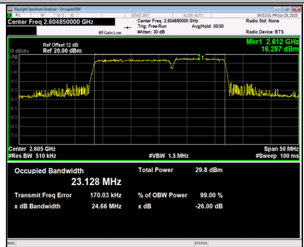
41(2555-2655)-41(2555-2655)-15MHz-10MHz-16QAM-16Q AM-41067-41187-75RB#0-50RB#0-PASS
