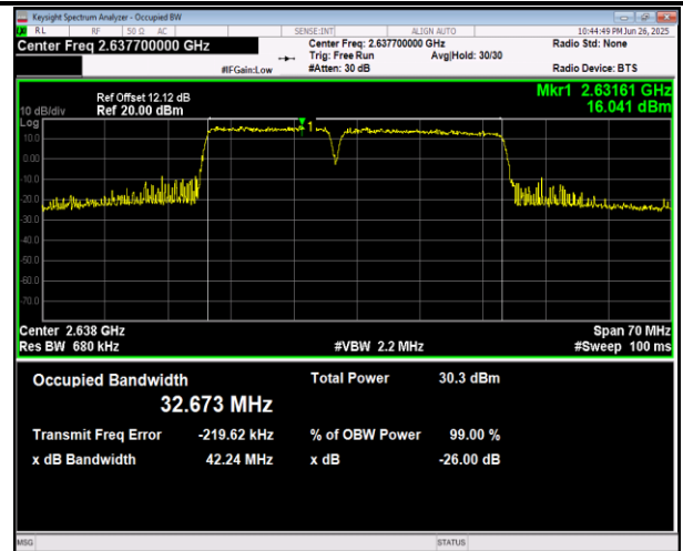
41(2555-2655)-41(2555-2655)-20MHz-5MHz-16QAM-16QA M-40340-40457-100RB#0-25RB#0-PASS
