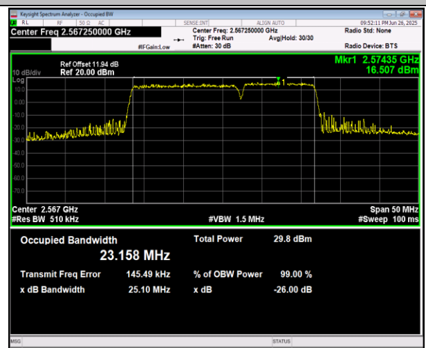
41(2555-2655)-41(2555-2655)-15MHz-10MHz-16QAM-16Q AM-40691-40811-75RB#0-50RB#0-PASS
