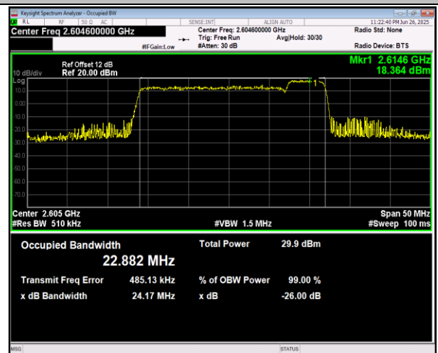
41(2555-2655)-41(2555-2655)-20MHz-5MHz-16QAM-16QA M-41090-41207-100RB#0-25RB#0-PASS
