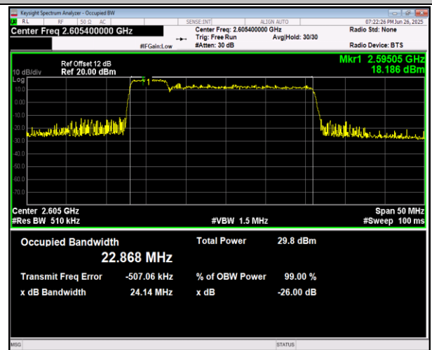
41(2555-2655)-41(2555-2655)-5MHz-20MHz-16QAM-16QA M-41023-41140-25RB#0-100RB#0-PASS
