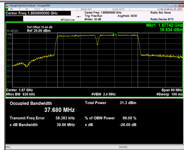
2-2-20MHz-20MHz-QPSK-QPSK-18801-18999-100RB#0-100RB#0-PASS
