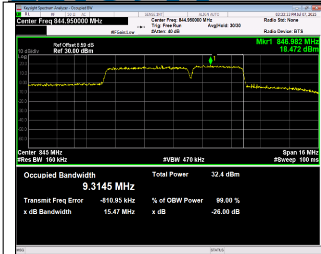
5-5-5MHz-10MHz-QPSK-QPSK-20428-20500-25RB#0-50 RB#0-PASS
