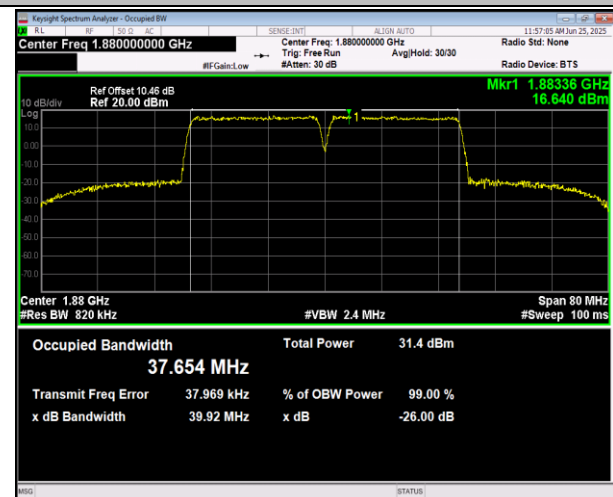
2-2-20MHz-20MHz-QPSK-QPSK-18902-19100-100RB#0-100RB#0-PASS
