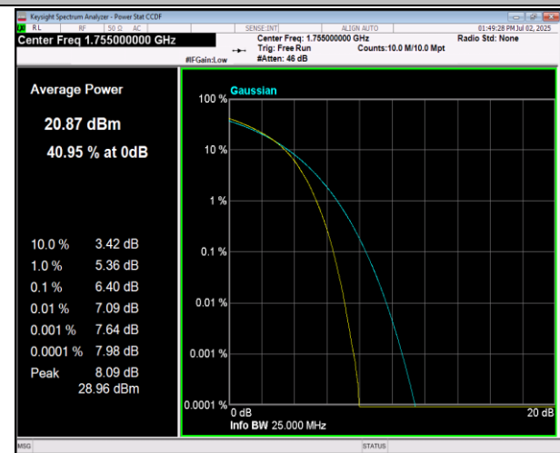
66-66-20MHz-20MHz-16QAM-16QAM-132323-132521-10 ORB#0-100RB#0-PASS
