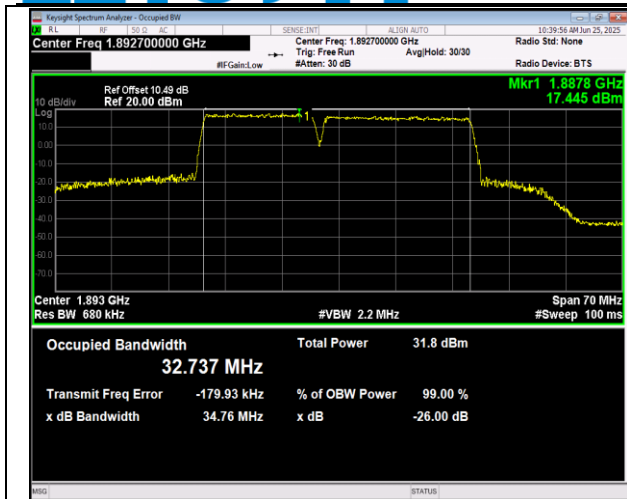
2-2-20MHz-5MHz-QPSK-QPSK-18700-18817-100RB#0-2 5RB#0-PASS
