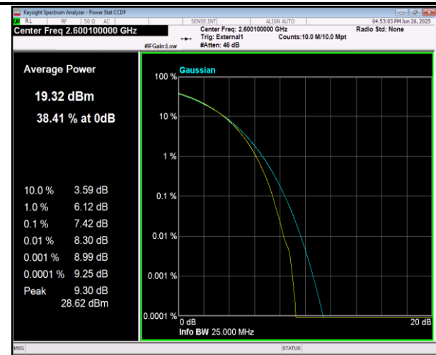
41(2555-2655)-41(2555-2655)-20MHz-20MHz-16QAM-16 QAM-40641-40839-100RB#0-100RB#0-PASS
