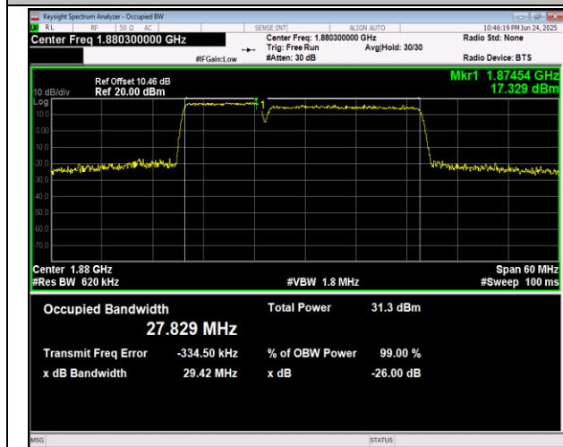
2-2-10MHz-20MHz-QPSK-QPSK-18956-19100-50RB#0-1 00RB#0-PASS
