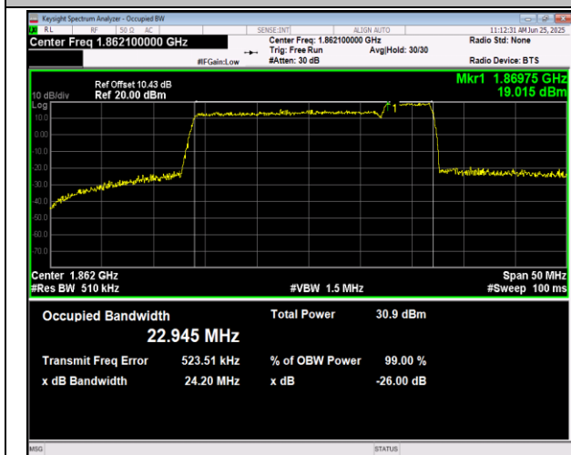
2-2-20MHz-5MHz-QPSK-QPSK-18875-18992-100RB#0-2 5RB#0-PASS
