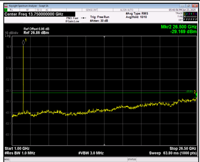
Band38-5MHz-QPSK-38225-1RB#0-Range2:1000~2 6500MHz
