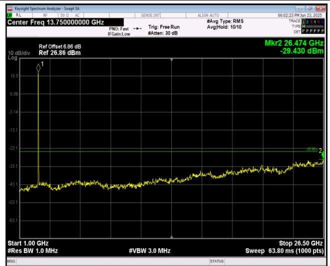
Band38-20MHz-QPSK-38150-1RB#0-Range2:1000~26500MHz
