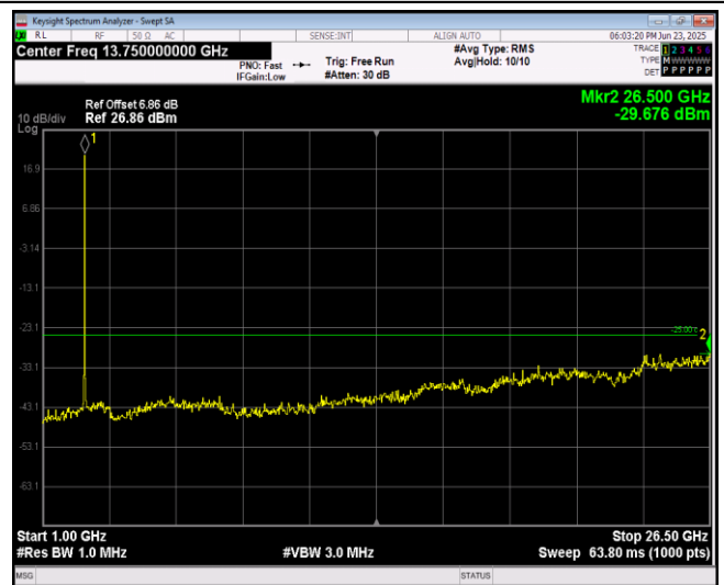
Band38-20MHz-16QAM-37850-1RB#0-Range2:1000~26500MHz
