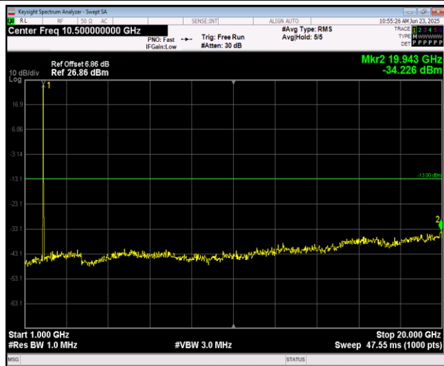
Band2-20MHz-64QAM-18900-1RB#0-Range2:1000~20000MHz
