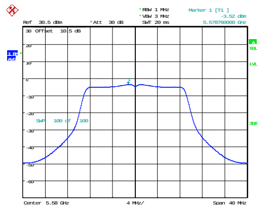
802.11n20_5580MHz_Chain 0
