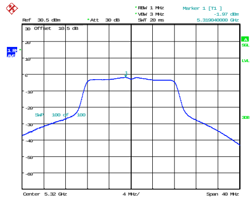
802.11a_5320MHz_Chain 1
