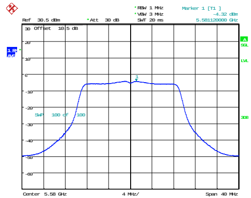
802.11n20_5580MHz_Chain 1
