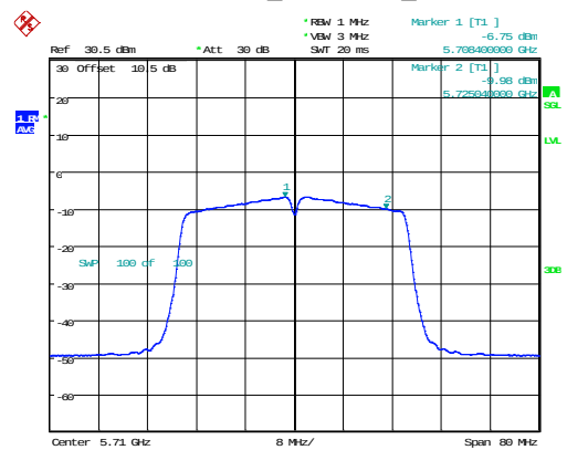
802.11n40_5710MHz_Chain 1
