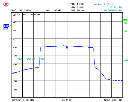
802.11ac80_5290MHz_Chain 1
