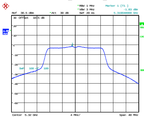
802.11n20_5320MHz_Chain 0
