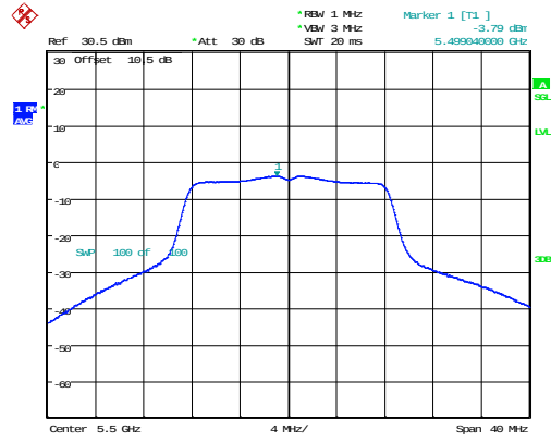
802.11a_5500MHz_Chain 1
