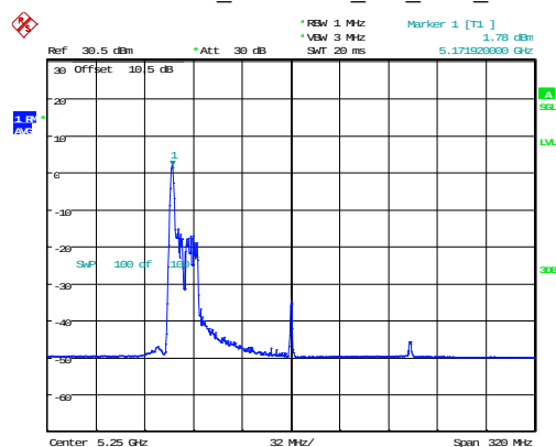
802.11ax160 5250MHz RU 26/0 Chain 1
