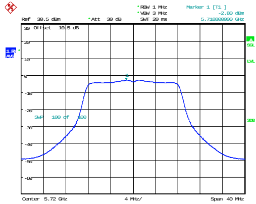
802.11a_5720MHz_Chain 0
