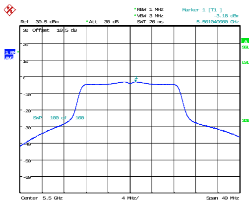
802.11n20_5500MHz_Chain 0
