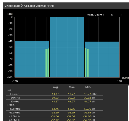
80MHz_30kHz_3660MHz-OFDM QPSK_RB216@0
