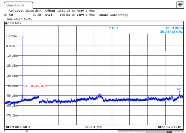
n78_2_50MHz_30kHz_3575MHz_DFT-s-OFDM QPSK_RB1@132 -46.94dBm
