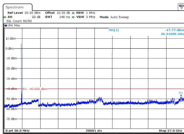
n78_2_90MHz_30kHz_3595MHz_DFT-s-OFDM QPSK_RB1@0 -47.77dBm
