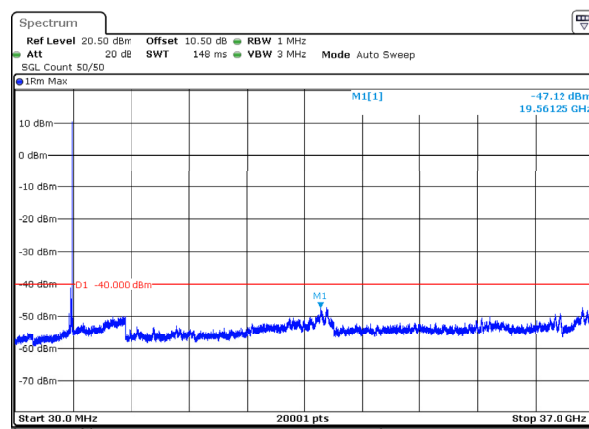
n78_2_90MHz_30kHz_3595MHz_DFT-s-OFDM QPSK_RB1@244 -47.12dBm
