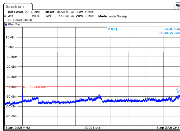
n78_2_60MHz_30kHz_3670MHz_DFT-s-OFDM QPSK_RB1@0 -46.46dBm
