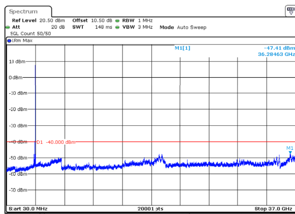
n78_2_90MHz_30kHz_3625MHz_DFT-s-OFDM QPSK_RB1@244 -47.41dBm
