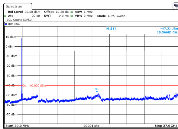
n78_2_90MHz_30kHz_3625MHz_DFT-s-OFDM QPSK_RB1@0 -47.23dBm
