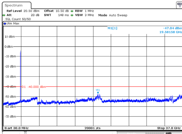
n78_2_50MHz_30kHz_3575MHz_DFT-s-OFDM QPSK_RB128@0 -47.04dBm
