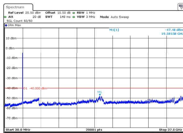
n78_2_60MHz_30kHz_3670MHz_DFT-s-OFDM QPSK_RB162@0 -47.48dBm
