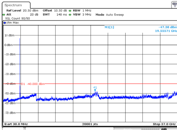
n78_2_50MHz_30kHz_3575MHz_DFT-s-OFDM QPSK_RB1@0 -47.38dBm
