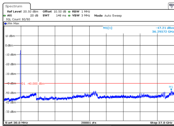
n78_2_90MHz_30kHz_3595MHz_DFT-s-OFDM QPSK_RB243@0 -47.21dBm
