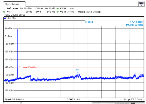
n78_2_50MHz_30kHz_3625MHz_DFT-s-OFDM QPSK_RB1@0 -47.48dBm
