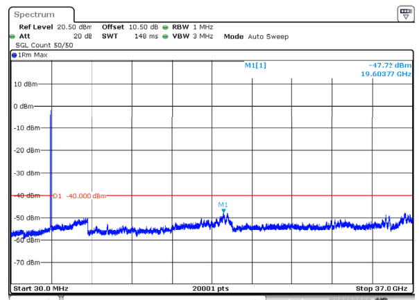
n78_2_50MHz_30kHz_3625MHz_DFT-s-OFDM QPSK_RB128@0 -47.72dBm
