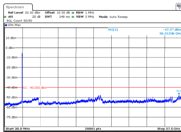
n78_2_90MHz_30kHz_3625MHz_DFT-s-OFDM QPSK_RB243@0 -47.27dBm
