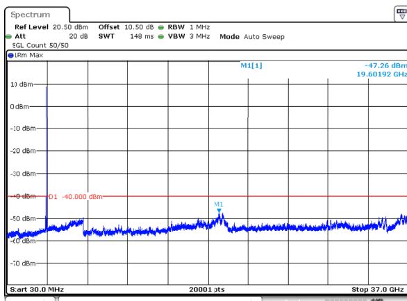
n78_2_50MHz_30kHz_3625MHz_DFT-s-OFDM QPSK_RB1@132 -47.26dBm
