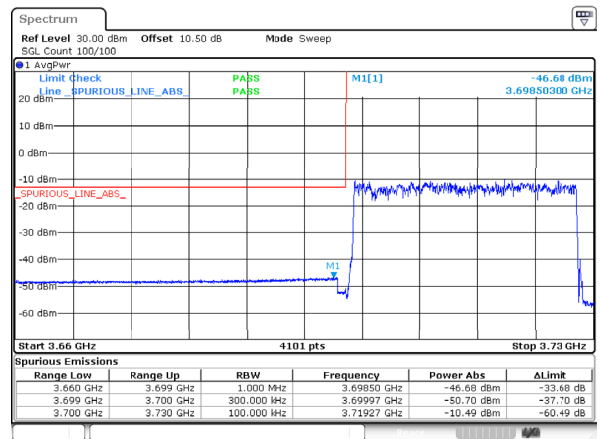
n78_3_30MHz_30kHz_3715MHz_DFT-s-OFDM QPSK_RB75@0
