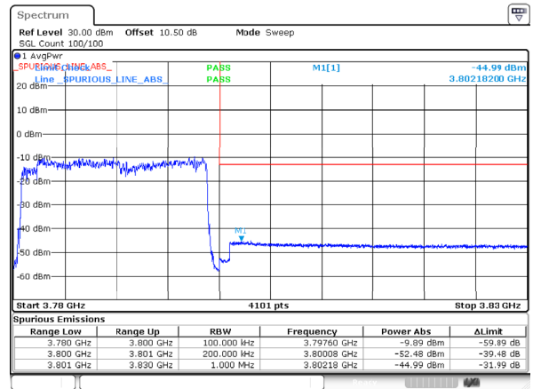
n78_3_20MHz_30kHz_3790MHz_DFT-s-OFDM QPSK_RB50@0
