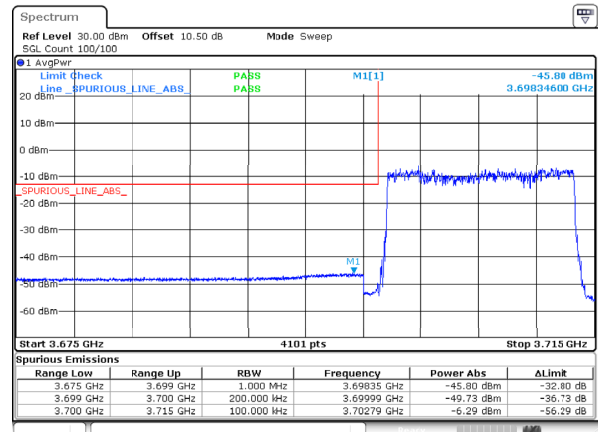
n78_3_15MHz_30kHz_3707.5MHz_DFT-s-OFDM QPSK_RB36@0
