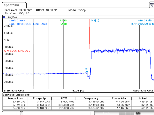
n78_1_30MHz_30kHz_3465MHz_DFT-s-OFDM QPSK_RB75@0
