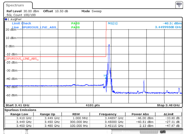
n78_1_30MHz_30kHz_3465MHz_DFT-s-OFDM QPSK_RB1@0
