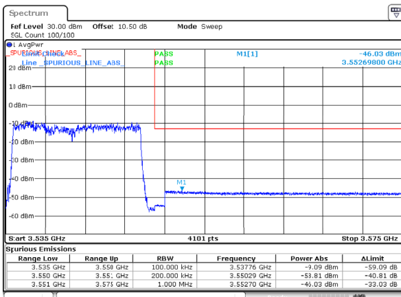
n78_1_15MHz_30kHz_3542.5MHz_DFT-s-OFDM QPSK_RB36@0
