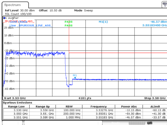
n78_1_20MHz_30kHz_3540MHz_DFT-s-OFDM QPSK_RB50@0
