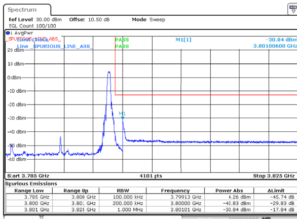
n78_3_15MHz_30kHz_3792.5MHz_DFT-s-OFDM QPSK_RB1@37
