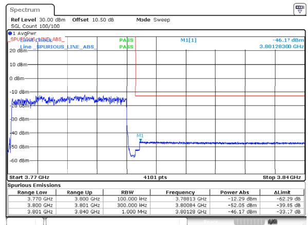
n78_3_30MHz_30kHz_3785MHz_DFT-s-OFDM QPSK_RB75@0
