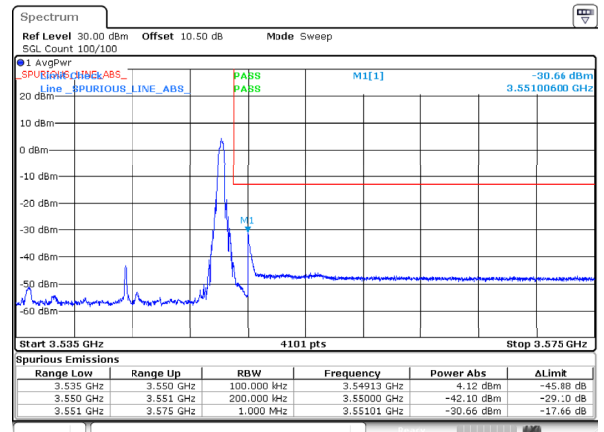
n78_1_15MHz_30kHz_3542.5MHz_DFT-s-OFDM QPSK_RB1@37
