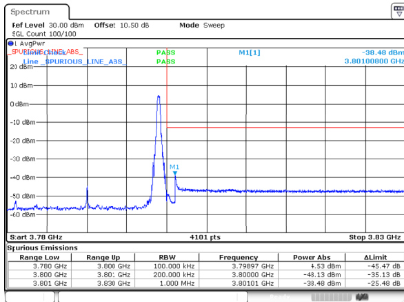
n78_3_20MHz_30kHz_3790MHz_DFT-s-OFDM QPSK_RB1@50
