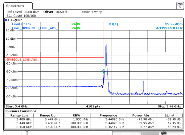
n78_1_40MHz_30kHz_3470MHz_DFT-s-OFDM QPSK_RB1@0
