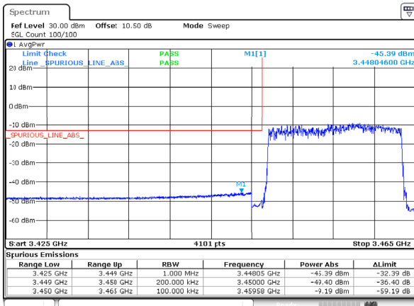
n78_1_15MHz_30kHz_3457.5MHz_DFT-s-OFDM QPSK_RB36@0
