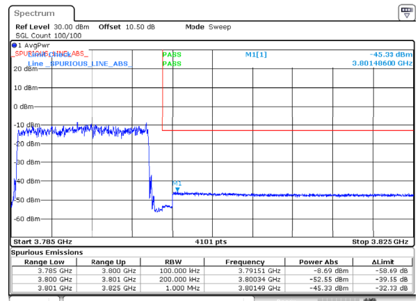
n78_3_15MHz_30kHz_3792.5MHz_DFT-s-OFDM QPSK_RB36@0
