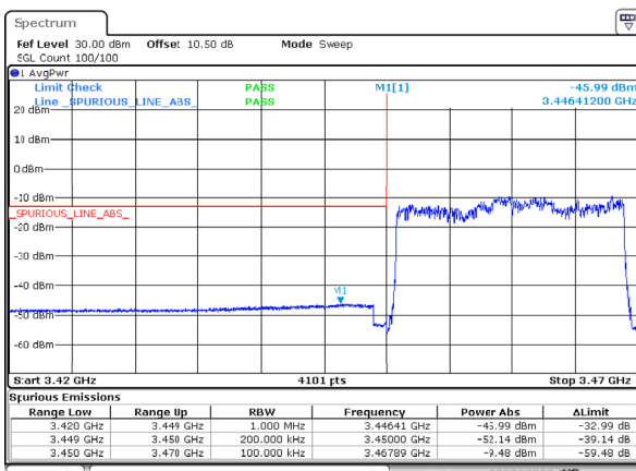
n78_1_20MHz_30kHz_3460MHz_DFT-s-OFDM QPSK_RB50@0
