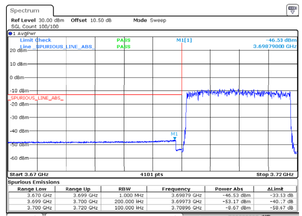
n78_3_20MHz_30kHz_3710MHz_DFT-s-OFDM QPSK_RB50@0
