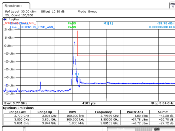
n78_3_30MHz_30kHz_3785MHz_DFT-s-OFDM QPSK_RB1@77
