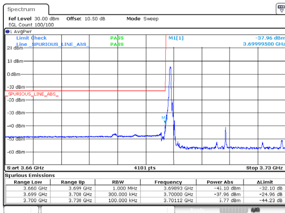
n78_3_30MHz_30kHz_3715MHz_DFT-s-OFDM QPSK_RB1@0
