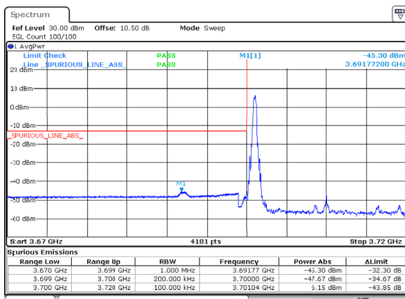
n78_3_20MHz_30kHz_3710MHz_DFT-s-OFDM QPSK_RB1@0
