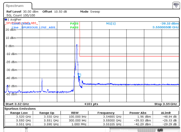
n78_1_30MHz_30kHz_3535MHz_DFT-s-OFDM QPSK_RB1@77
