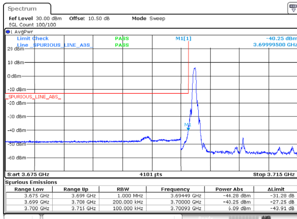
n78_3_15MHz_30kHz_3707.5MHz_DFT-s-OFDM QPSK_RB1@0
