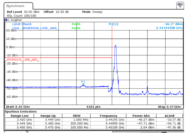
n78_1_20MHz_30kHz_3460MHz_DFT-s-OFDM QPSK_RB1@0
