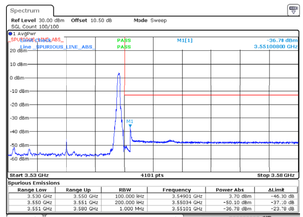
n78_1_20MHz_30kHz_3540MHz_DFT-s-OFDM QPSK_RB1@50
