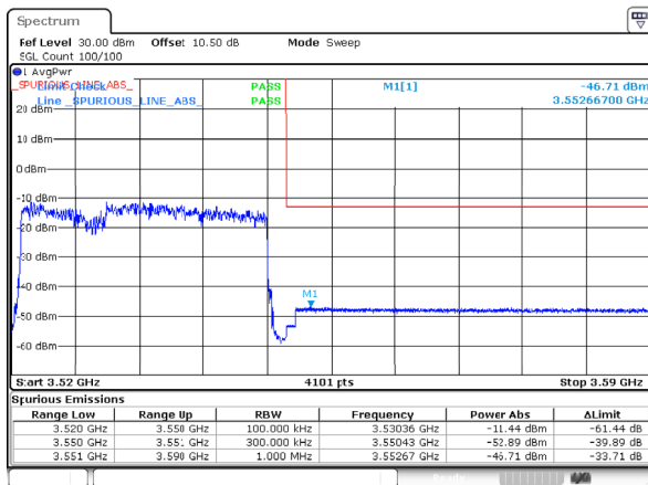
n78_1_30MHz_30kHz_3535MHz_DFT-s-OFDM QPSK_RB75@0
