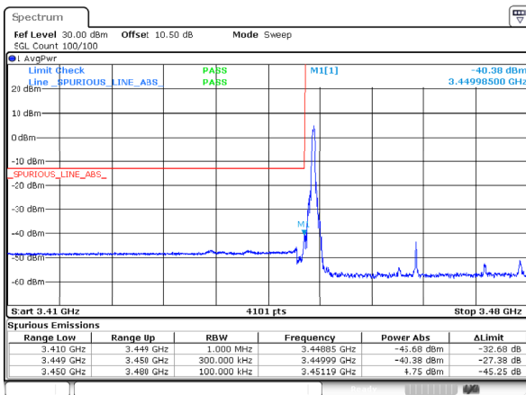
n77_1_30MHz_30kHz_3465MHz_DFT-s-OFDM QPSK_RB1@0
