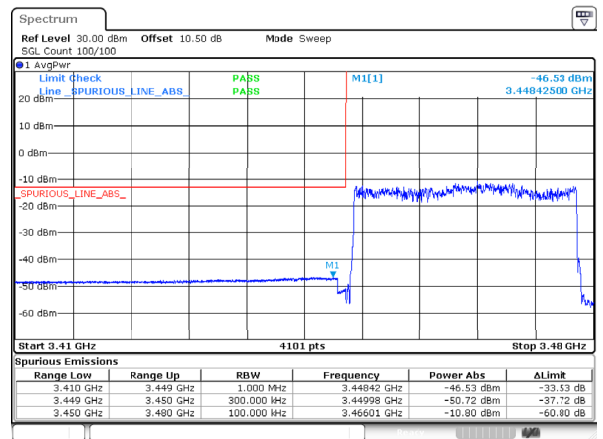
n77_1_30MHz_30kHz_3465MHz_DFT-s-OFDM QPSK_RB75@0
