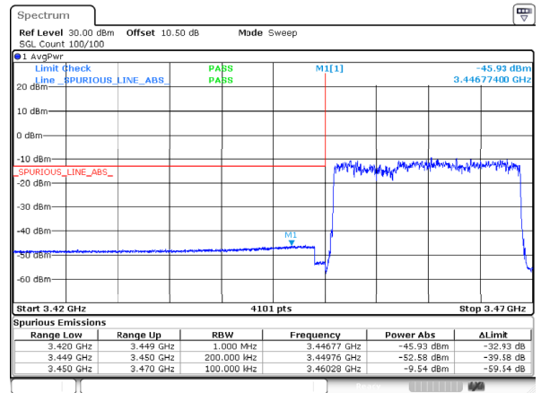
n77_1_20MHz_30kHz_3460MHz_DFT-s-OFDM QPSK_RB50@0
