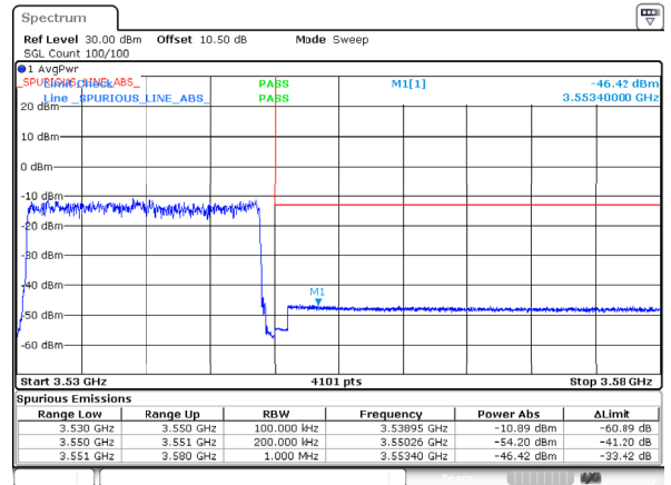
n77_1_20MHz_30kHz_3540MHz_DFT-s-OFDM QPSK_RB50@0
