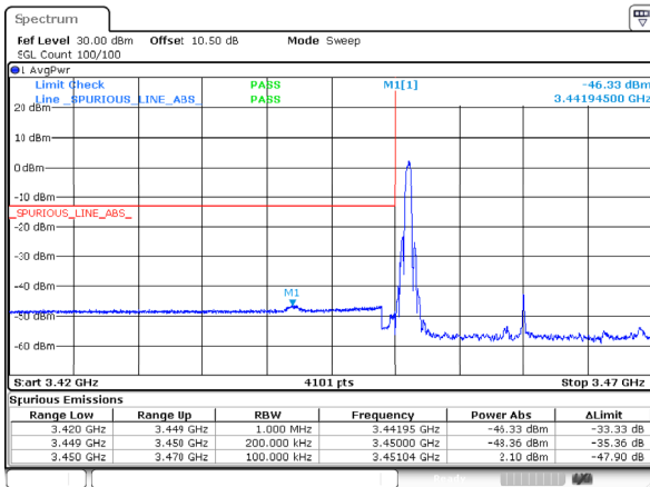
n77_1_20MHz_30kHz_3460MHz_DFT-s-OFDM QPSK_RB1@0
