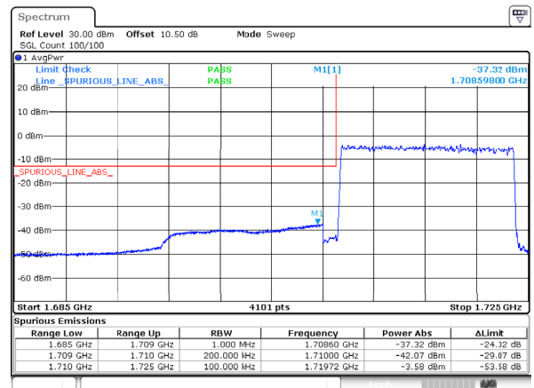
n66_15MHz_15kHz_1717.5MHz_DFT-s-OFDM QPSK_RB75@0
