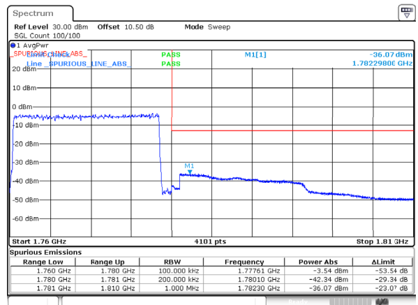
n66_20MHz_15kHz_1770MHz_DFT-s-OFDM QPSK_RB100@0
