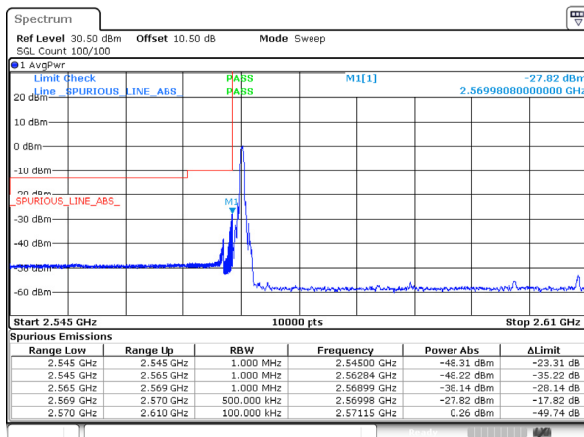
n38_40MHz_30kHz_2590MHz_DFT-s-OFDM QPSK_RB1@0
