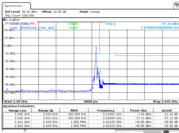
n38_30MHz_30kHz_2605MHz_DFT-s-OFDM QPSK_RB1@77
