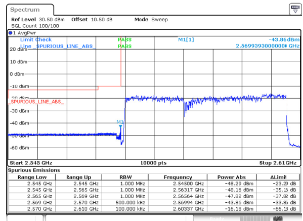
n38_40MHz_30kHz_2590MHz_DFT-s-OFDM QPSK_RB100@0
