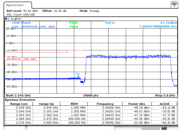
n38_30MHz_30kHz_2585MHz_DFT-s-OFDM QPSK_RB75@0
