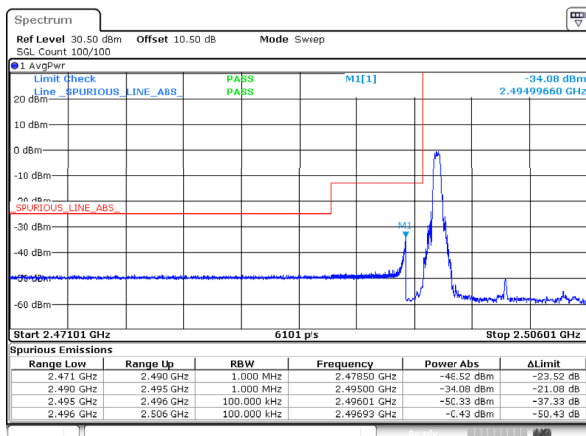
n41_10MHz_30kHz_2501.01MHz_DFT-s-OFDM QPSK_RB1@0
