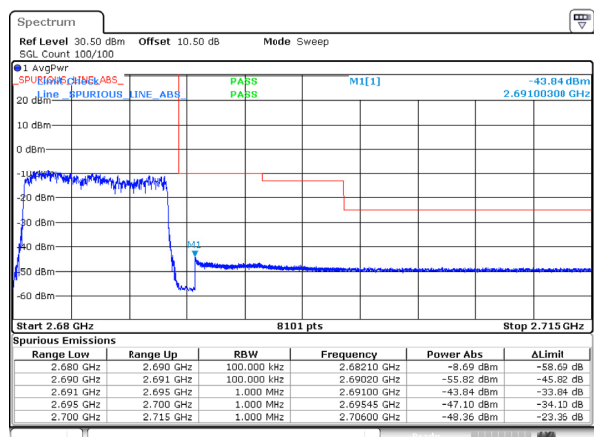
n41_10MHz_30kHz_2685MHz_DFT-s-OFDM QPSK_RB24@0
