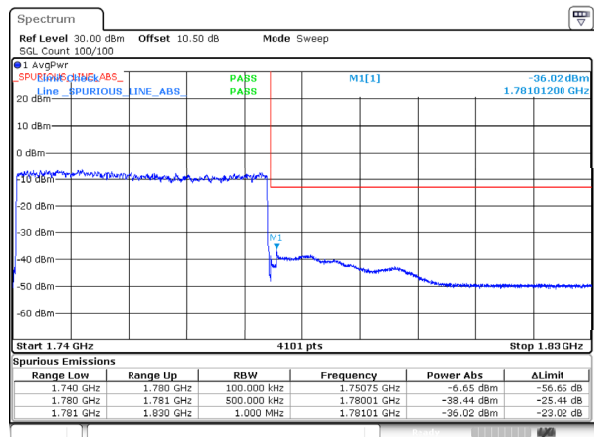
n66_40MHz_15kHz_1760MHz_DFT-s-OFDM QPSK_RB216@0
