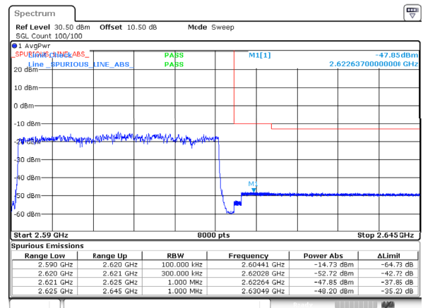
n38_30MHz_30kHz_2605MHz_DFT-s-OFDM QPSK_RB75@0
