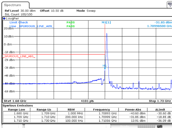
n66_20MHz_15kHz_1720MHz_DFT-s-OFDM QPSK_RB1@0
