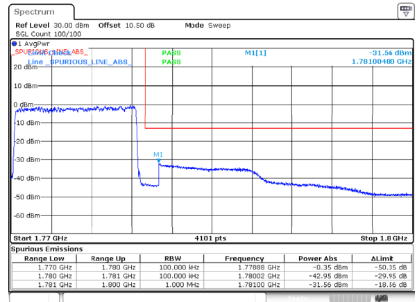
n66_10MHz_15kHz_1775MHz_DFT-s-OFDM QPSK_RB50@0
