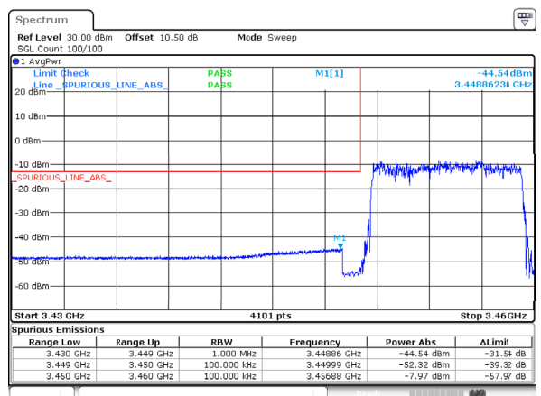
n77_1_10MHz_30kHz_3455MHz_DFT-s-OFDM QPSK_RB24@0
