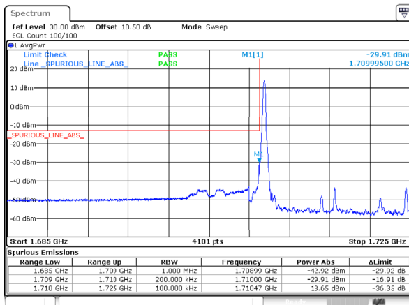
n66_15MHz_15kHz_1717.5MHz_DFT-s-OFDM QPSK_RB1@0
