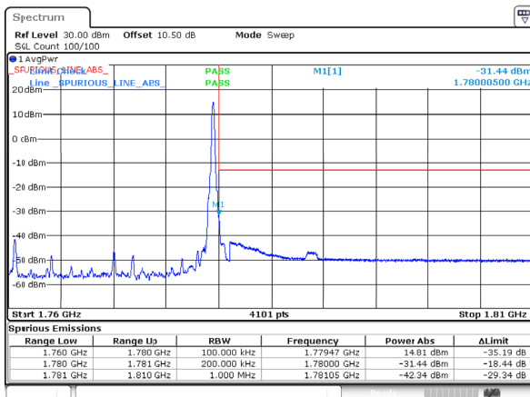
n66_20MHz_15kHz_1770MHz_DFT-s-OFDM QPSK_RB1@105
