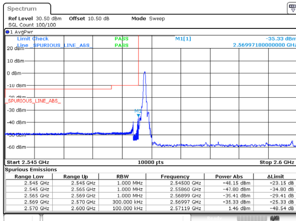
n38_30MHz_30kHz_2585MHz_DFT-s-OFDM QPSK_RB1@0
