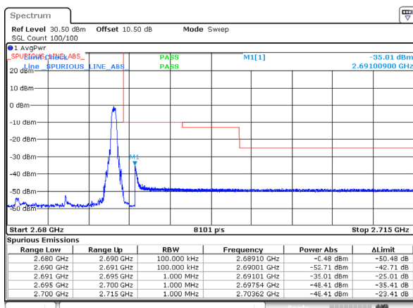
n41_10MHz_30kHz_2685MHz_DFT-s-OFDM QPSK_RB1@23
