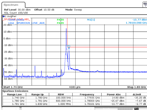
n66_40MHz_15kHz_1760MHz_DFT-s-OFDM QPSK_RB1@215
