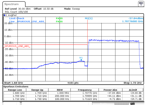
n66_20MHz_15kHz_1720MHz_DFT-s-OFDM QPSK_RB100@0
