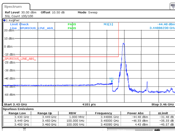
n77_1_10MHz_30kHz_3455MHz_DFT-s-OFDM QPSK_RB1@0
