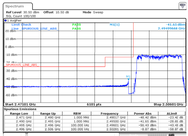
n41_10MHz_30kHz_2501.01MHz_DFT-s-OFDM QPSK_RB24@0
