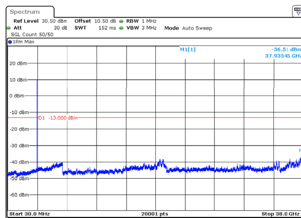
n78_3_40MHz_30kHz_3750MHz_DFT-s-OFDM QPSK_RB1@0 -36.51dBm
