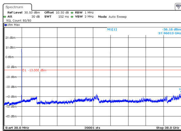
n78_3_40MHz_30kHz_3750MHz_DFT-s-OFDM QPSK_RB1@105 -36.16dBm
