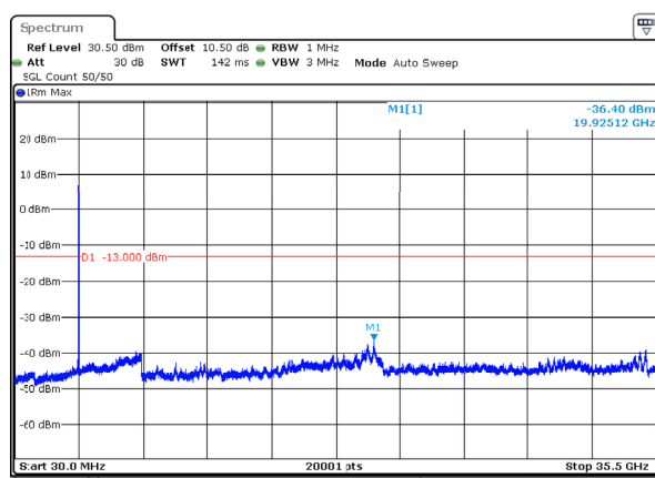
n78_1_80MHz_30kHz_3510MHz_DFT-s-OFDM QPSK_RB1@216 -36.40dBm
