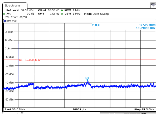
n78_1_90MHz_30kHz_3495MHz_DFT-s-OFDM QPSK_RB1@0 -37.98dBm
