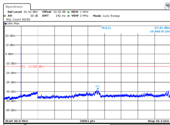
n78_1_80MHz_30kHz_3500MHz_DFT-s-OFDM QPSK_RB1@216 -37.84dBm
