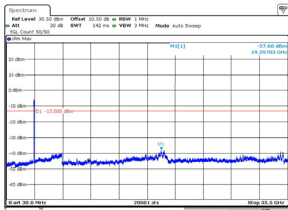
n78_1_90MHz_30kHz_3495MHz_DFT-s-OFDM QPSK_RB243@0 -37.60dBm
