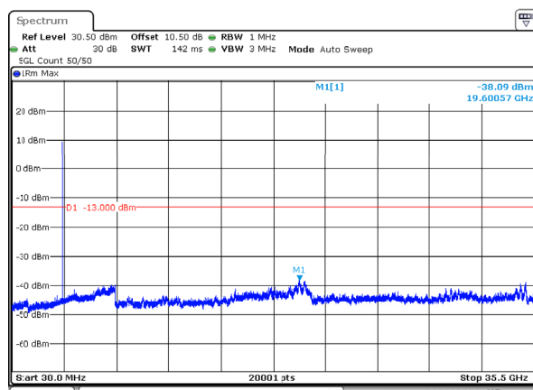
n78_1_80MHz_30kHz_3500MHz_DFT-s-OFDM QPSK_RB1@0 -38.09dBm
