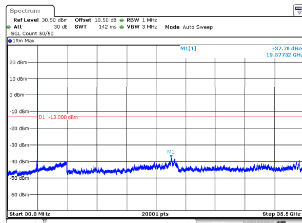
n78_1_90MHz_30kHz_3495MHz_DFT-s-OFDM QPSK_RB1@244 -37.70dBm
