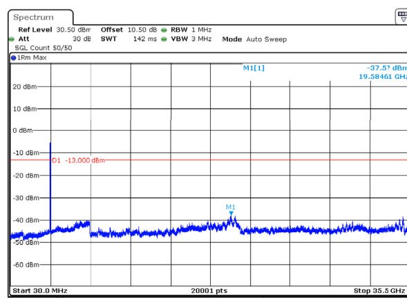
n78_1_80MHz_30kHz_3510MHz_DFT-s-OFDM QPSK_RB216@0 -37.57dBm
