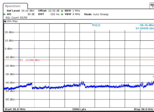
n78_3_40MHz_30kHz_3720MHz_DFT-s-OFDM QPSK_RB1@105 -36.46dBm
