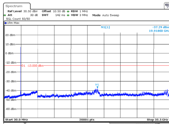
n78_1_90MHz_30kHz_3500MHz_DFT-s-OFDM QPSK_RB1@0 -37.29dBm
