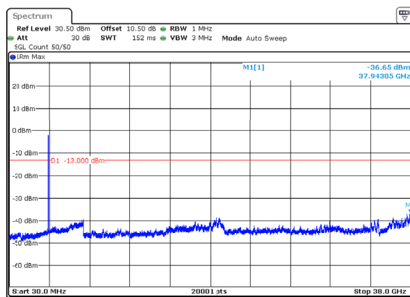
n78_3_40MHz_30kHz_3720MHz_DFT-s-OFDM QPSK_RB100@0 -36.65dBm
