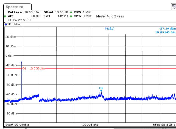
n78_1_90MHz_30kHz_3500MHz_DFT-s-OFDM QPSK_RB243@0 -37.29dBm
