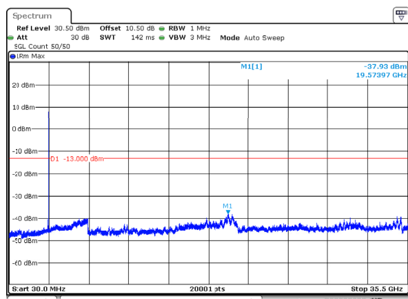
n78_1_90MHz_30kHz_3500MHz_DFT-s-OFDM QPSK_RB1@244 -37.93dBm
