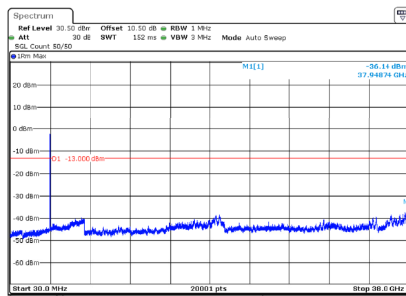
n78_3_40MHz_30kHz_3750MHz_DFT-s-OFDM QPSK_RB100@0 -36.14dBm
