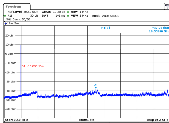
n78_1_80MHz_30kHz_3510MHz_DFT-s-OFDM QPSK_RB1@0 -37.70dBm
