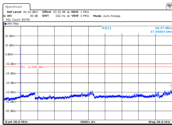
n78_3_40MHz_30kHz_3720MHz_DFT-s-OFDM QPSK_RB1@0 -36.57dBm
