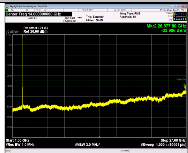
41-41-20MHz-10MHz-QPSK-QPSK-39750-39894-1RB#99- ORB#0-1000~27000MHz-PASS
