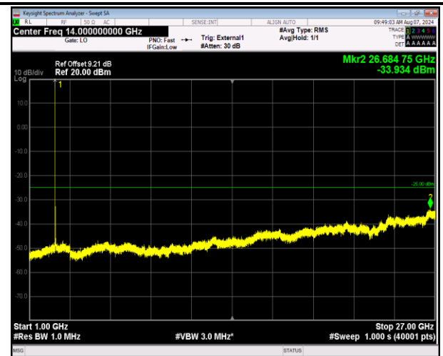
41-41-20MHz-10MHz-QPSK-QPSK-41391-41535-1RB#0-0 RB#0-1000~27000MHz-PASS
