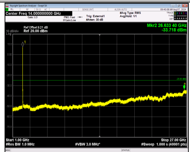
41-41-20MHz-10MHz-QPSK-QPSK-39750-39894-100RB#0 -50RB#0-1000~27000MHz-PASS
