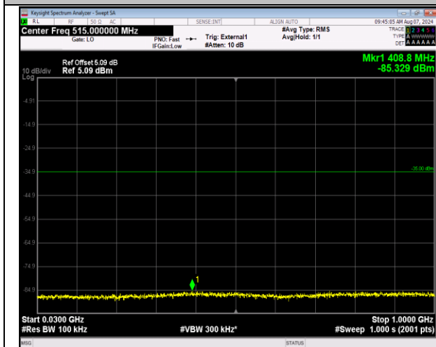
41-41-20MHz-10MHz-QPSK-QPSK-40571-40715-1RB#0 -1RB#49-30~1000MHz-PASS
