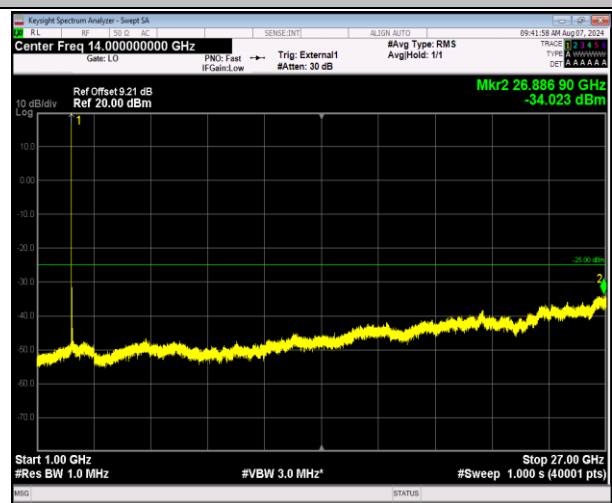
41-41-20MHz-10MHz-QPSK-QPSK-40571-40715-1RB#0-0 RB#0-1000~27000MHz-PASS
