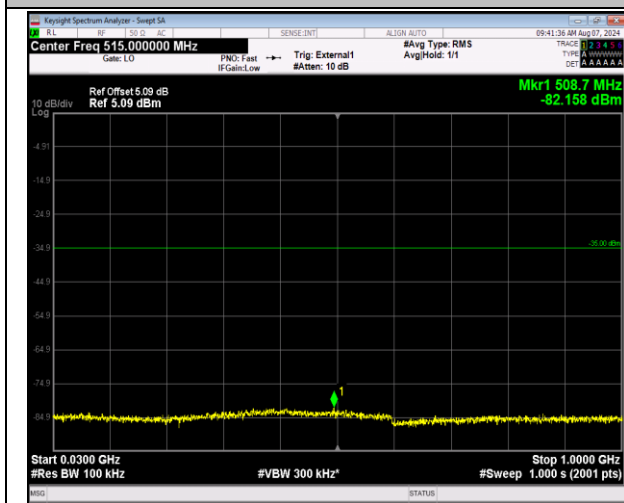
41-41-20MHz-10MHz-QPSK-QPSK-40571-40715-1RB#0 -ORB#0-30~1000MHz-PASS
