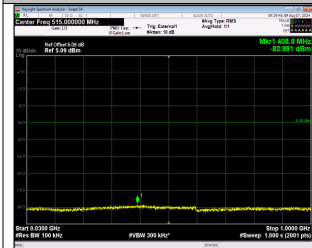
41-41-20MHz-10MHz-QPSK-QPSK-39750-39894-100RB #0-50RB#0-30~1000MHz-PASS
