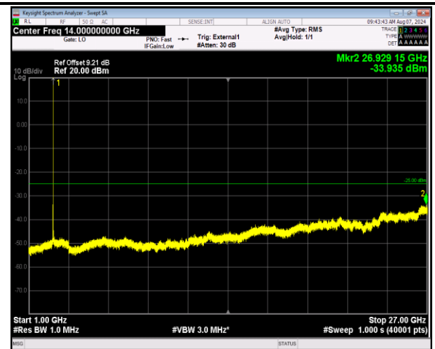
41-41-20MHz-10MHz-QPSK-QPSK-40571-40715-1RB#99- ORB#0-1000~27000MHz-PASS
