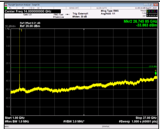
41-41-20MHz-20MHz-QPSK-QPSK-40521-40719-1RB#99- ORB#0-1000~27000MHz-PASS
