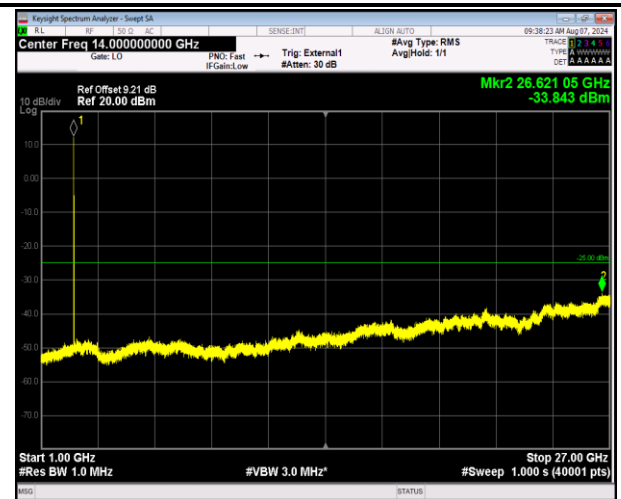
41-41-20MHz-10MHz-QPSK-QPSK-39750-39894-1RB#0-1 RB#49-1000~27000MHz-PASS
