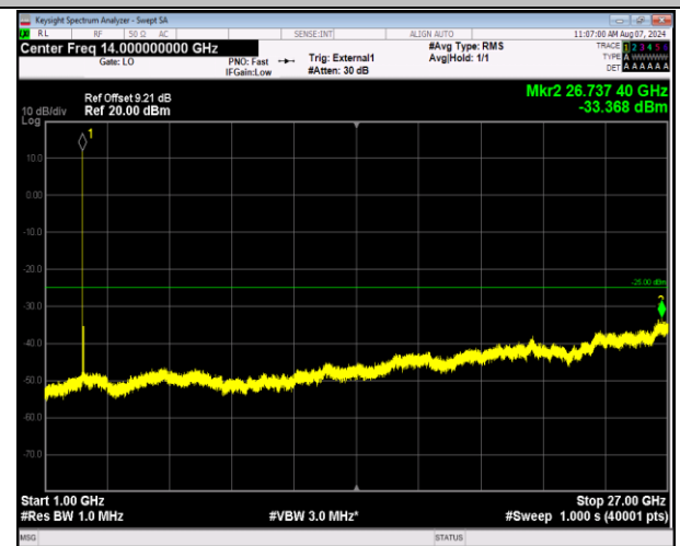
41-41-20MHz-20MHz-QPSK-QPSK-40521-40719-1RB#0-1 RB#99-1000~27000MHz-PASS
