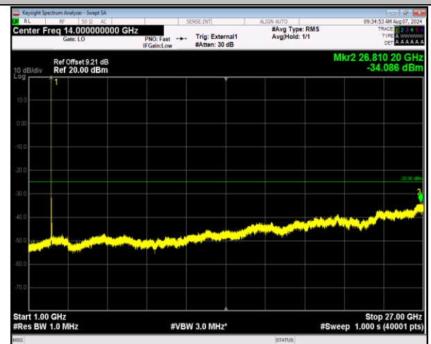
41-41-20MHz-10MHz-QPSK-QPSK-39750-39894-1RB#0-0 RB#0-1000~27000MHz-PASS
