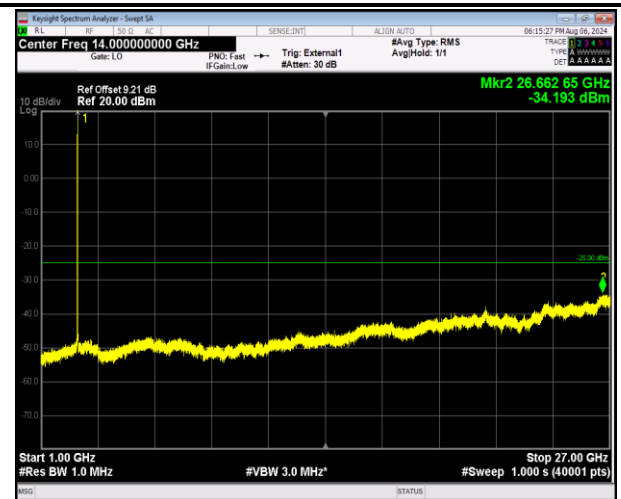
41-41-20MHz-5MHz-QPSK-QPSK-41440-41557-1RB#0-ORB#0-1000~27000MHz-PASS
