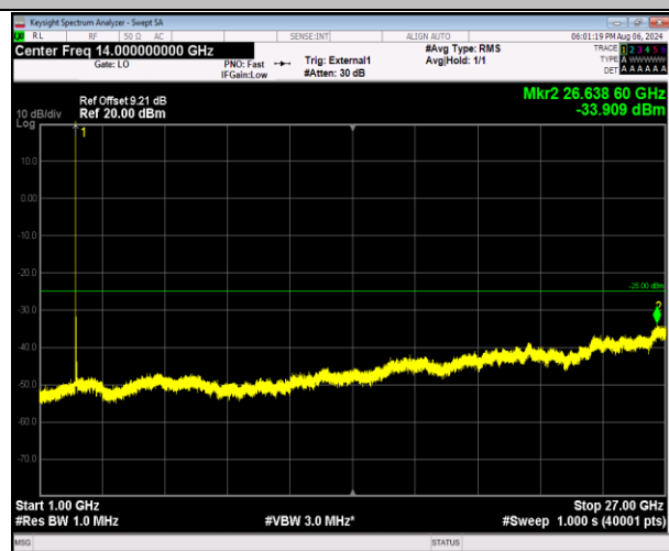
41-41-20MHz-5MHz-QPSK-QPSK-39750-39867-1RB#0-0R B#0-1000~27000MHz-PASS
