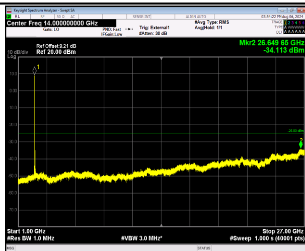
41-41-5MHz-20MHz-QPSK-QPSK-39683-39800-1RB#0-1RB#99-1000~27000MHz-PASS
