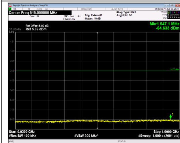
41-41-5MHz-20MHz-QPSK-QPSK-40528-40645-1RB#0- 1RB#99-30~1000MHz-PASS
