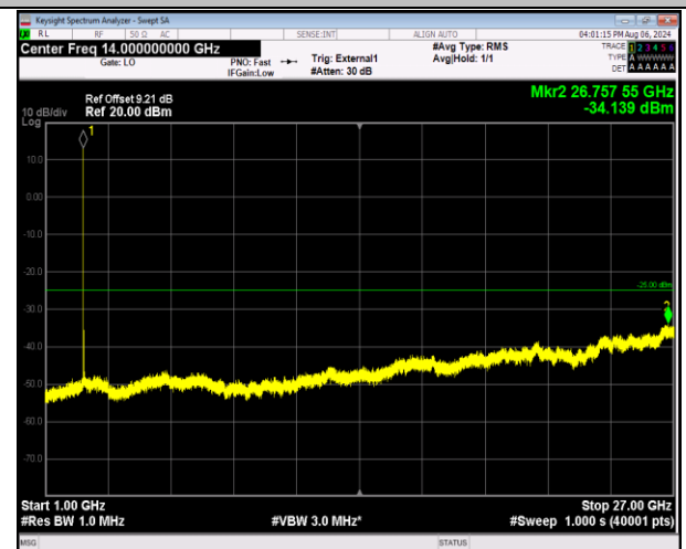
41-41-5MHz-20MHz-QPSK-QPSK-40528-40645-1RB#0-1R B#99-1000~27000MHz-PASS
