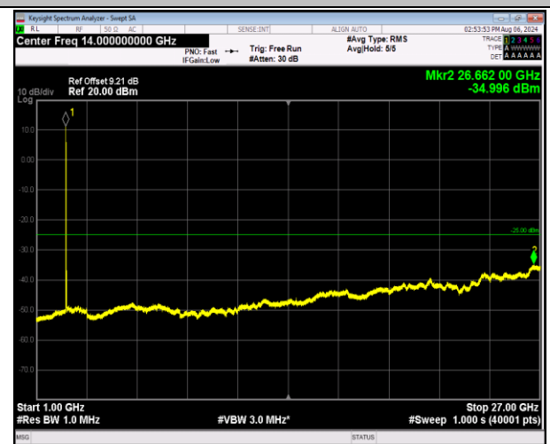
7-7-20MHz-20MHz-QPSK-QPSK-21152-21350-1RB#0-1RB #99-1000~27000MHz-PASS
