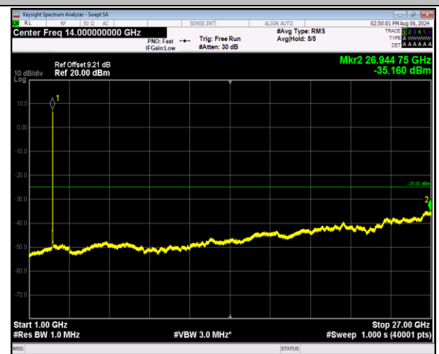
7-7-20MHz-20MHz-QPSK-QPSK-21001-21199-100RB#0-1 00RB#0-1000~27000MHz-PASS
