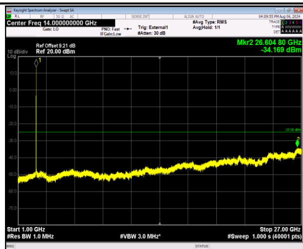
41-41-5MHz-20MHz-QPSK-QPSK-41373-41490-25RB#0-1 00RB#0-1000~27000MHz-PASS
