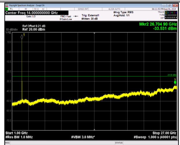
41-41-20MHz-5MHz-QPSK-QPSK-40595-40712-1RB#0-1RB#24-1000~27000MHz-PASS
