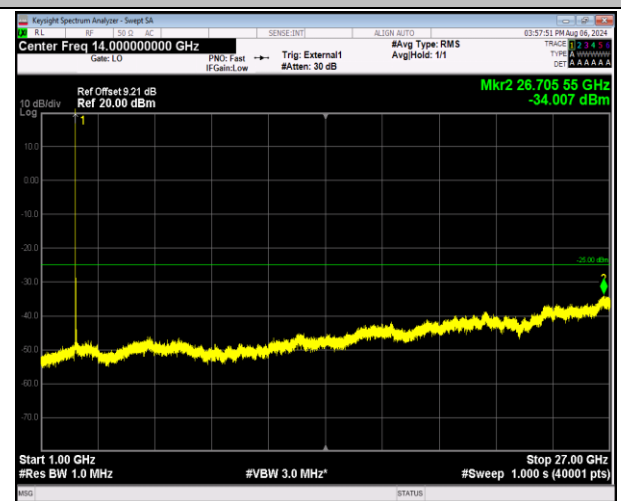
41-41-5MHz-20MHz-QPSK-QPSK-40528-40645-1RB#0-0RB#0-1000~27000MHz-PASS
