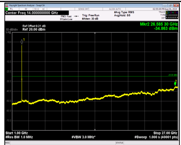
7-7-20MHz-20MHz-QPSK-QPSK-21152-21350-100RB#0-1 00RB#0-1000~27000MHz-PASS
