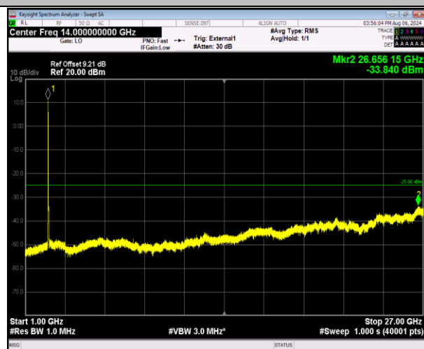
41-41-5MHz-20MHz-QPSK-QPSK-39683-39800-25RB#0-100RB#0-1000~27000MHz-PASS
