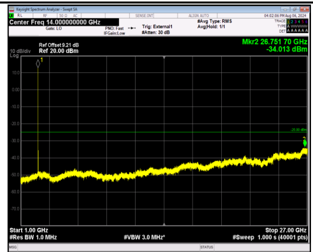
41-41-5MHz-20MHz-16QAM-16QAM-40528-40645-1RB#0- 1RB#99-1000~27000MHz-PASS
