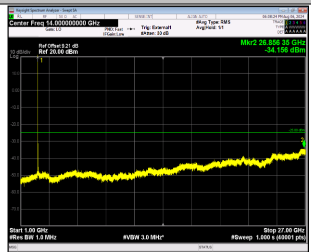
41-41-20MHz-5MHz-QPSK-QPSK-40595-40712-1RB#0-0RB#0-1000~27000MHz-PASS
