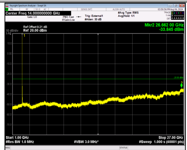
41-41-5MHz-20MHz-QPSK-QPSK-39683-39800-1RB#0-0R B#0-1000~27000MHz-PASS
