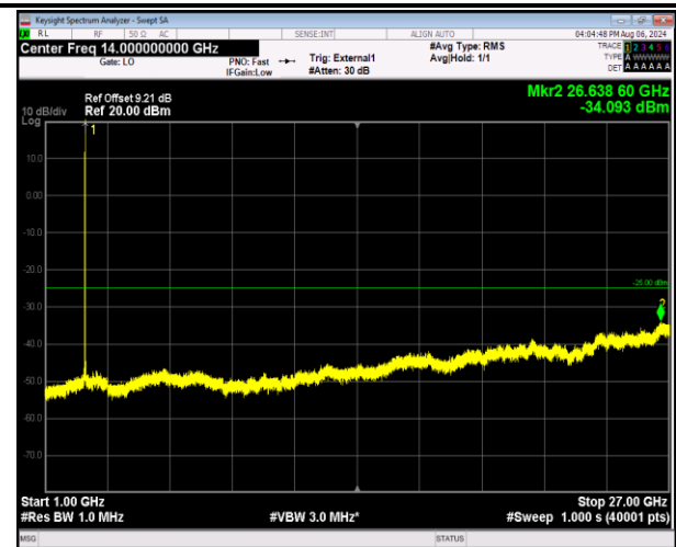
41-41-5MHz-20MHz-QPSK-QPSK-41373-41490-1RB#0-0R B#0-1000~27000MHz-PASS
