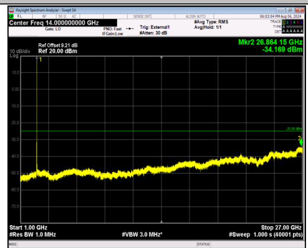
41-41-20MHz-5MHz-QPSK-QPSK-39750-39867-1RB#99-0 RB#0-1000~27000MHz-PASS
