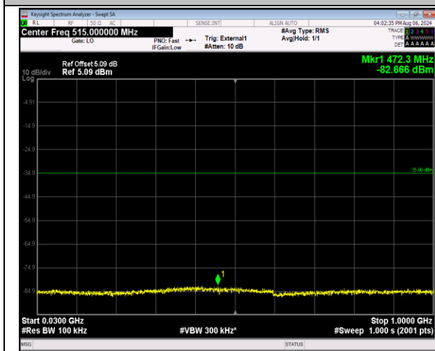
41-41-5MHz-20MHz-QPSK-QPSK-40528-40645-25RB#0 -100RB#0-30~1000MHz-PASS
