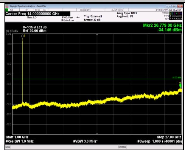
41-41-5MHz-20MHz-QPSK-QPSK-40528-40645-25RB#0-1 00RB#0-1000~27000MHz-PASS
