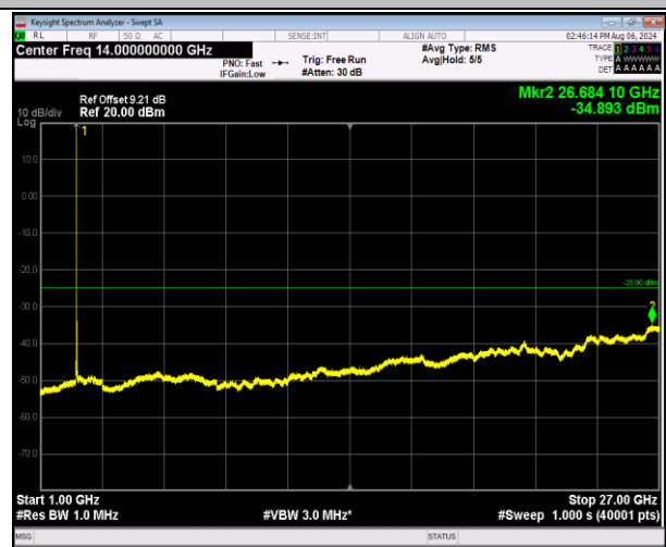
7-7-20MHz-20MHz-QPSK-QPSK-21001-21199-1RB#0-0RB #0-1000~27000MHz-PASS
