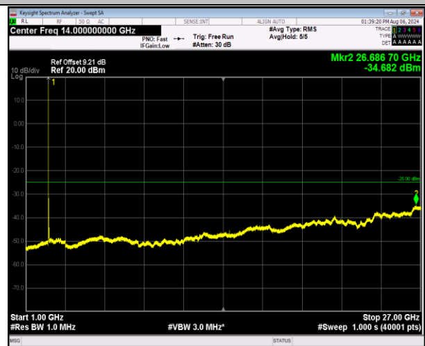
7-7-20MHz-10MHz-QPSK-QPSK-20850-20994-1RB#0-0-1000~27000MHz-PASS
