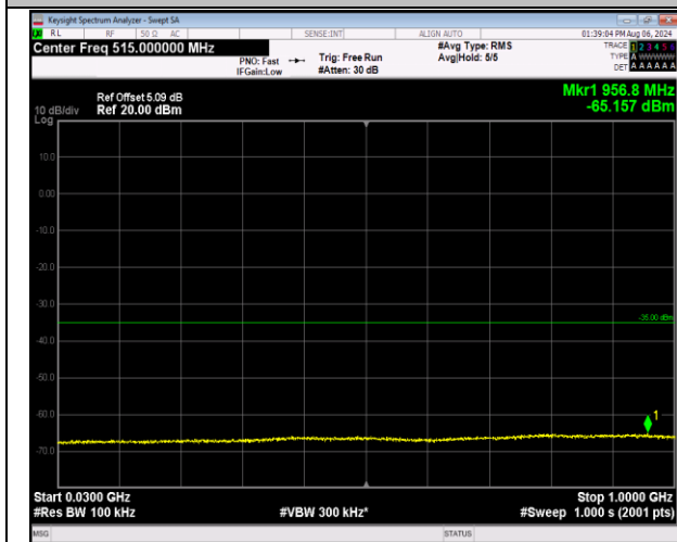
7-7-20MHz-10MHz-QPSK-QPSK-20850-20994-1RB#0-0-30~1000MHz-PASS
