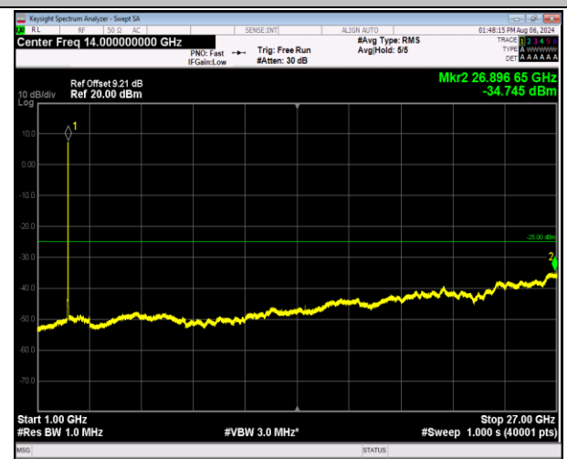
7-7-20MHz-10MHz-QPSK-QPSK-21051-21195-100RB#0-5 ORB#0-1000~27000MHz-PASS
